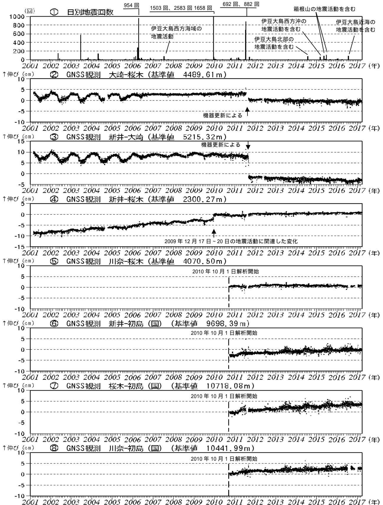
図3 伊豆東部火山群 火山活動経過図(2001年1月1日~2017年3月31日)
