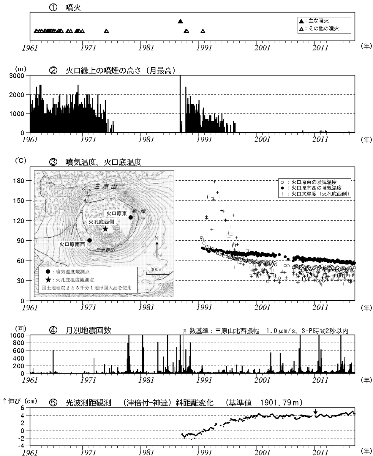
図1 伊豆大島 長期間の火山活動経過図 (1961年1月~2016年11月30日)
