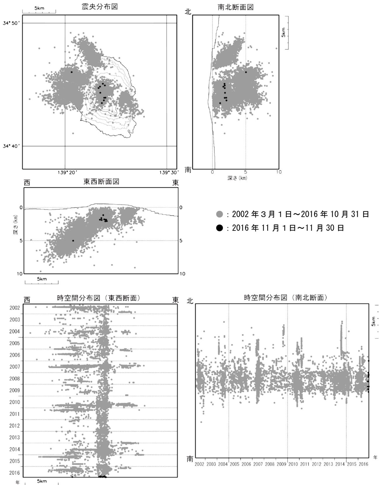
図 4 伊豆大島 震源分布図 (2002 年 3 月 1 日 ~ 2016 年 11 月 30 日)
