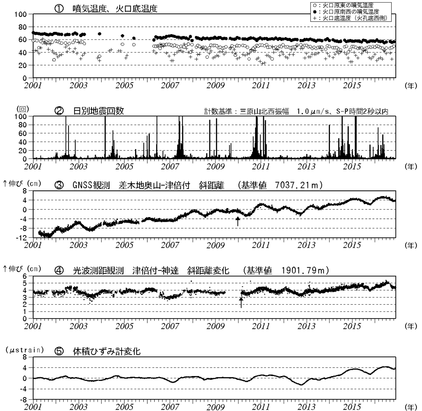
図2 伊豆大島 最近の火山活動経過図 (2001年1月～2016年11月30日)
