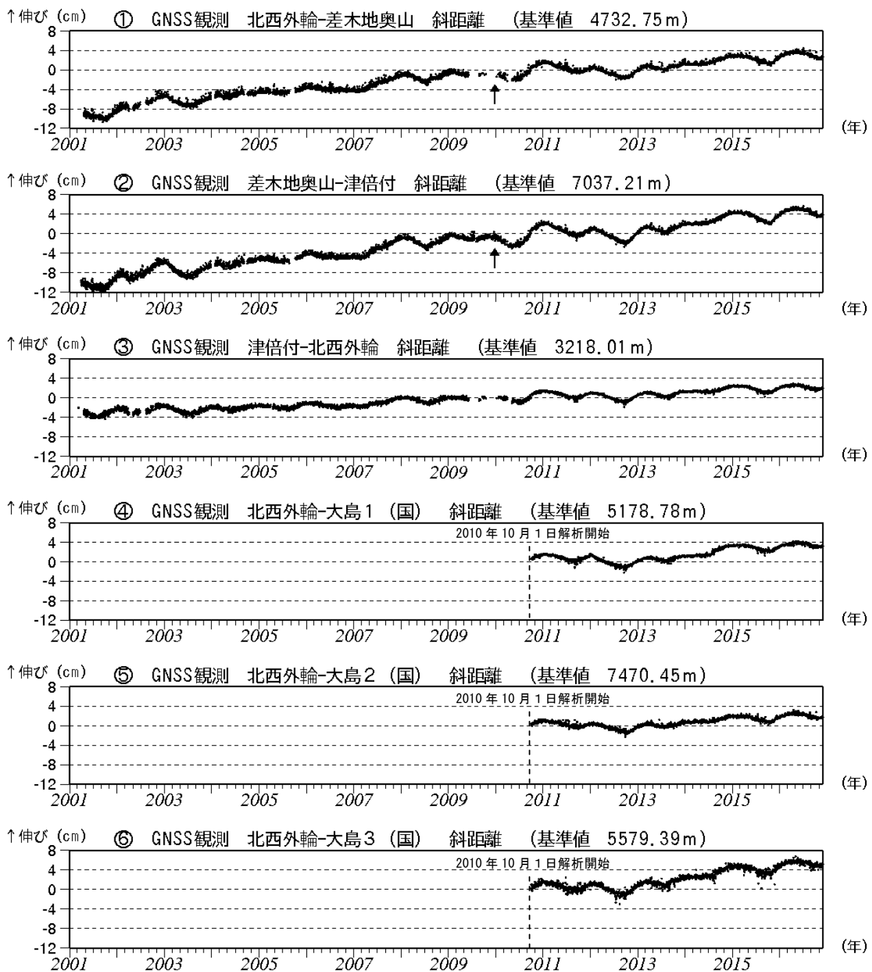
図3 伊豆大島 GNSS 連続観測による基線長変化(2001年1月~2016年11月30日)(国): 国土地理院 2010年10月以降のデータについては、電離層の影響を補正する等、解析方法を改良しています。
