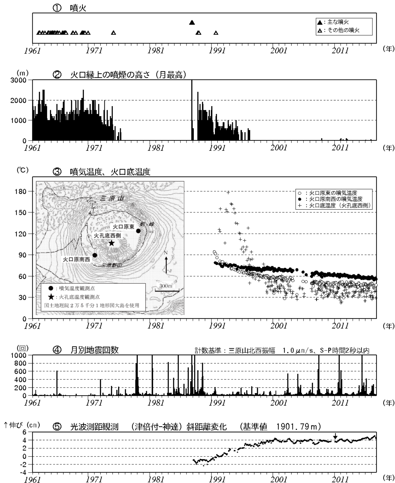
図 1 伊豆大島 長期間の火山活動経過図（1961 年 1 月～2016 年 10 月 31 日）
