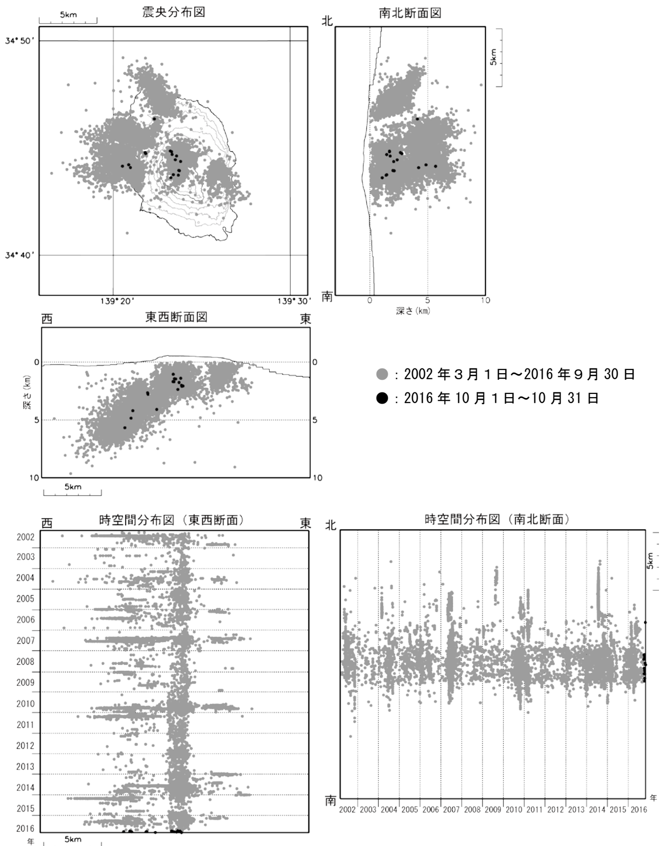
図 4 伊豆大島 震源分布図（2002 年 3 月 1 日～2016 年 10 月 31 日）
