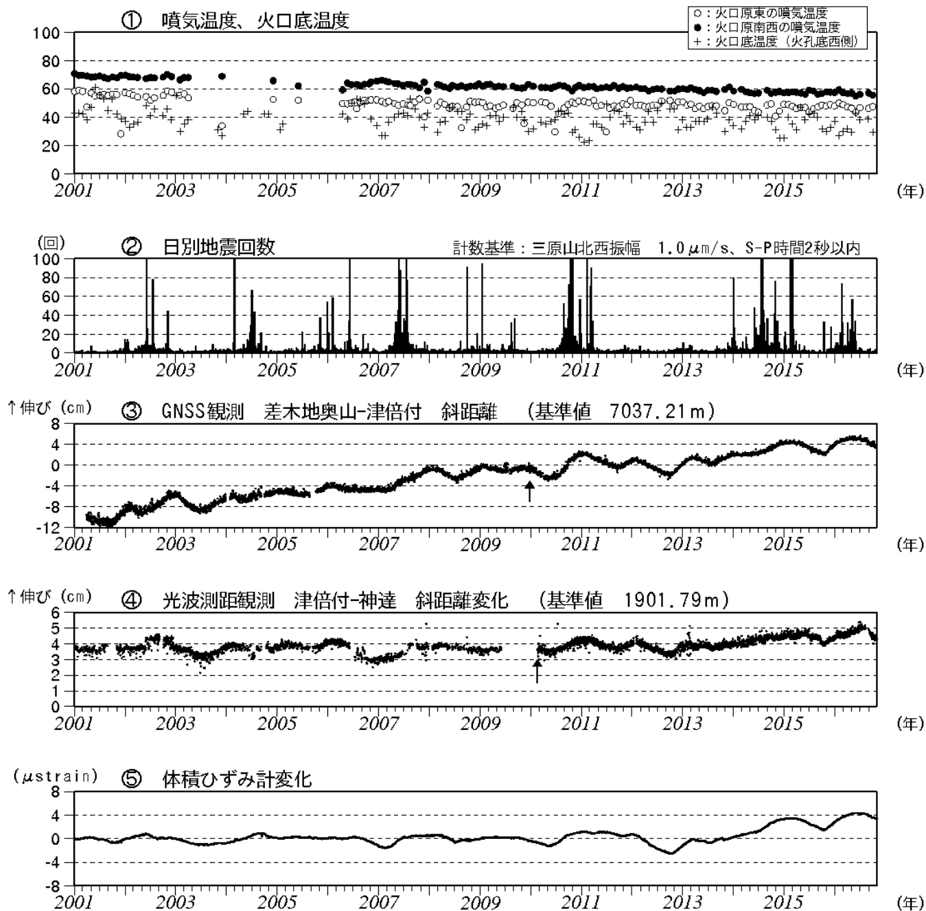
図2 伊豆大島 最近の火山活動経過図（2001年1月～2016年10月31日）
