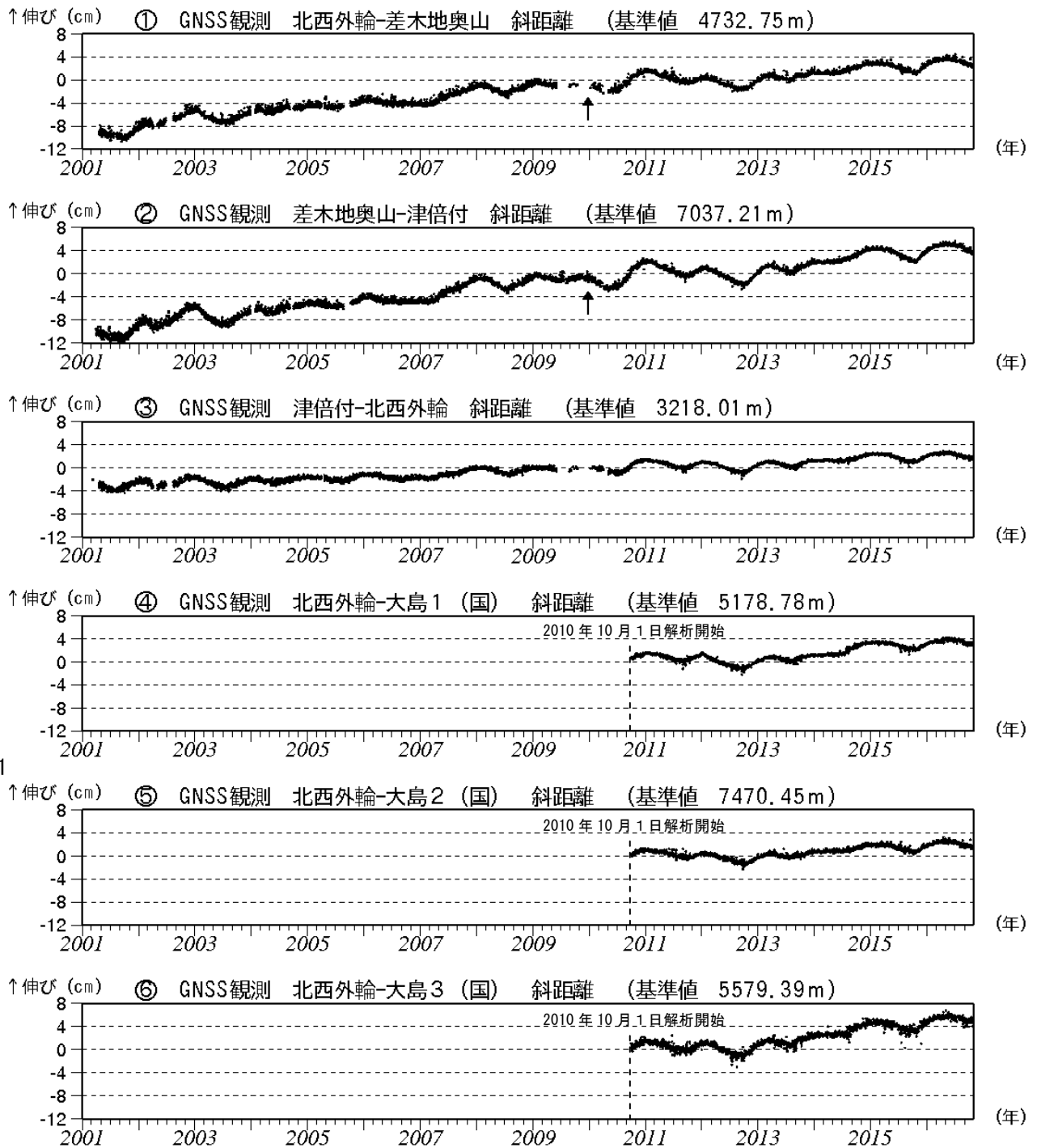
図3 伊豆大島 GNSS 連続観測による基線長変化(2001 年 1 月～2016 年 10 月 31 日)(国)：国土地理院 2010 年 10 月以降のデータについては、電離層の影響を補正する等、解析方法を改良しています。
