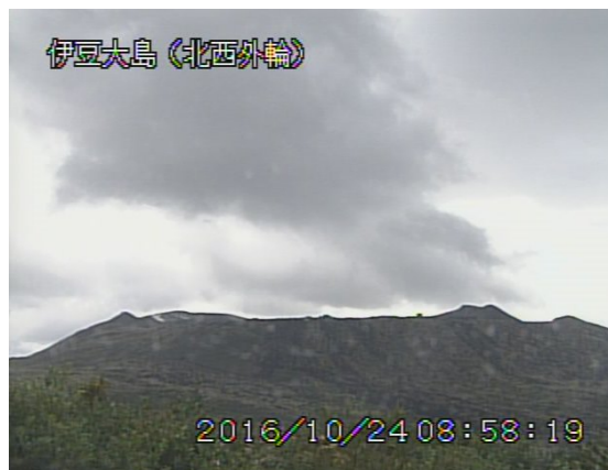
図 5 伊豆大島 三原山山頂部の状況（10 月 24 日、北西外輪遠望カメラによる）
