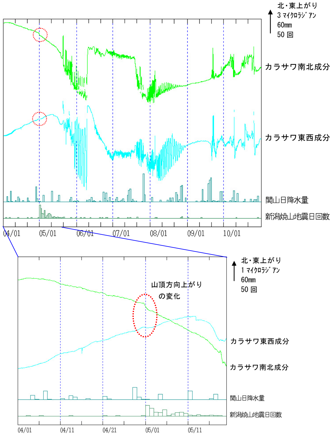
図9 新潟焼山 カラサワ観測点（山頂の北約4km）の傾斜変動（2016年4月1日～10月31日）
