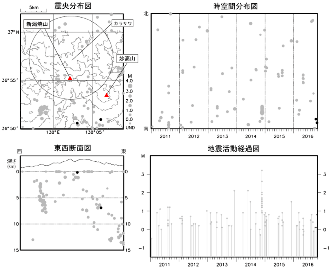
図 8 新潟焼山 広域地震観測網による山体周辺の地震活動（2011 年 1 月 1 日～2016 年 10 月 31 日）
