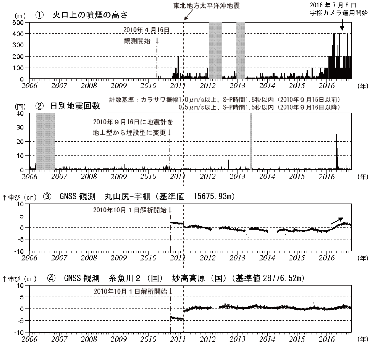
図3 新潟焼山 火山活動経過図（2006年1月1日～2016年10月31日）
