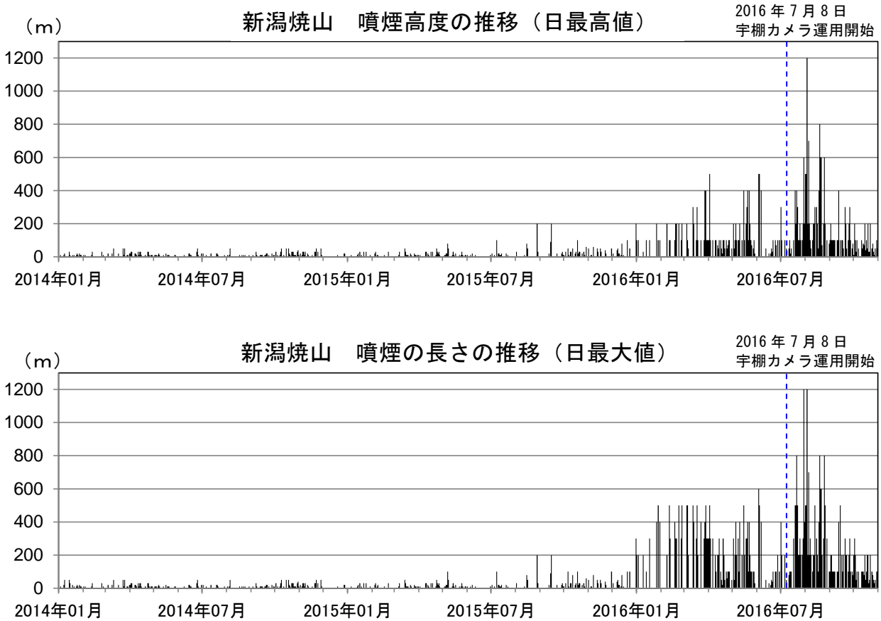
図4 新潟焼山 噴煙高度と噴煙の長さの推移 （それぞれ日最高値及び日最大値、2014年1月1日～2016年10月31日）
