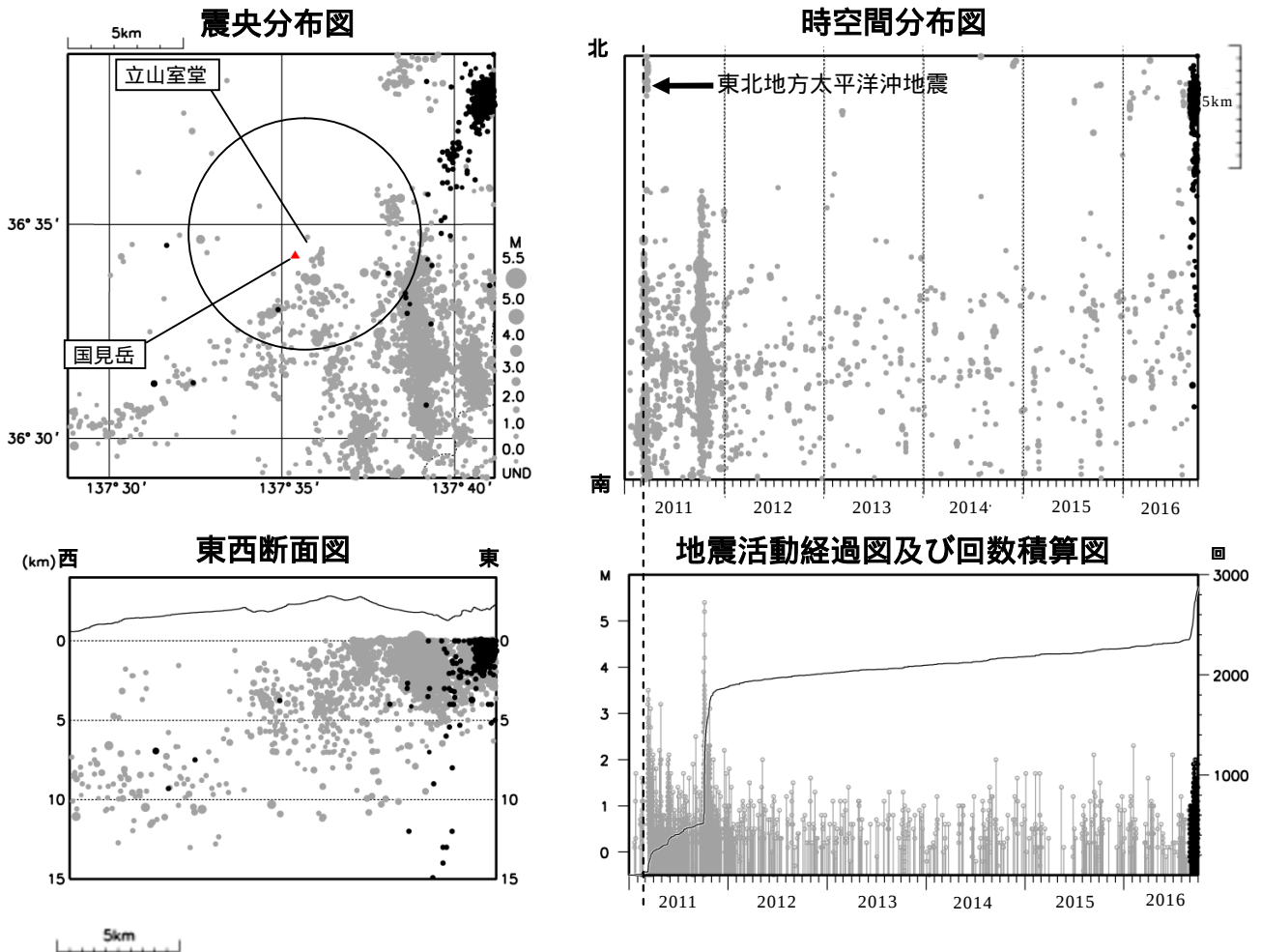
図 2 弥陀ヶ原 広域地震観測網による山体・周辺の地震活動（2011 年 1 月 1 日～2016 年 9 月 30 日）
