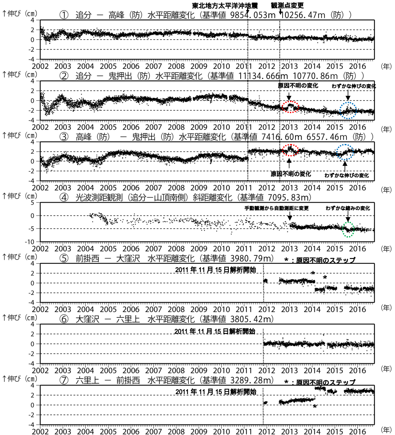
図6 浅間山 GNSS 連続観測及び光波測距観測の結果(2002年1月1日~2016年9月30日) GNSSの2010年10月以降のデータについては、電離層の影響を補正する等、解析方法を改良しました。(防)は国立研究開発法人防災科学技術研究所の観測機器を示しています。 ~ は図7の ~ にそれぞれ対応しています。 ~ の空白部分は欠測を示しています。 ・赤丸で示す変化は原因不明ですが、火山活動に起因するものではないと考えられます。 ・2015年5月頃からみられていたわずかな伸び(青丸で示す変化)の傾向が、10月頃から停滞しています。 2002年1月1日~2012年7月31日 気象庁の高峰-鬼押観測点間の基線長。 2012年8月1日~ 防災科学技術研究所の高峰-鬼押出観測点間の基線長。 光波測距観測は、2013年1月より手動観測から自動測距による観測に変更しました。 ・2015年6月頃からみられていた山頂と追分の間の縮みの傾向(緑丸で示す変化)が、10月頃から停滞しています。
