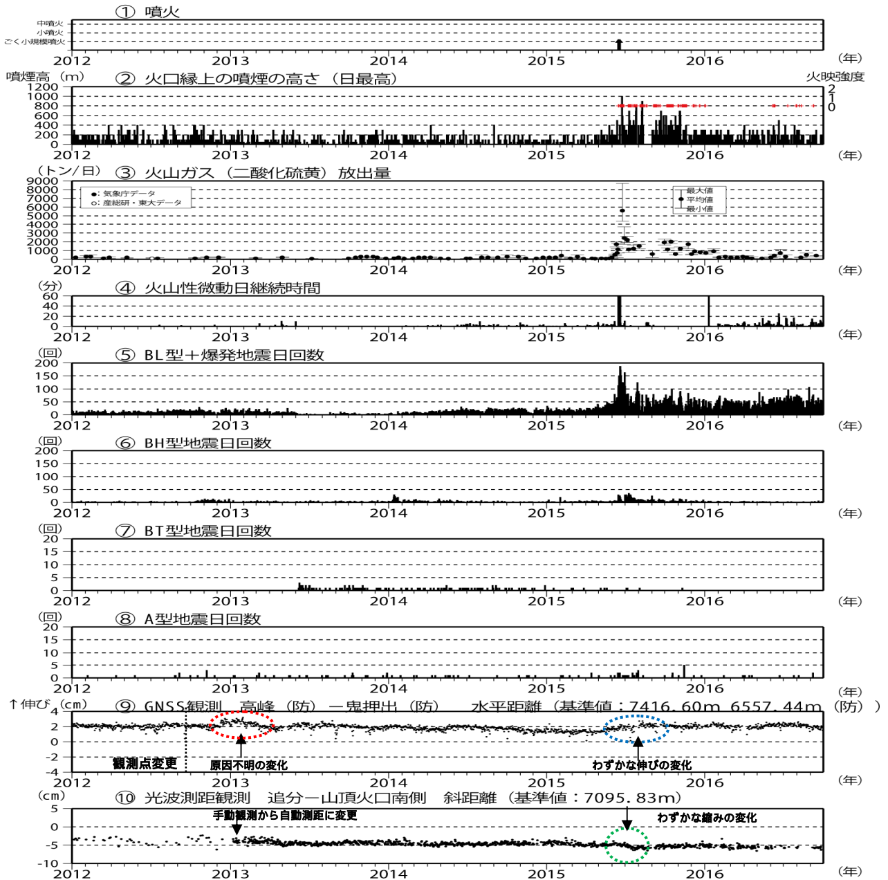
図4 浅間山 最近の火山活動経過図(2012年1月1日~2016年9月30日)
