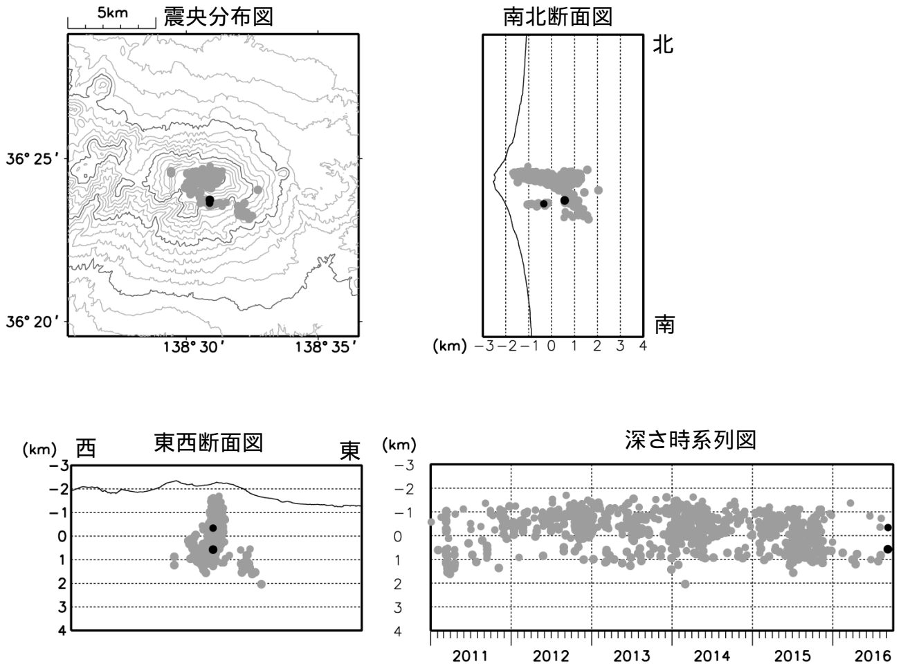
図5 浅間山 震源分布図(2011年1月1日~2016年9月30日)
