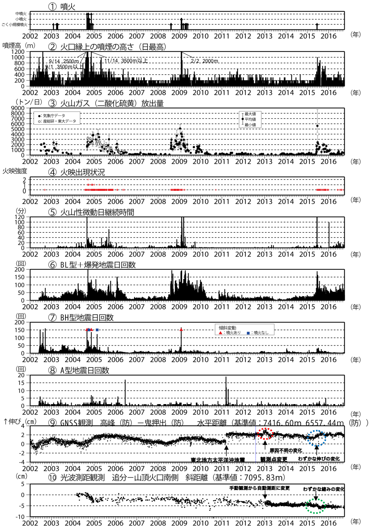
図3 浅間山 火山活動経過図 (2002年1月1日~2016年9月30日)
