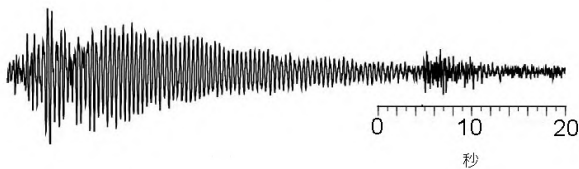
図9 浅間山で見られる火山性地震の特徴と波形例
