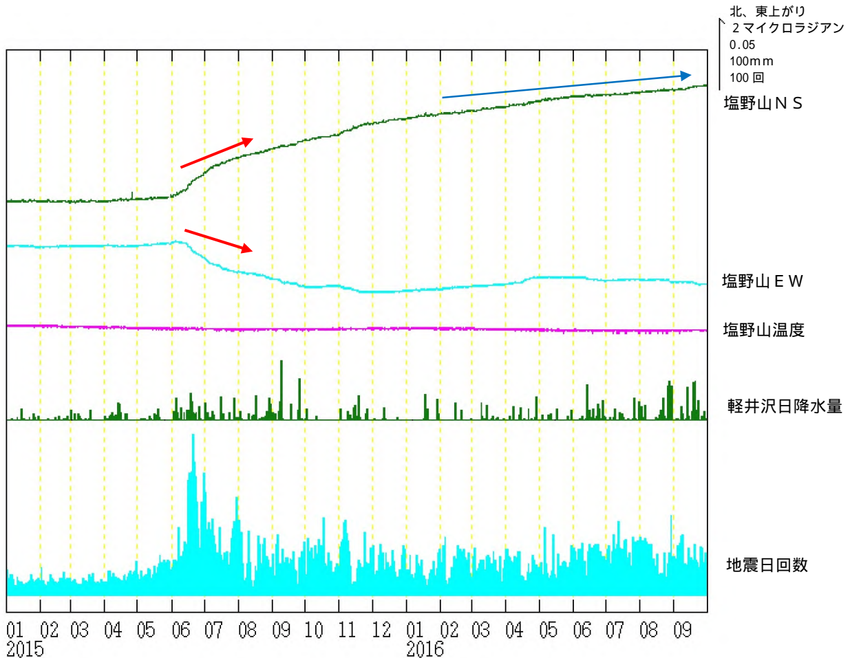
図8 浅間山 塩野山観測点における傾斜データ(2015年1月1日~2016年9月30日)
