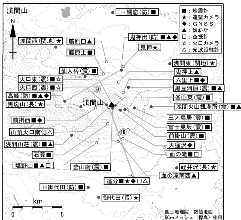
図10 浅間山 観測点配置図
