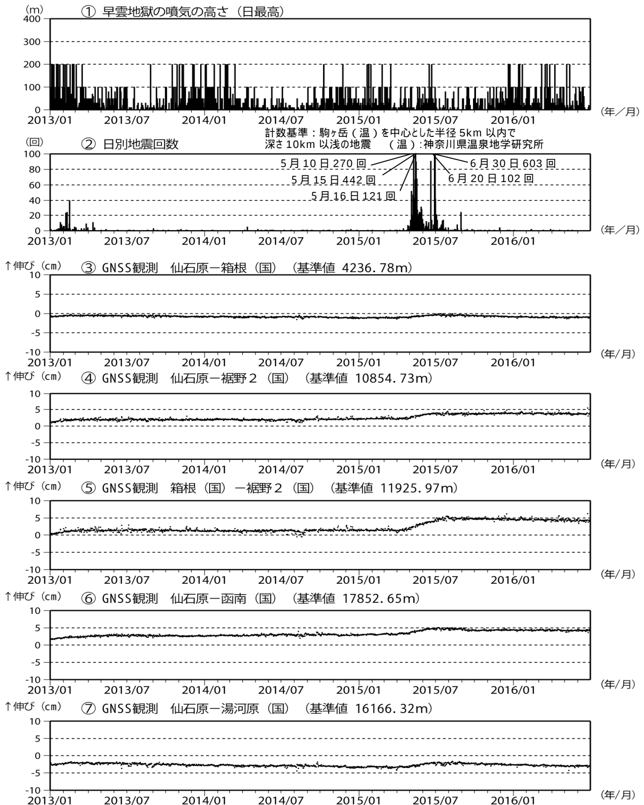
図6 箱根山 火山活動経過図（2013年1月1日～2016年6月30日）
