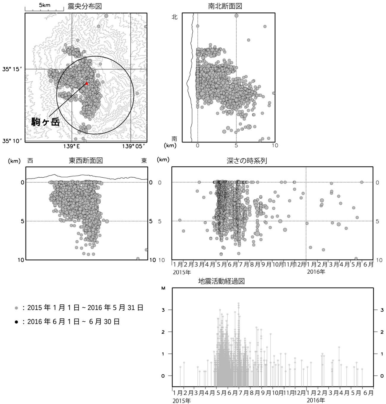
図 7 箱根山 広域地震観測網による山体周辺の震源分布図(2015 年 1 月 1 日 ~ 2016 年 6 月 30 日)
