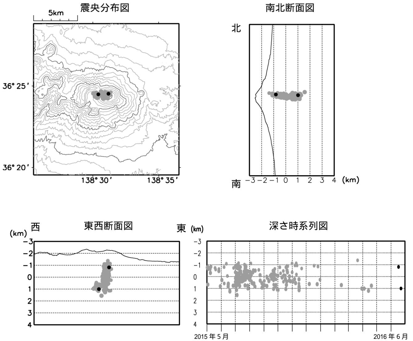
図4 浅間山 震源分布図(2015年5月1日~2016年6月30日)
