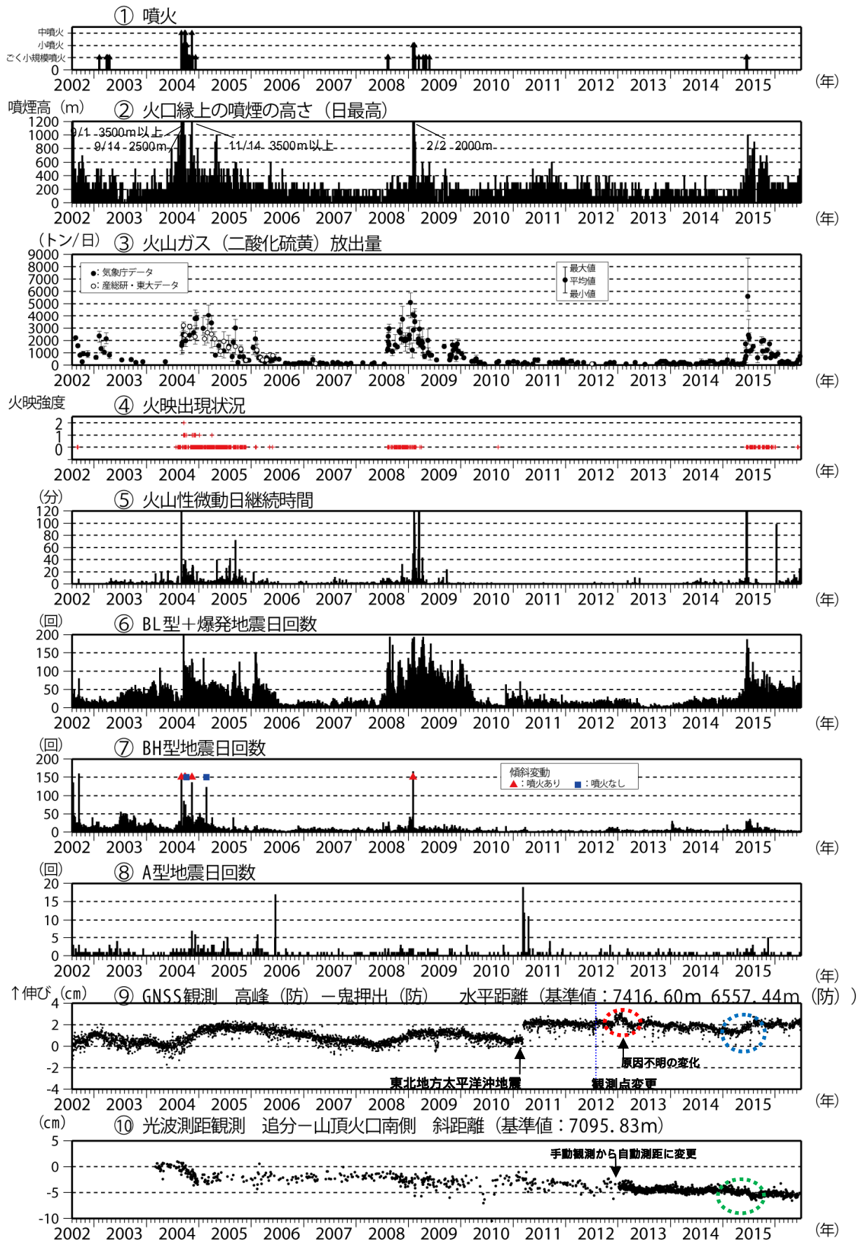
図2 浅間山 火山活動経過図 (2002年1月1日~2016年6月30日)
