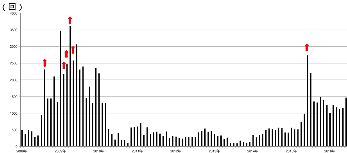
図6 浅間山 火山性地震の月別回数（2008年1月～2016年6月） ・6月の月回数は1,467回（5月は1,164回）でした。 ・赤矢印は噴火のあった月を示しています。
