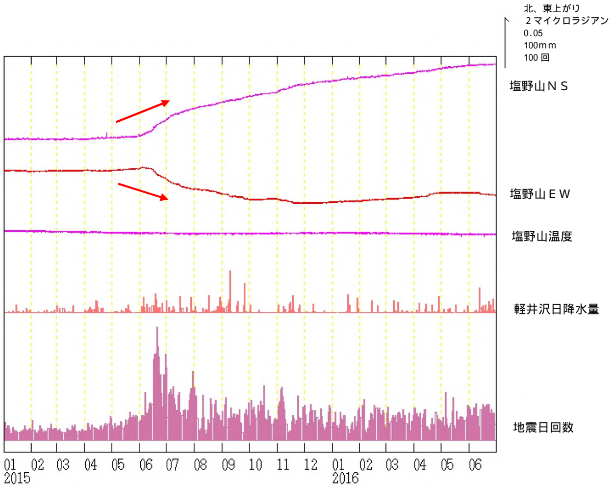
図 9 浅間山 塩野山観測点における傾斜データ(2015 年 4 月 1 日~2016 年 6 月 30 日)
