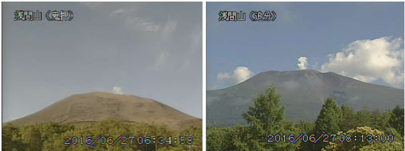
図 1 浅間山 山頂部の噴煙の状況
