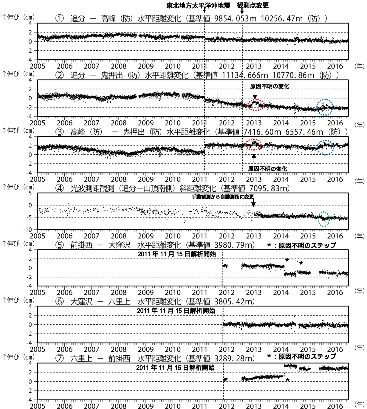
図7 浅間山 GNSS 連続観測及び光波測距観測の結果(2005年1月1日~2016年6月30日)
