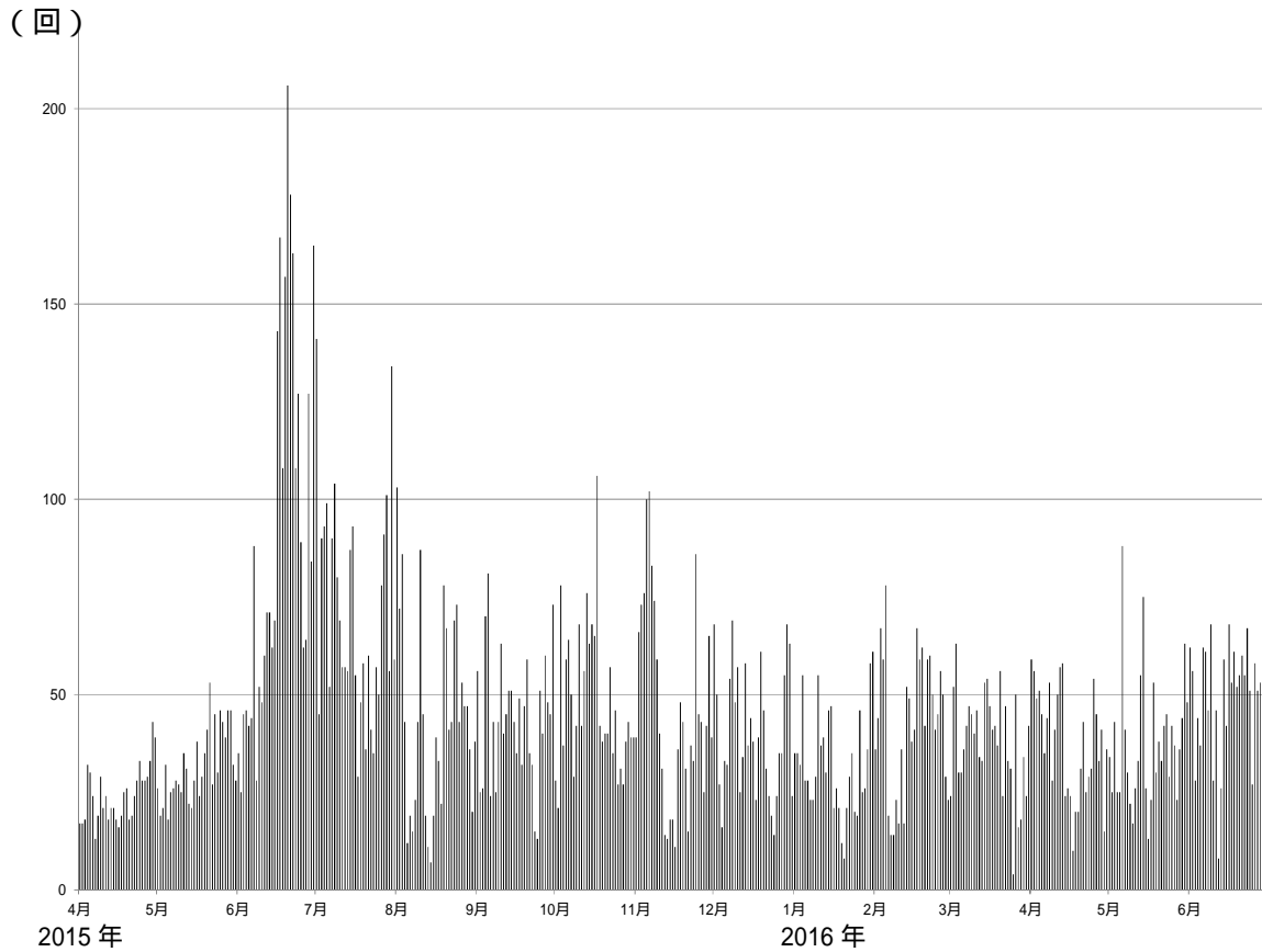
図5 浅間山 火山性地震の日別回数（2015年4月1日～2016年6月30日） ・2015年4月下旬頃から増加し6月以降多い状態で経過していました。12月頃から減少し、やや多い状態で経過しています。 ・6月の日回数の最多は9日、16日の68回（5月の日回数の最多は88回）でした。
