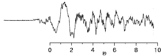
図10 浅間山で見られる火山性地震の特徴と波形例
