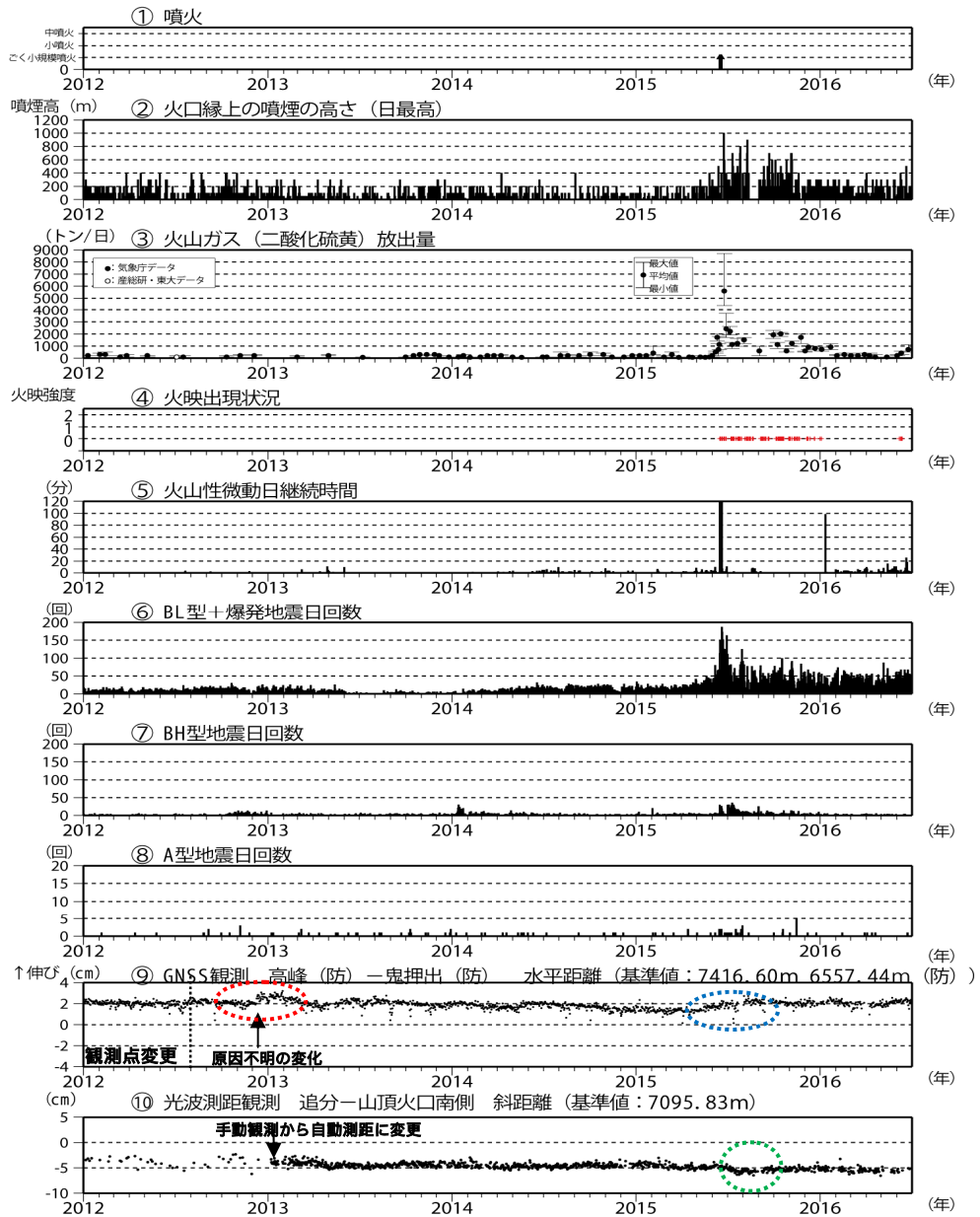
図3 浅間山 最近の火山活動経過図(2012年1月1日~2016年6月30日)
