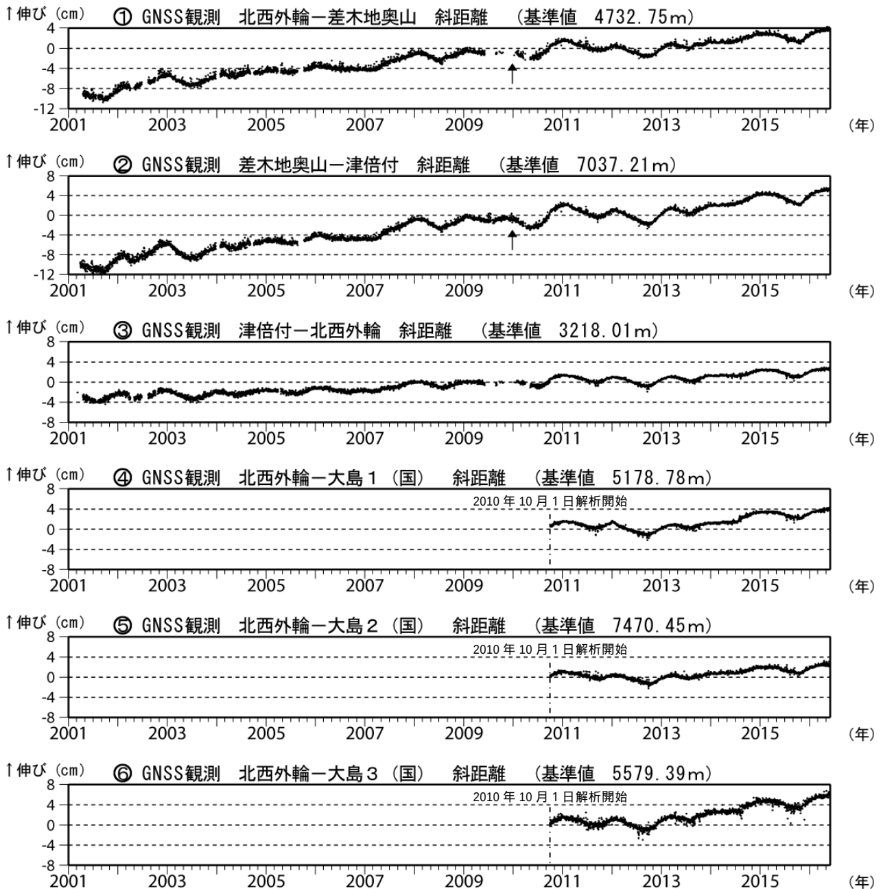
図3 伊豆大島 GNSS連続観測による基線長変化(2001年1月~2016年5月31日)(国): 国土地理院
