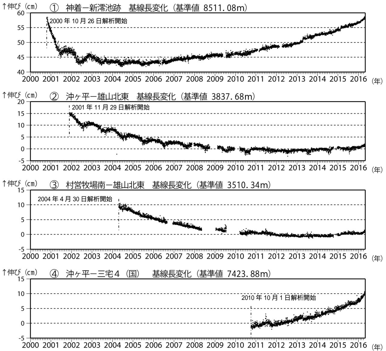
図6 三宅島 GNSS 連続観測結果 (2000年10月26日~2016年4月30日) (国): 国土地理院 ・基線 ~ は図9 (観測点配置図) の ~ にそれぞれ対応します。 ・グラフの空白部分は欠測を示します。 ・2010年10月以降のデータについては、電離層の影響を補正する等、解析方法を改良しています。
