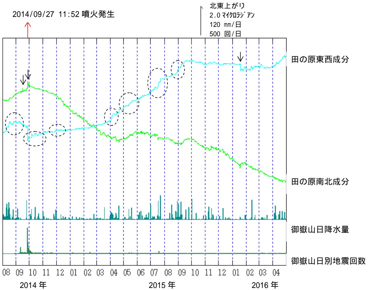
図5 御嶽山 田の原観測点(剣ヶ峰山頂の南東約3 km)の傾斜変動 (2014年8月1日~2016年4月30日)
