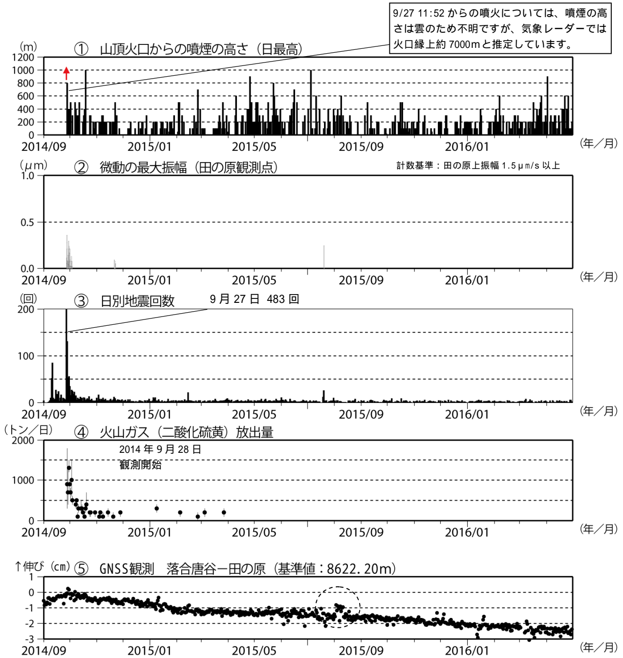
図3 御嶽山 最近の火山活動経過図(2014年9月1日~2016年4月30日)
