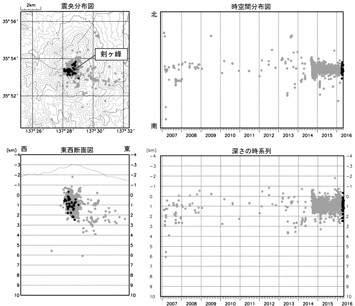
図 2 御嶽山 震源分布図（2006 年 12 月 1 日～2016 年 4 月 30 日）
