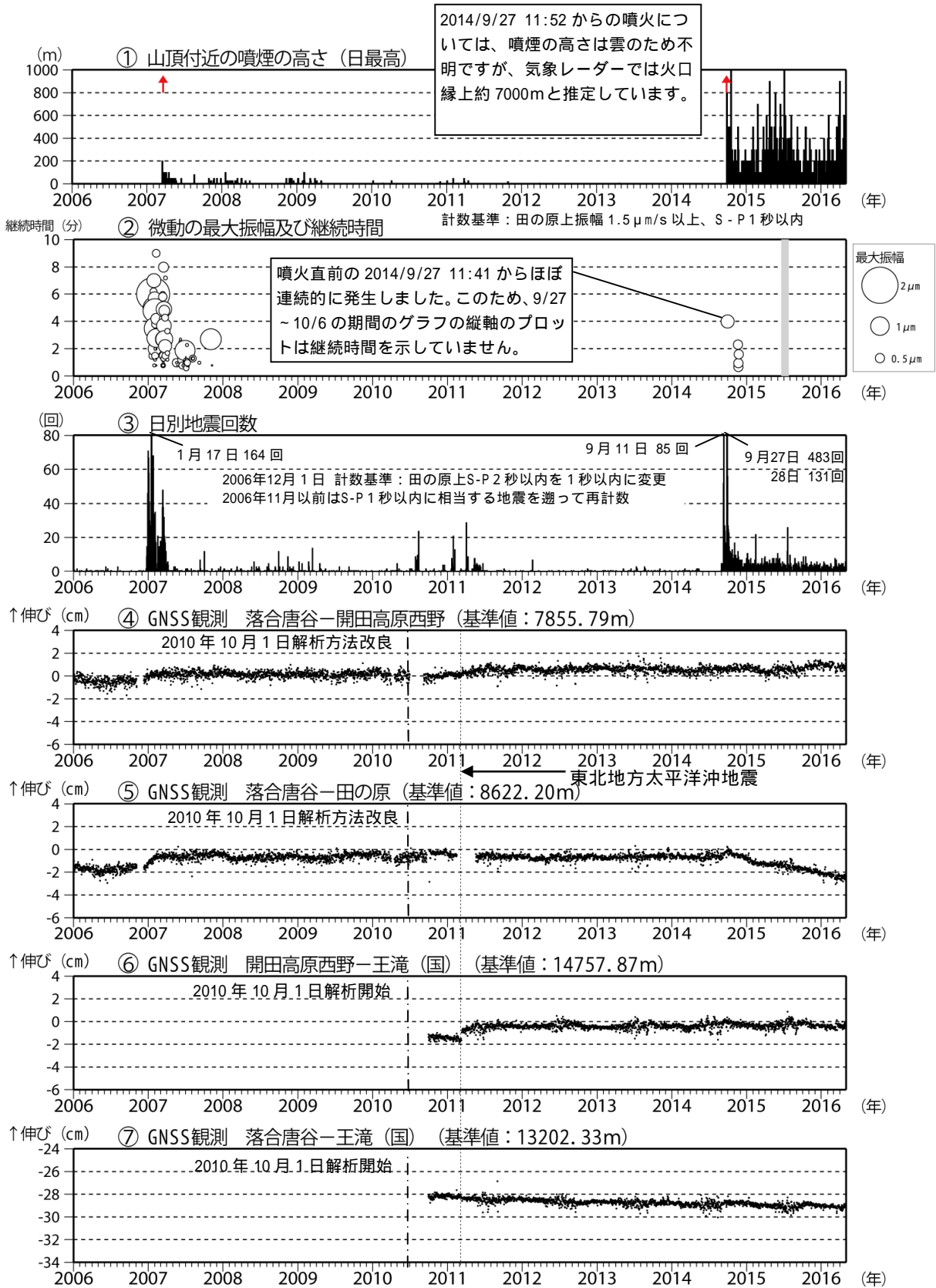
図4 御嶽山 長期間の火山活動経過図(2006年1月1日~2016年4月30日)
