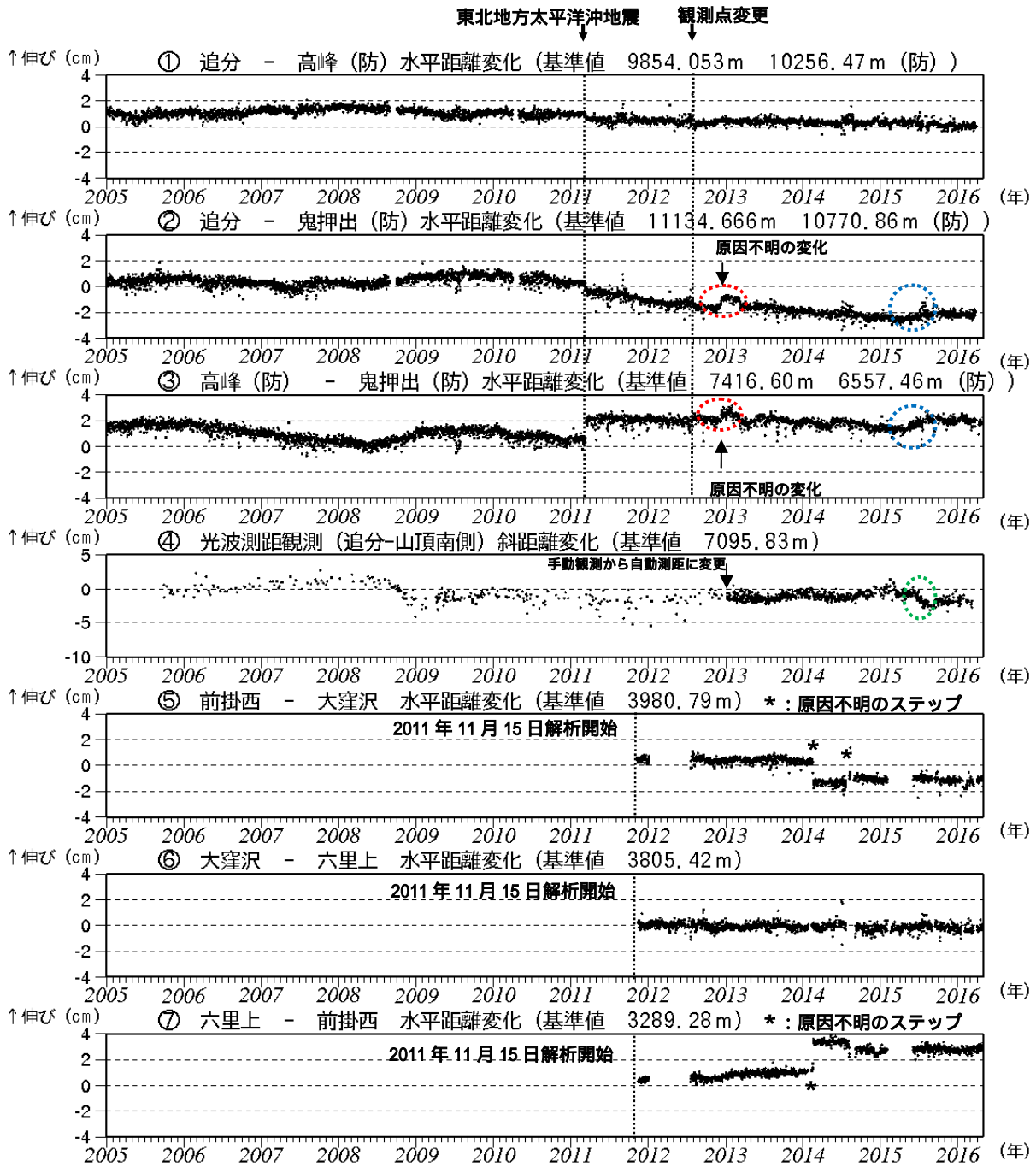
図7 浅間山 GNSS 連続観測及び光波測距観測の結果(2005年1月1日~2016年4月30日) GNSSの2010年10月以降のデータについては、電離層の影響を補正する等、解析方法を改良しました。(防)は国立研究開発法人防災科学技術研究所の観測機器を示しています。
