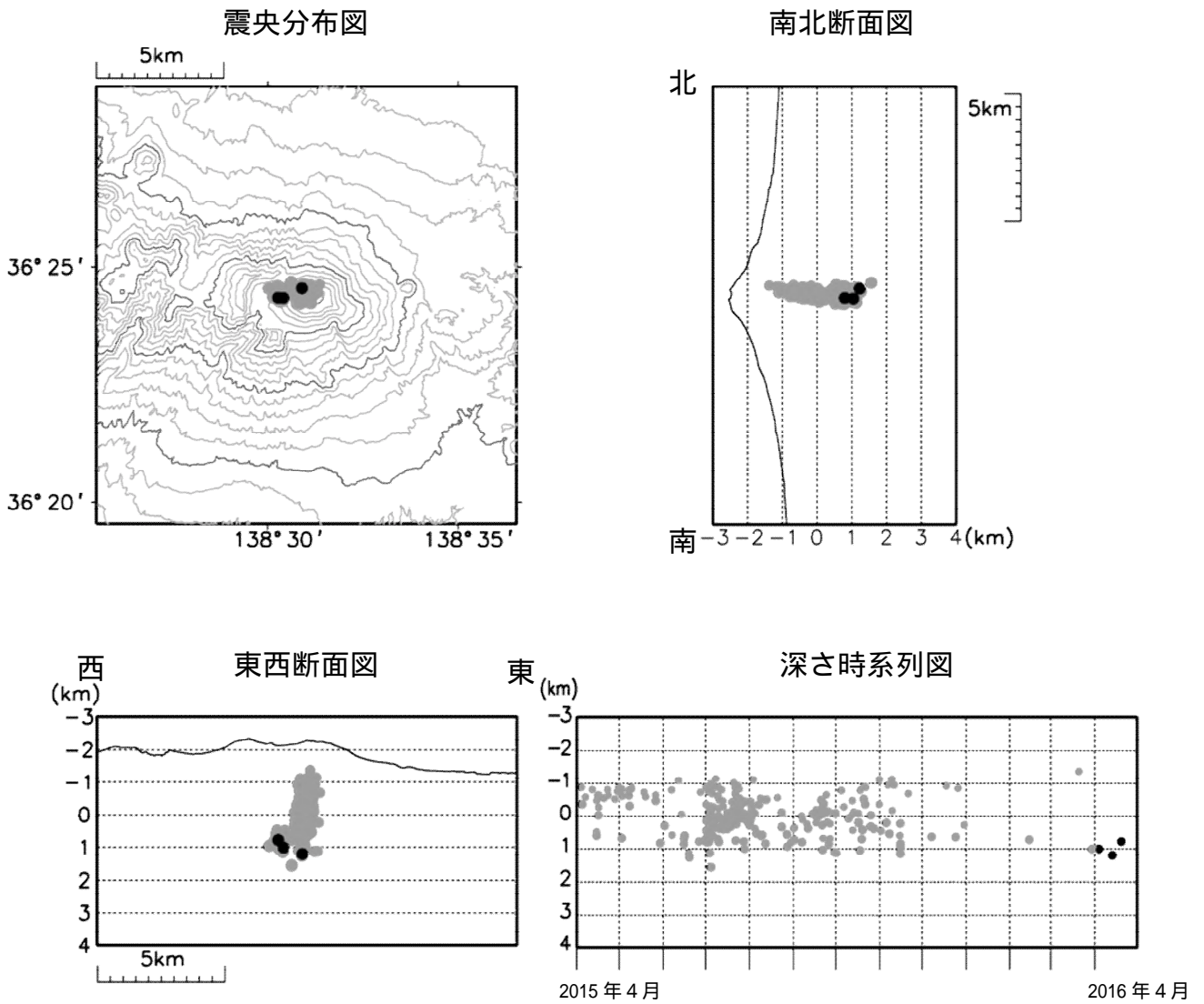
図 4 浅間山 震源分布図 (2015 年 4 月 1 日 ~ 2016 年 4 月 30 日)
