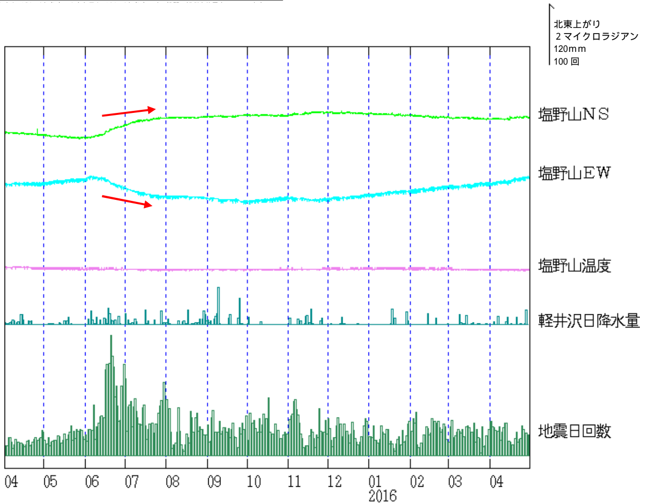
図 9 浅間山 塩野山観測点における傾斜データ(2015年4月1日~2016年4月30日)
