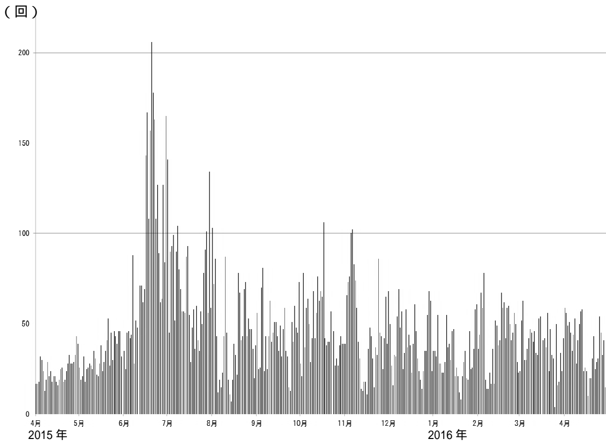
図5 浅間山 火山性地震の日別回数（2015年4月1日～2016年4月30日） ・2015年4月下旬頃から増加し6月以降多い状態で経過していました。12月頃から減少し、やや多い状態で経過しています。 ・4月の日回数の最多は1日の59回（3月の日回数の最多は63回）でした。
