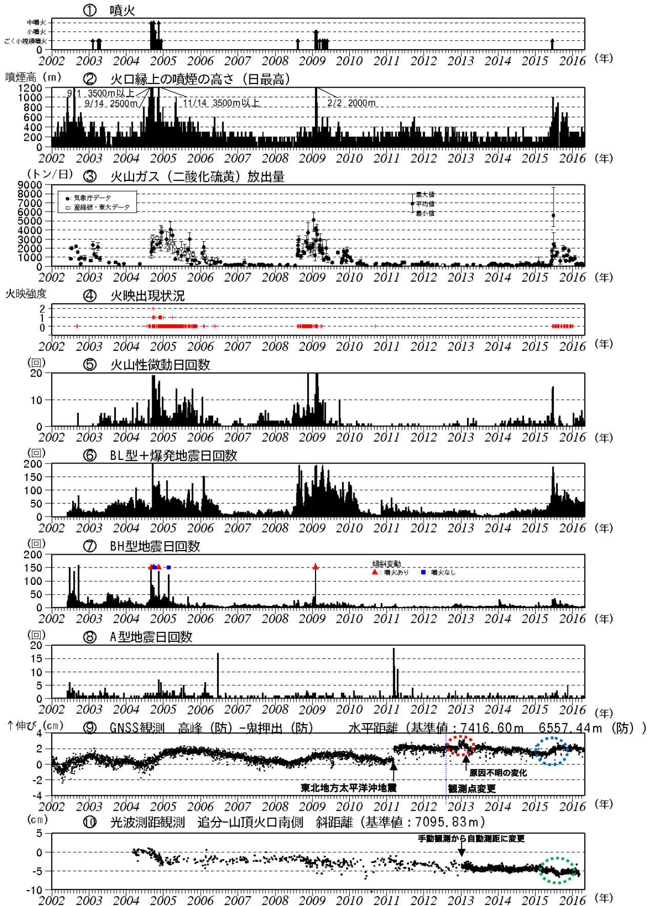
図2 浅間山 火山活動経過図(2002年1月1日~2016年4月30日)
