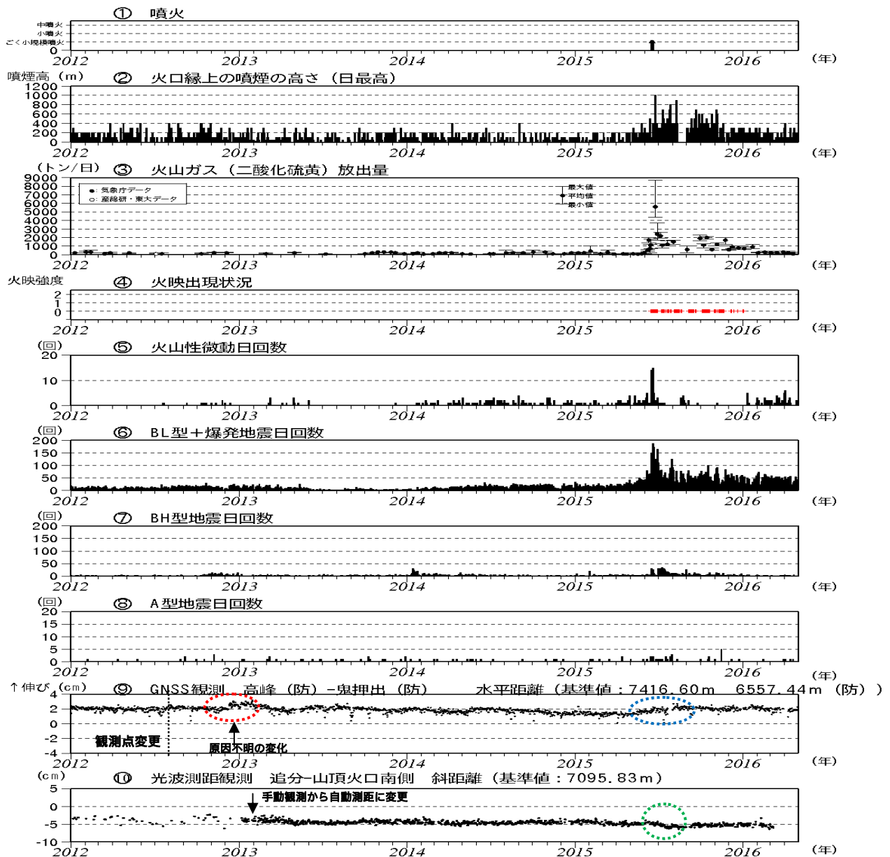
図3 浅間山 最近の火山活動経過図(2012年1月1日~2016年4月30日)
