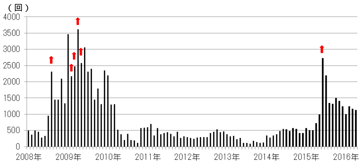
図6 浅間山 火山性地震の月別回数（2008年1月～2016年4月） ・4月の月回数は1,133回（3月は1,175回）でした。 ・赤矢印は噴火のあった月を示しています。
