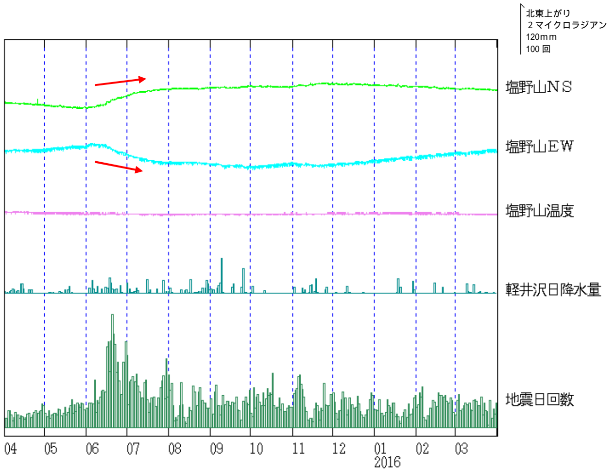
図 9 浅間山 塩野山観測点における傾斜データ(2015 年 4 月 1 日 ~ 2016 年 3 月 31 日)
