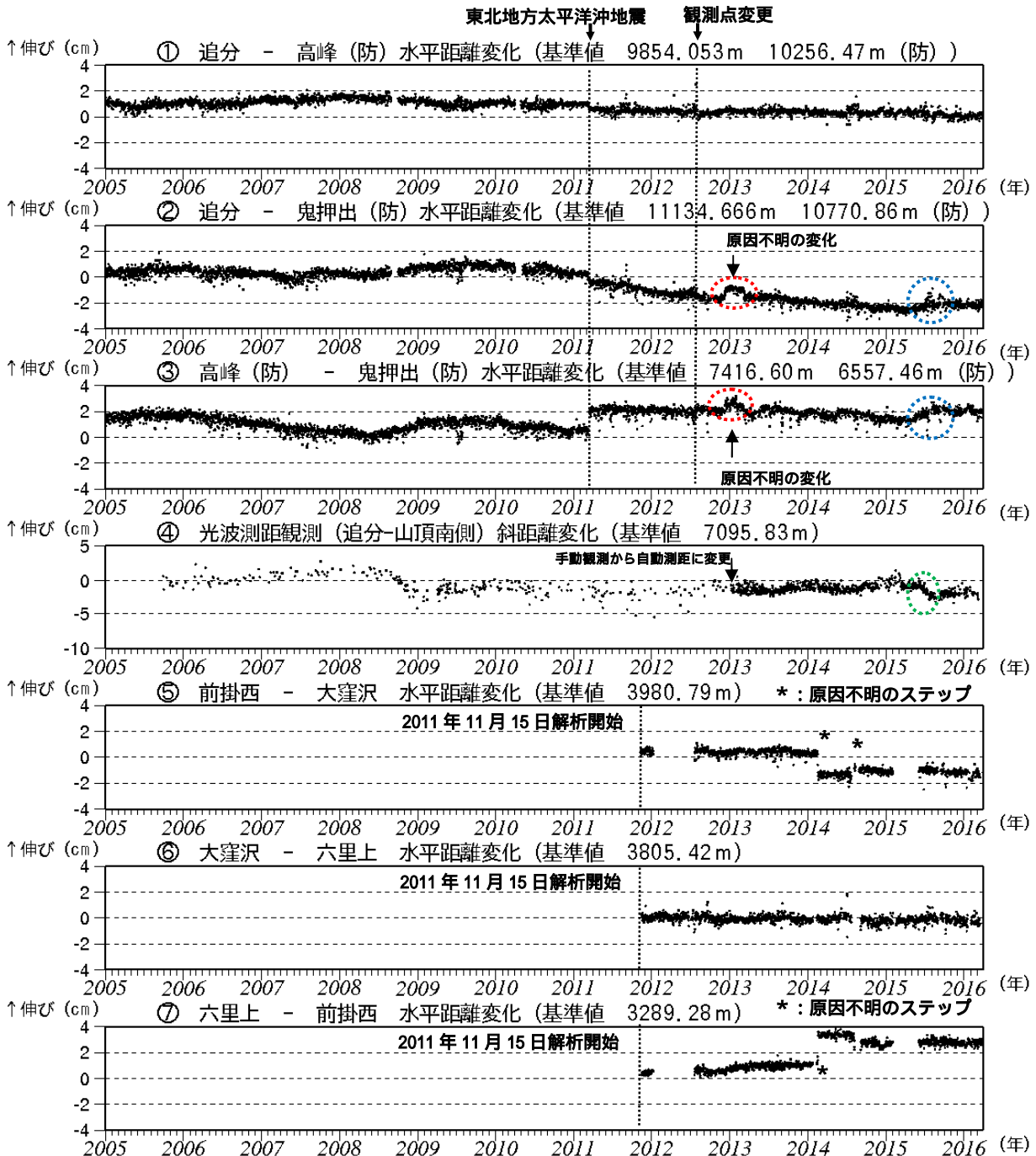
図7 浅間山 GNSS連続観測及び光波測距観測の結果(2005年1月1日~2016年3月31日) GNSSの2010年10月以降のデータについては、電離層の影響を補正する等、解析方法を改良しました。(防)は国立研究開発法人防災科学技術研究所の観測機器を示しています。
