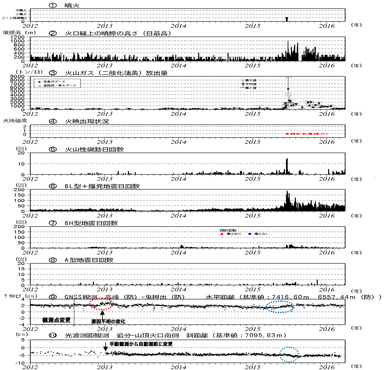
図3 浅間山 最近の火山活動経過図(2012年1月1日~2016年3月31日)
