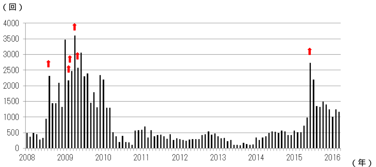
図6 浅間山 火山性地震の月別回数（2008年1月～2016年3月） ・3月の月回数は1,175回（2月は1,247回）でした。 ・赤矢印は噴火のあった月を示しています。
