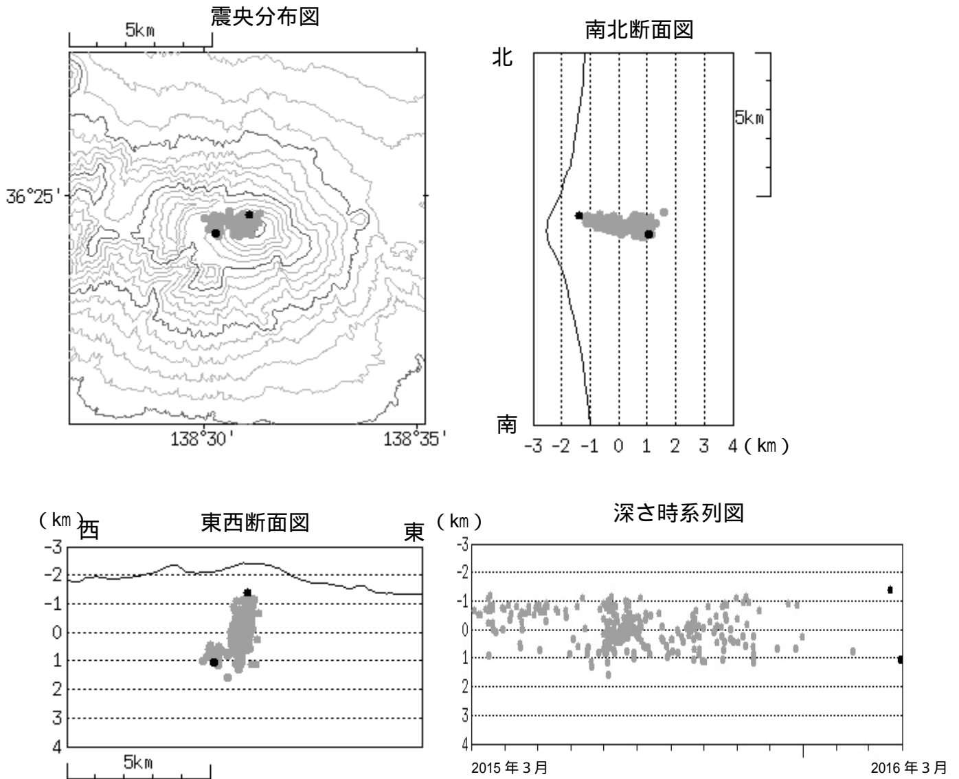
図4 浅間山 震源分布図(2015年3月1日~2016年3月31日)
