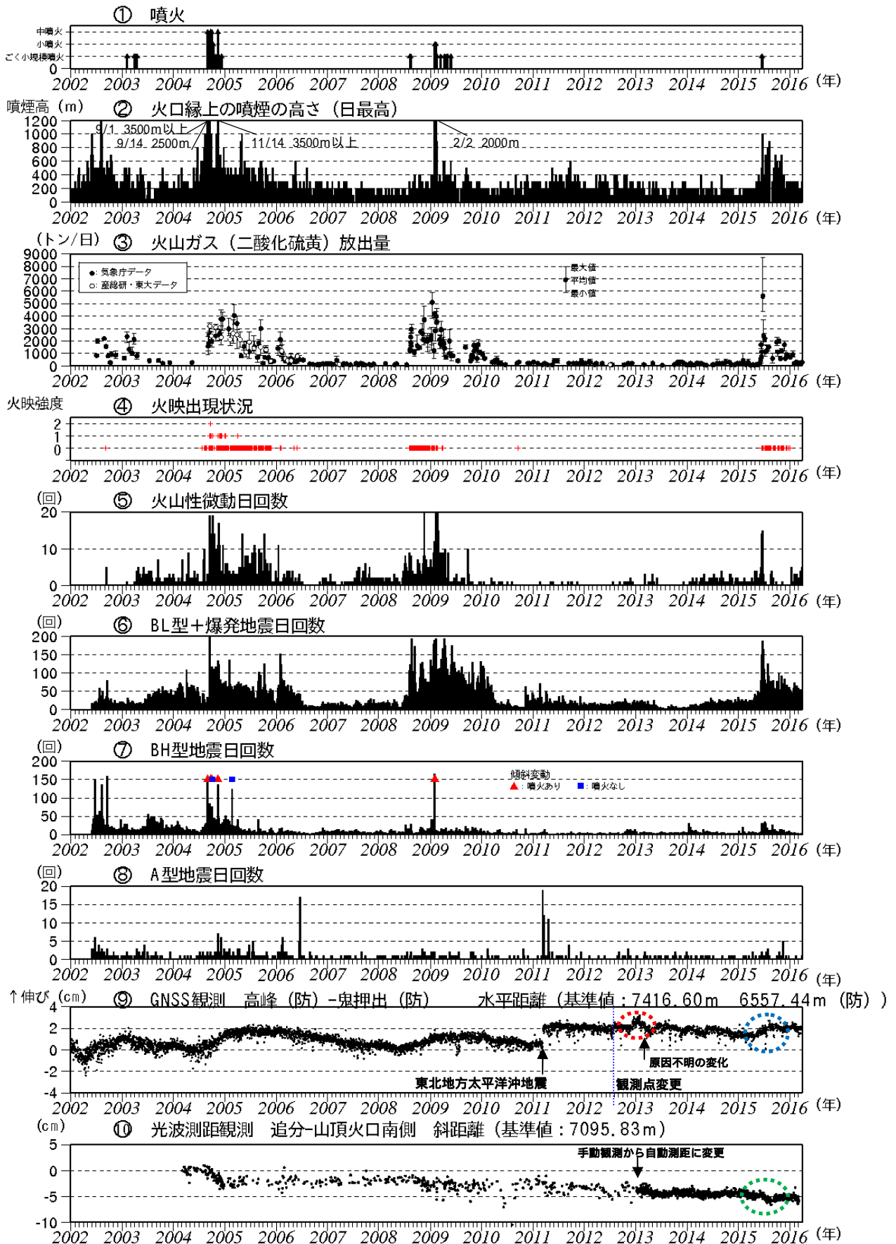
図2 浅間山 火山活動経過図 (2002年1月1日~2016年3月31日)
