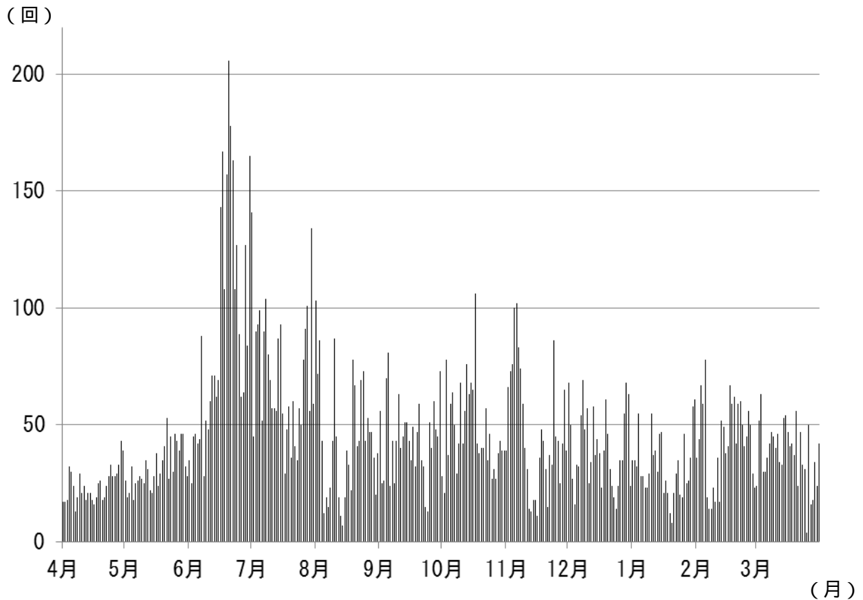
図5 浅間山 火山性地震の日別回数（2015年4月1日～2016年3月31日） ・2015年4月下旬頃から増加し6月以降多い状態で経過していました。12月頃から減少し、やや多い状態で経過しています。 ・3月の日回数の最多は3日の63回（2月の日回数の最多は78回）でした。
