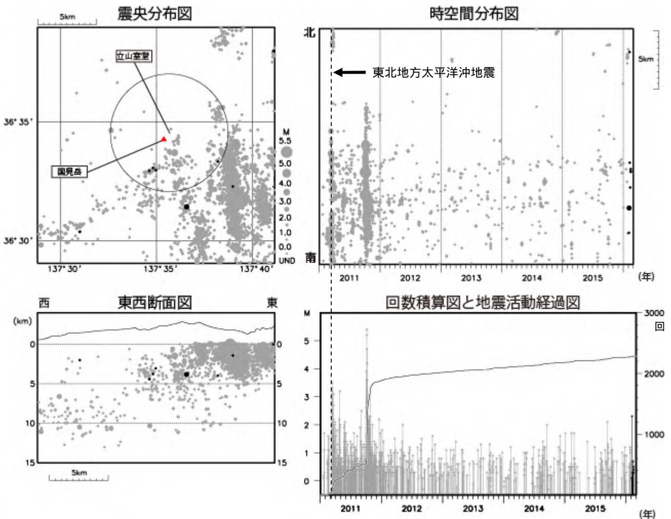
図2 弥陀ヶ原 広域地震観測網による山体・周辺の地震活動(2011年2月1日~2016年2月29日) : 2011年1月1日~2016年1月31日 : 2016年2月1日~2月29日 ・ 震央分布図内の円は、立山室堂に設置した地震計(立山室堂2)で地震回数を計数しているS-P時間1秒以内となるおよその範囲を示します。 ・ M(マグニチュード)は地震の規模を表します。 ・ 図中の震源要素は一部暫定値が含まれており、後日変更することがあります。 ・ 弥陀ヶ原近傍の地震活動は、低調に経過しています。
