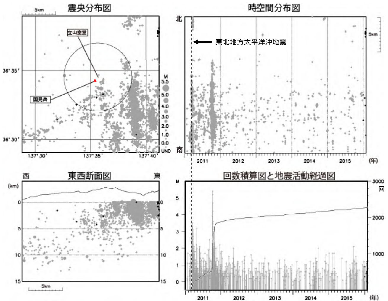
図2 弥陀ヶ原 広域地震観測網による山体・周辺の地震活動(2011年1月1日~2016年1月31日) : 2011年1月1日~2015年12月31日 : 2016年1月1日~1月31日 ・ 震央分布図内の円は、立山室堂に設置した地震計(立山室堂2)で地震回数を計数しているS-P時間1秒以内となるおよその範囲を示します。 ・ M(マグニチュード)は地震の規模を表します。 ・ 図中の震源要素は一部暫定値が含まれており、後日変更することがあります。 ・ 弥陀ヶ原近傍の地震活動は、低調に経過しています。
