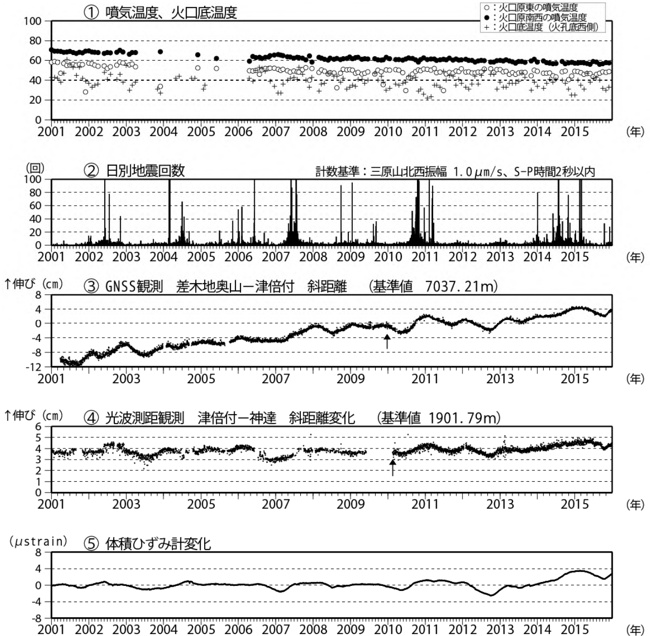
図2 伊豆大島 最近の火山活動経過図（2001年1月～2015年12月31日）
