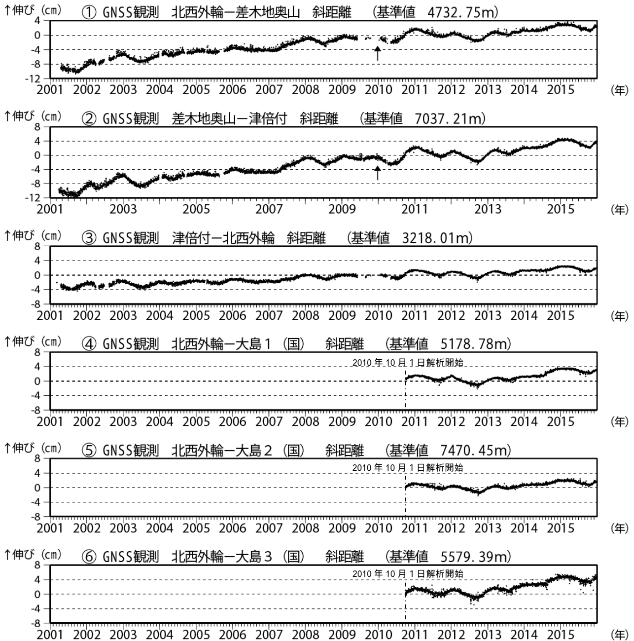
図3 伊豆大島 GNSS連続観測による基線長変化(2001年1月~2015年12月31日)(国): 国土地理院 2010年10月以降のデータについては、電離層の影響を補正する等、解析方法を改良しています。 ~ は図8のGNSS基線 ~ に対応しています。 グラフの空白部分は欠測。 の矢印は差木地奥山支柱工事を実施。 ・長期的な山体膨張に加えて約1年周期で膨張と収縮を繰り返す変動がみられています。2015年1月頃から収縮傾向がみられていましたが、10月頃から膨張傾向がみられています。
