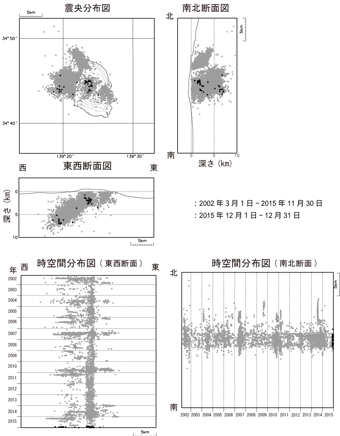
図4 伊豆大島 震源分布図(2002年3月1日~2015年12月31日)
