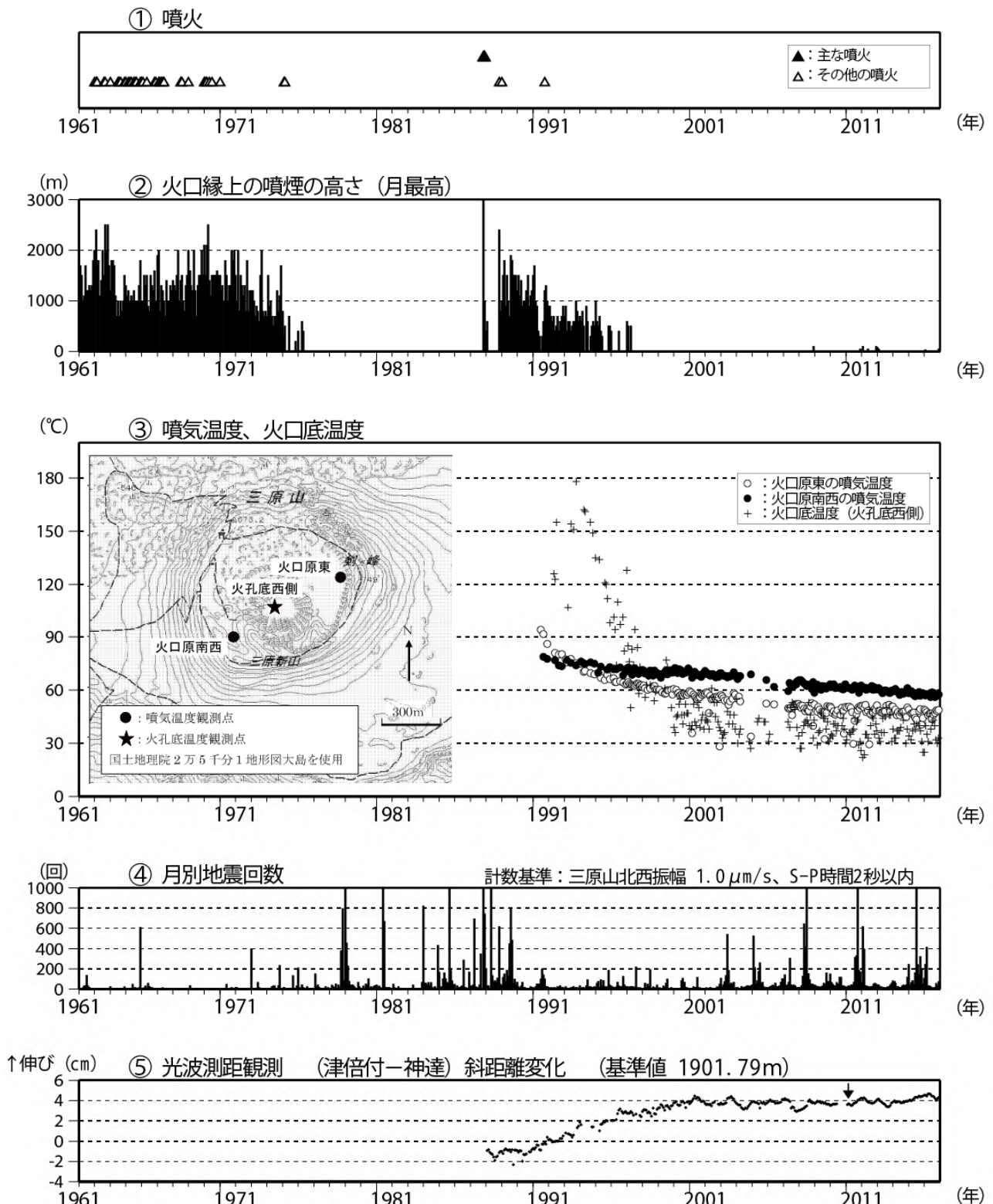
図1 伊豆大島 長期間の火山活動経過図(1961年1月~2015年12月31日)
