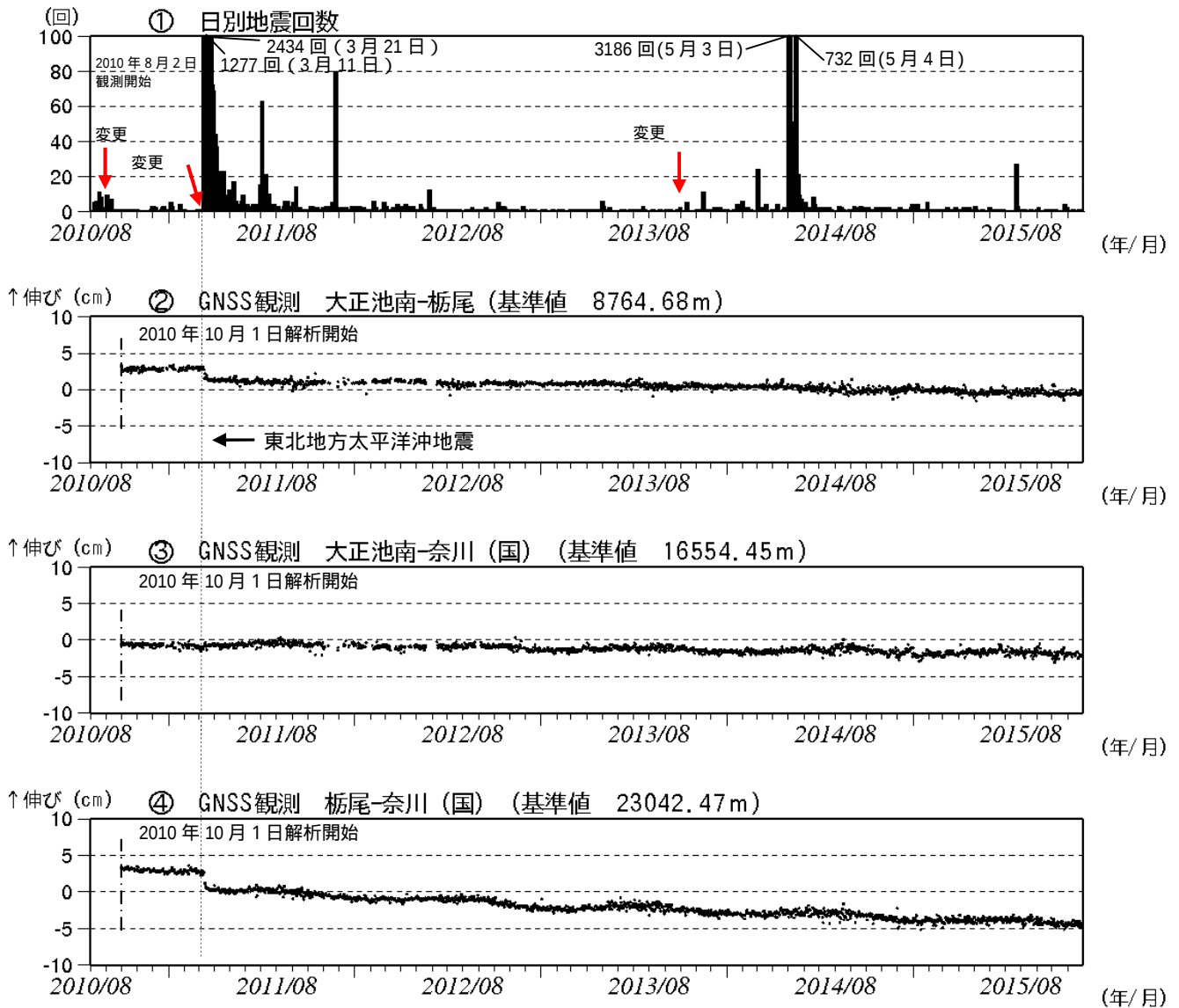
図 2 焼岳 火山活動経過図 (2010年 8 月 2 日～2015年11月30日)
