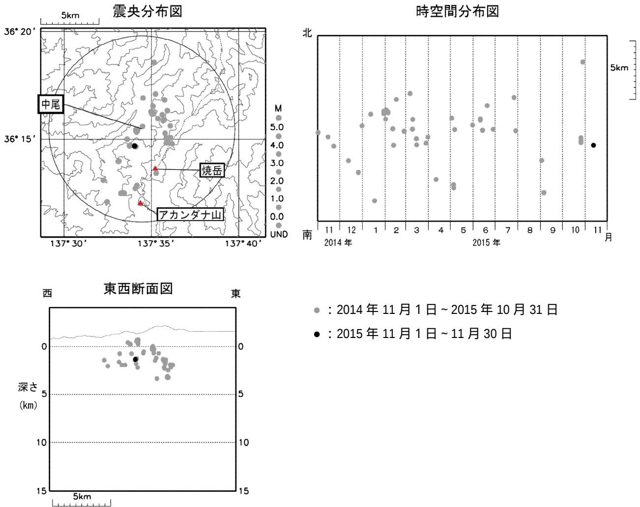
図 3 焼岳 震源分布図（2014 年 11 月 1 日～2015 年 11 月 30 日） 焼岳の地震観測点による震源分布図を示します。 震央分布図中の円は図 3 - の計数対象地震（中尾で S - P 時間 1 秒以内）のおよその範囲を示します。
