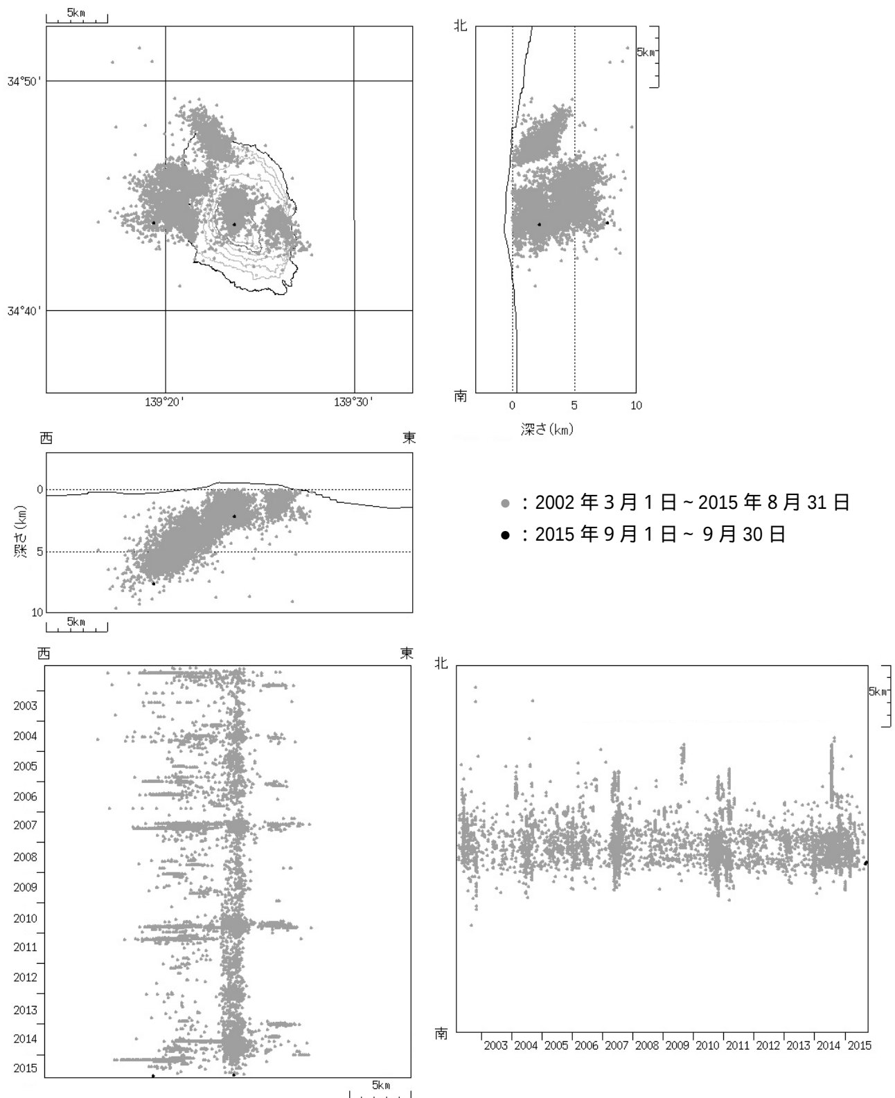
図4 伊豆大島 震源分布図（2002 年 3 月 1 日～2015 年 9 月 30 日）
