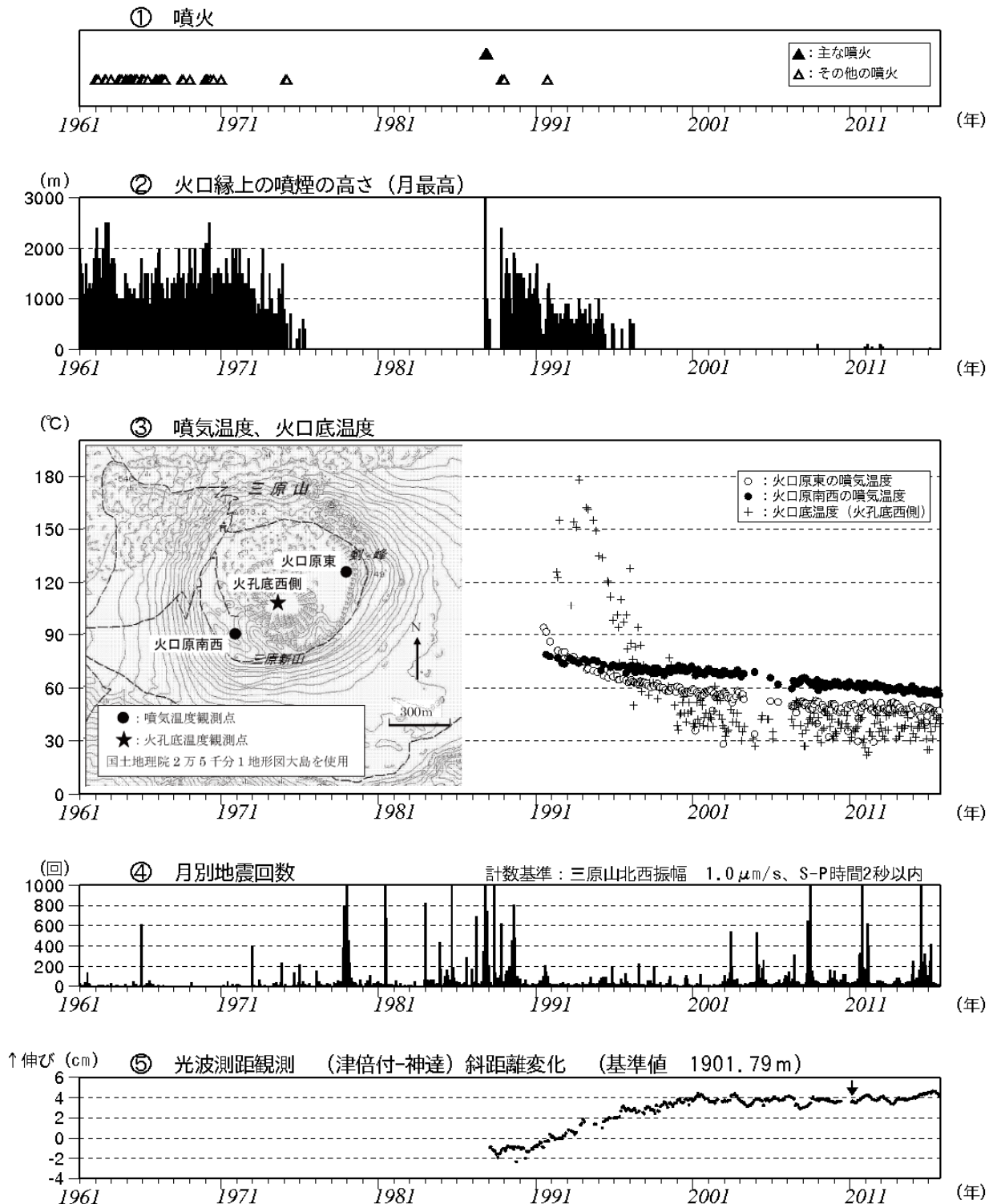
図1 伊豆大島 長期間の火山活動経過図（1961年1月～2015年9月30日）
