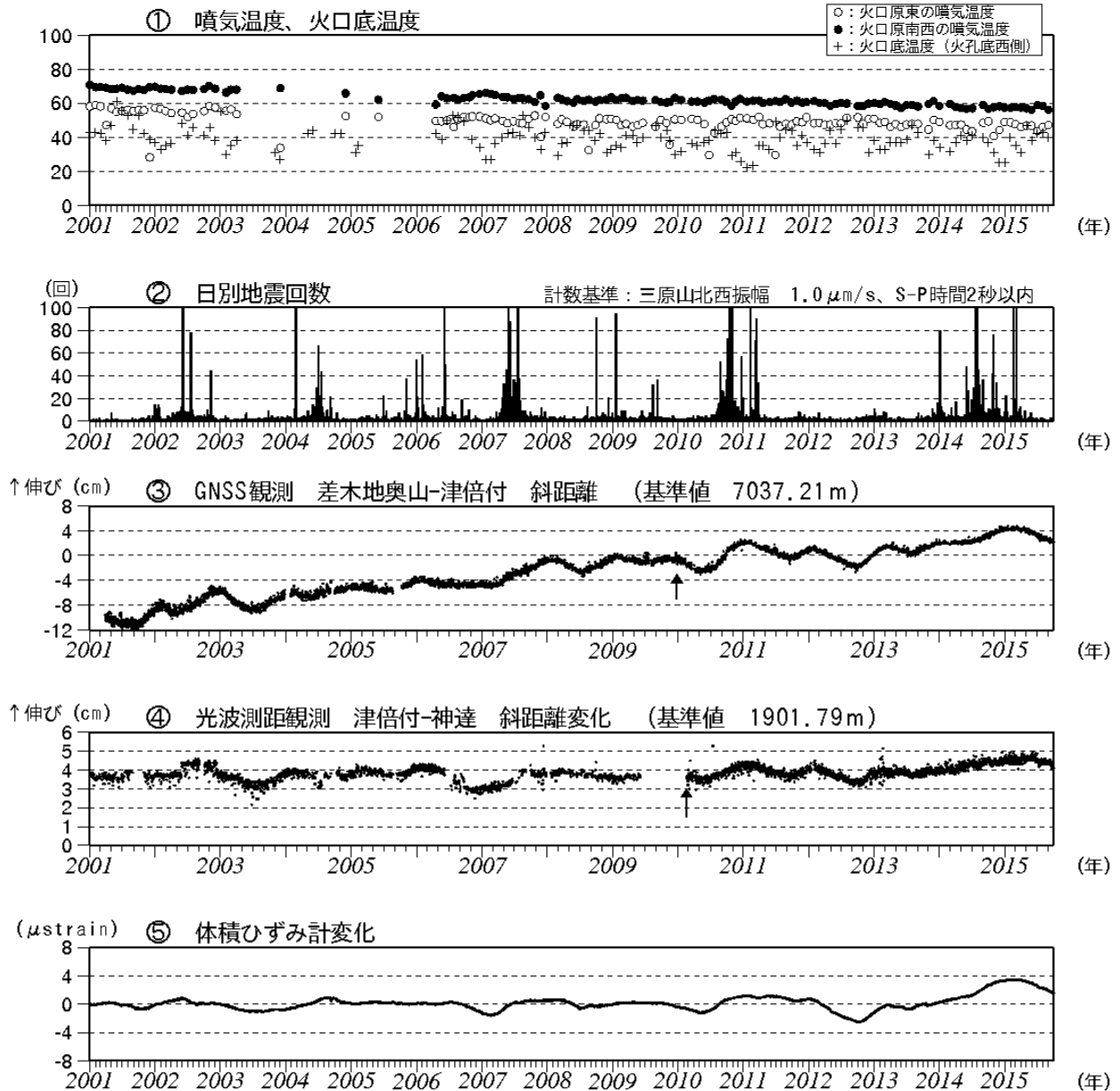
図2 伊豆大島 最近の火山活動経過図(2001年1月～2015年9月30日)
