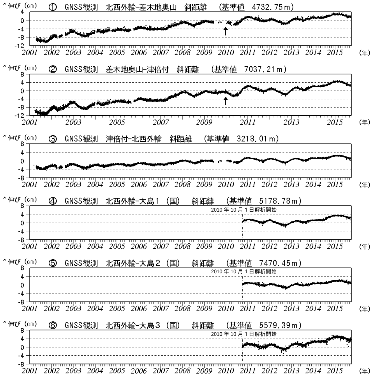
図3 伊豆大島 GNSS連続観測による基線長変化(2001年1月～2015年9月30日)(国): 国土地理院
