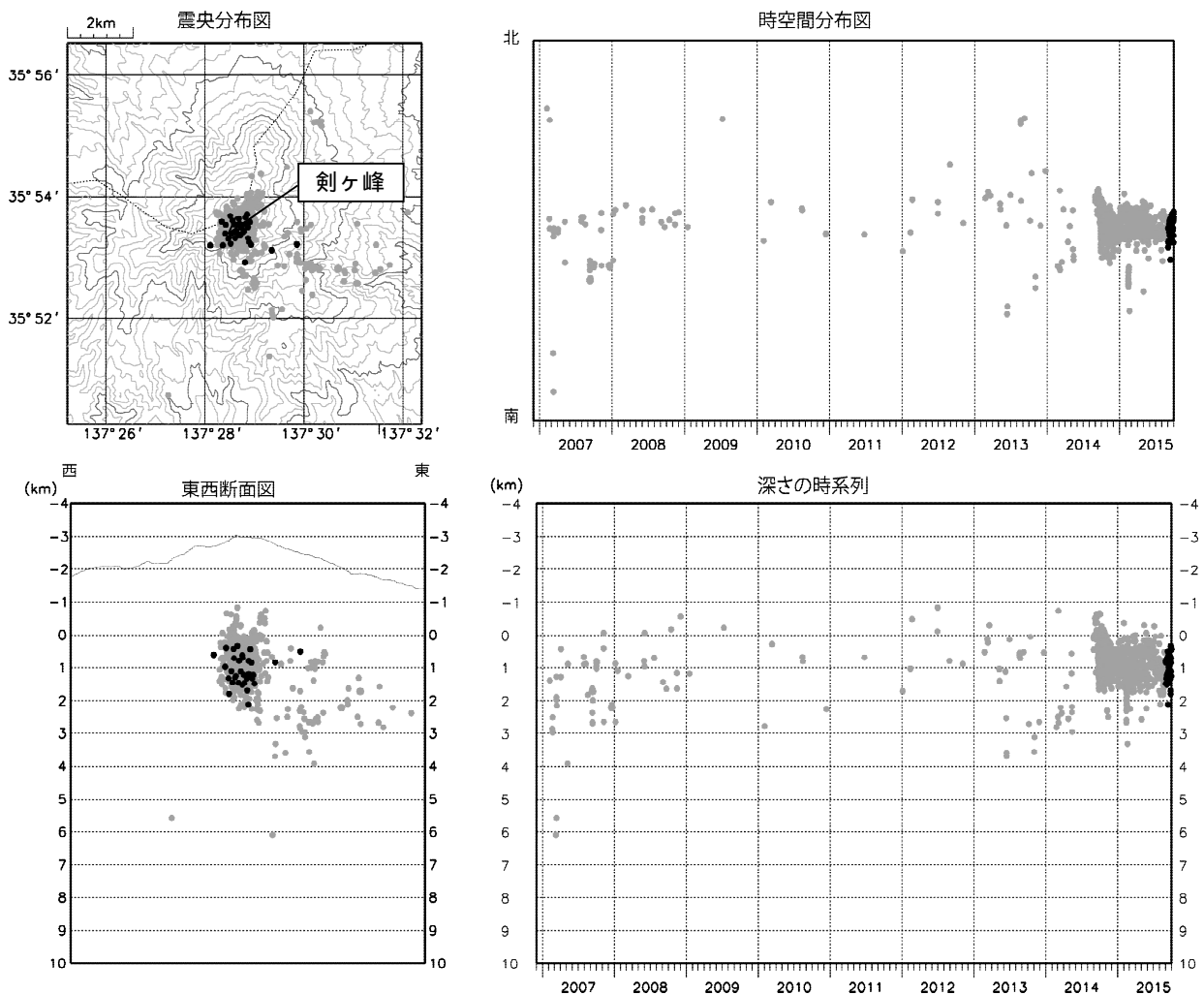
図 2 御嶽山 震源分布図（2006 年 12 月 1 日～2015 年 9 月 30 日）
