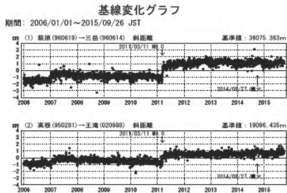
図 6 御嶽山 国土地理院による GNSS 基線変化グラフ 4)
