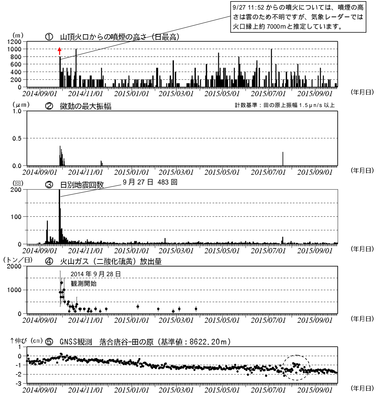
図3 御嶽山 最近の火山活動経過図(2014年8月15日~2015年9月30日)
