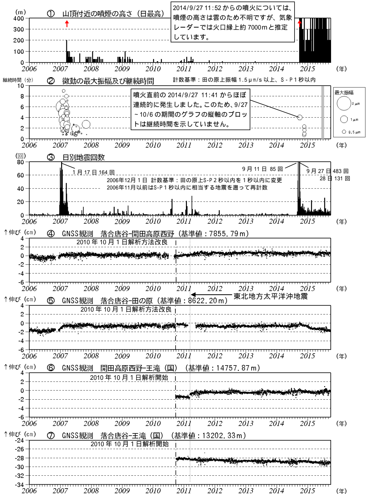
図4 御嶽山 長期間の火山活動経過図(2006年1月1日~2015年9月30日)
