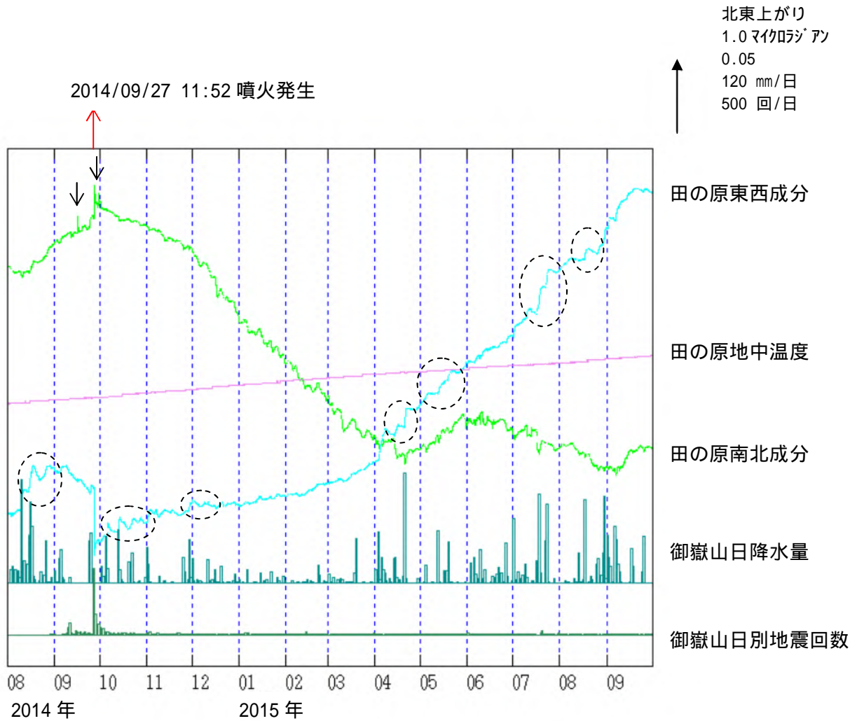
図5 御嶽山 田の原観測点(剣ヶ峰山頂の南東約3 km)の傾斜変動 (2014年8月1日~2015年9月30日)
