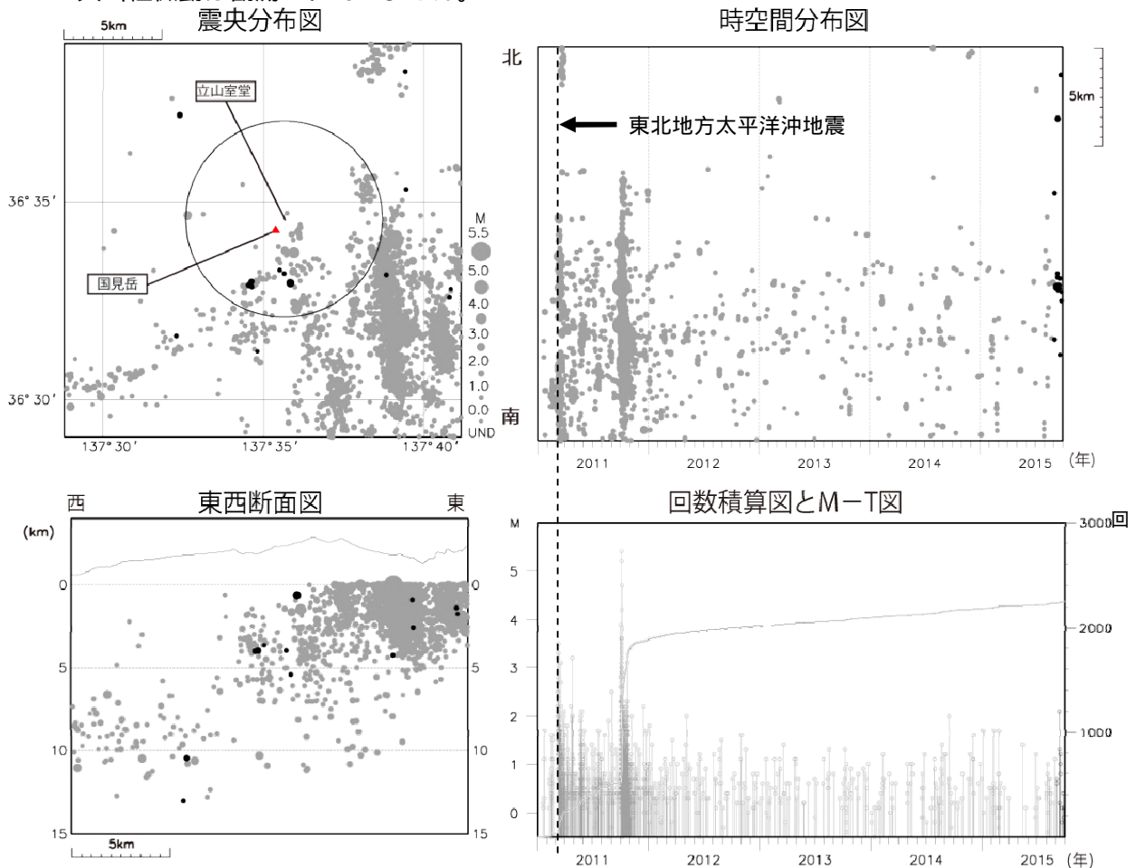
図 1 弥陀ヶ原 広域地震観測網による山体・周辺の地震活動（2011 年 1 月 1 日～2015 年 9 月 30 日） : 2011 年 1 月 1 日～2015 年 8 月 31 日 : 2015 年 9 月 1 日～9 月 30 日 ・ 震央分布図内の円は、立山室堂に設置した地震計（立山室堂 2）で地震回数を計数している S-P 時間 1 秒以内となるおおよその範囲を示します。 ・ M（マグニチュード）は地震の規模を表します。 ・ 図中の震源要素は一部暫定値が含まれており、後日変更することがあります。 ・ 弥陀ヶ原近傍の地震活動は、低調に経過しています。
