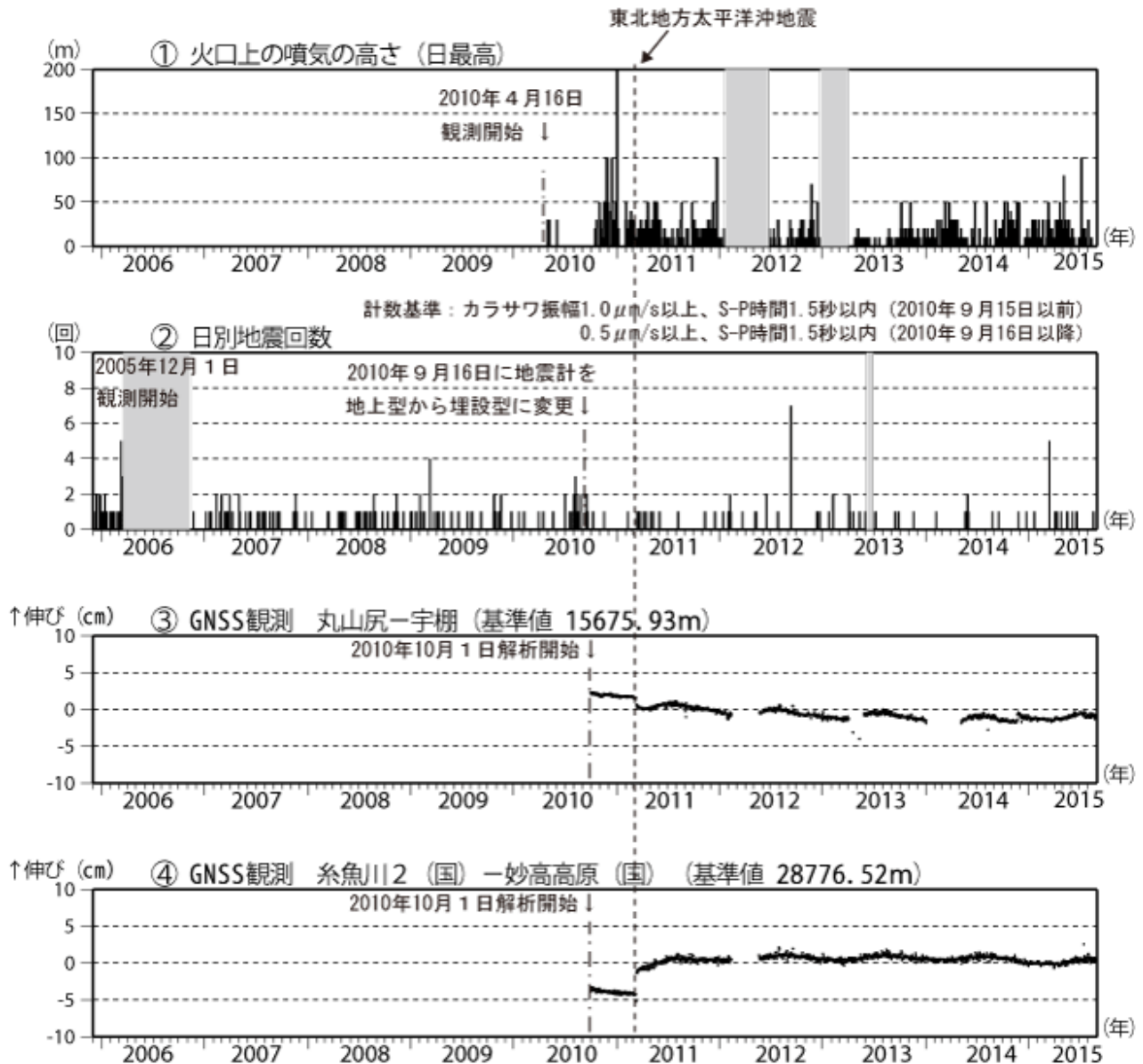
図 3 新潟焼山 火山活動経過図（2005 年 12 月 1 日～2015 年 8 月 31 日）
