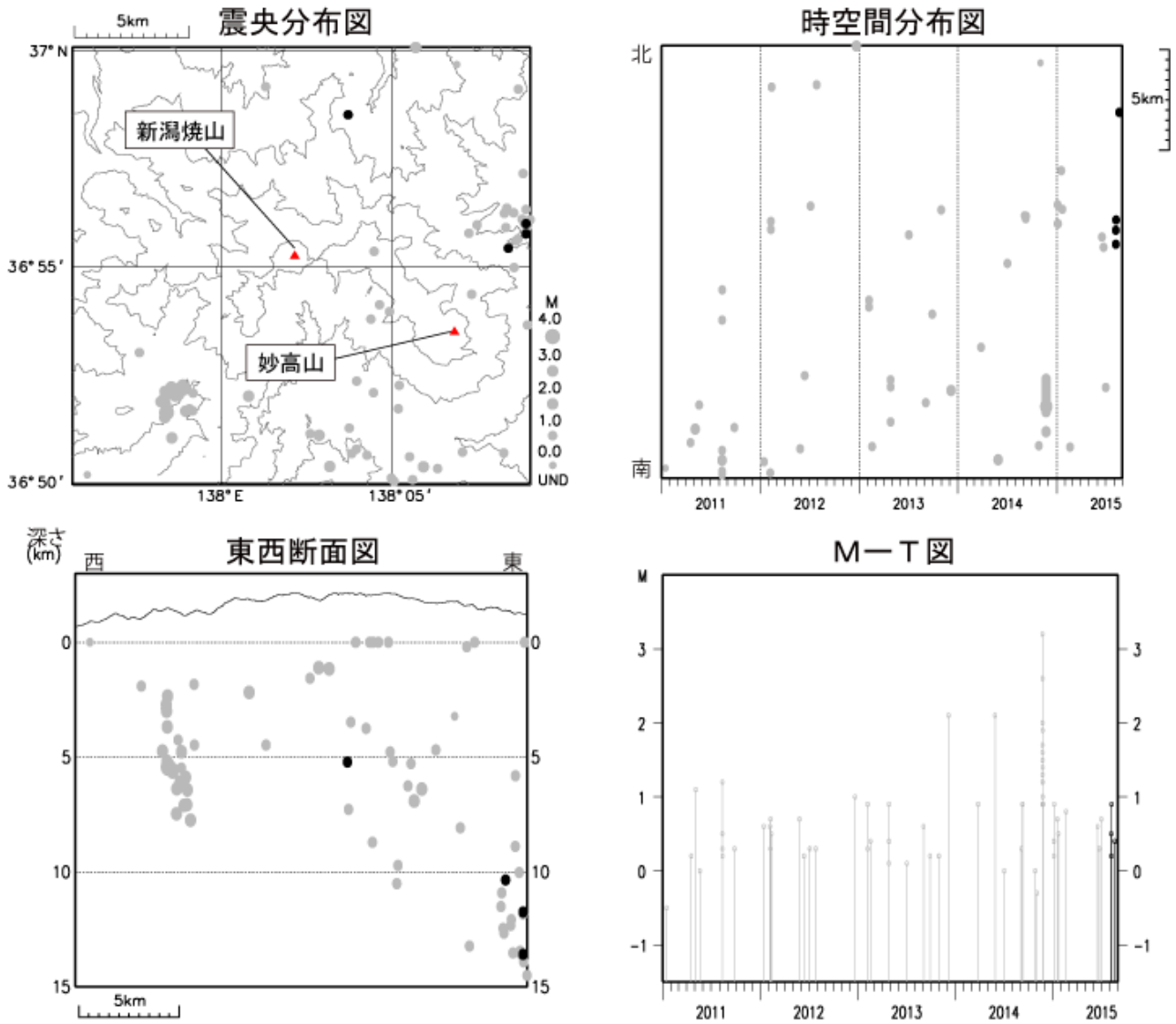
図4 新潟焼山 広域地震観測網による山体・周辺の地震活動（2011年1月1日～2015年8月31日）
