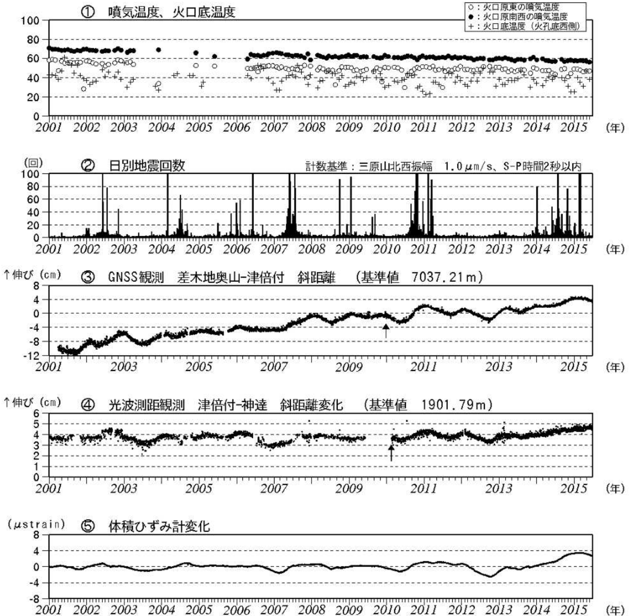
図2 伊豆大島 最近の火山活動経過図(2001年1月~2015年6月30日)
