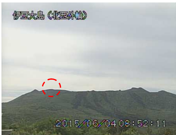
山頂部（6月4日、北西外輪遠望カメラによる） 剣ガ峰付近（6月25日、撮影方向は図7参照） 図5 伊豆大島 三原山山頂部及び山頂火口の状況 破線円内：ごく弱い噴気
