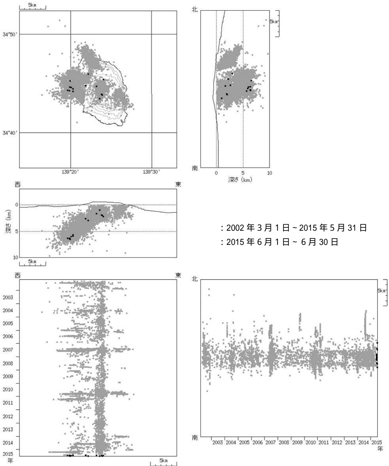
図4 伊豆大島 震源分布図(2002年3月1日~2015年6月30日)
