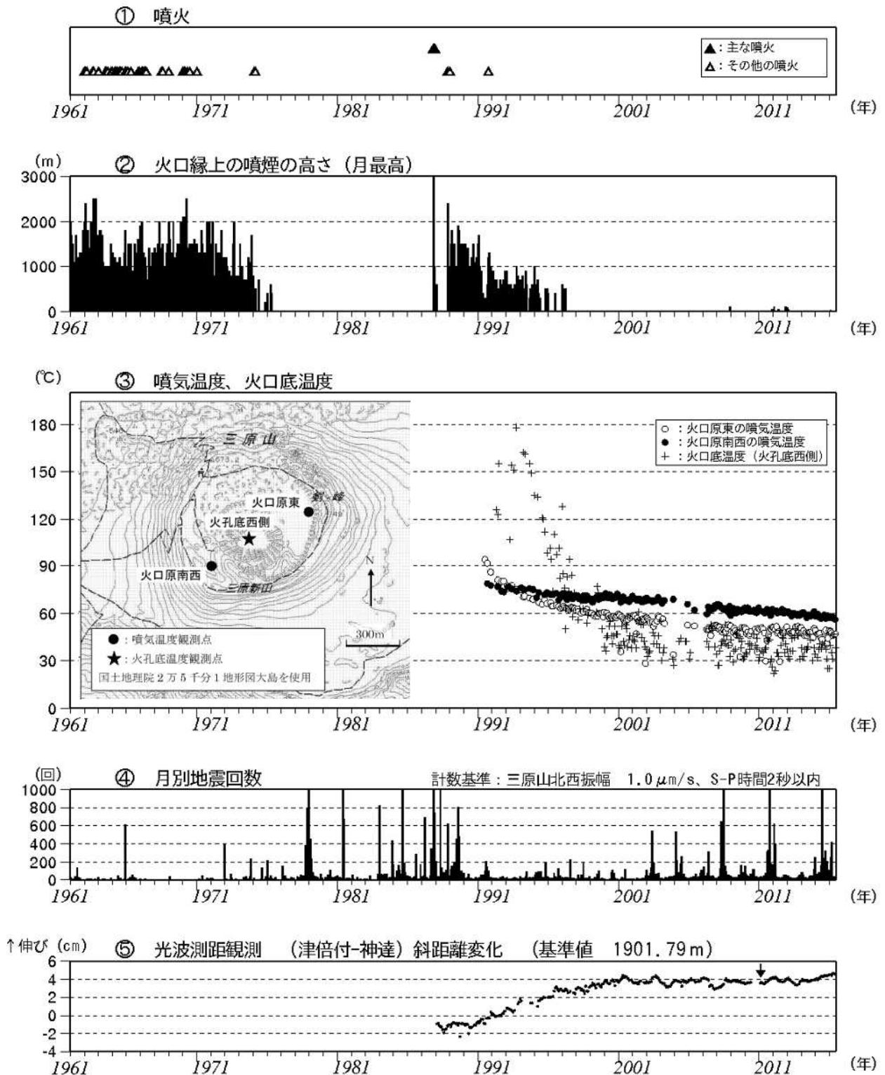
図1 伊豆大島 長期間の火山活動経過図 (1961年1月~2015年6月30日)
