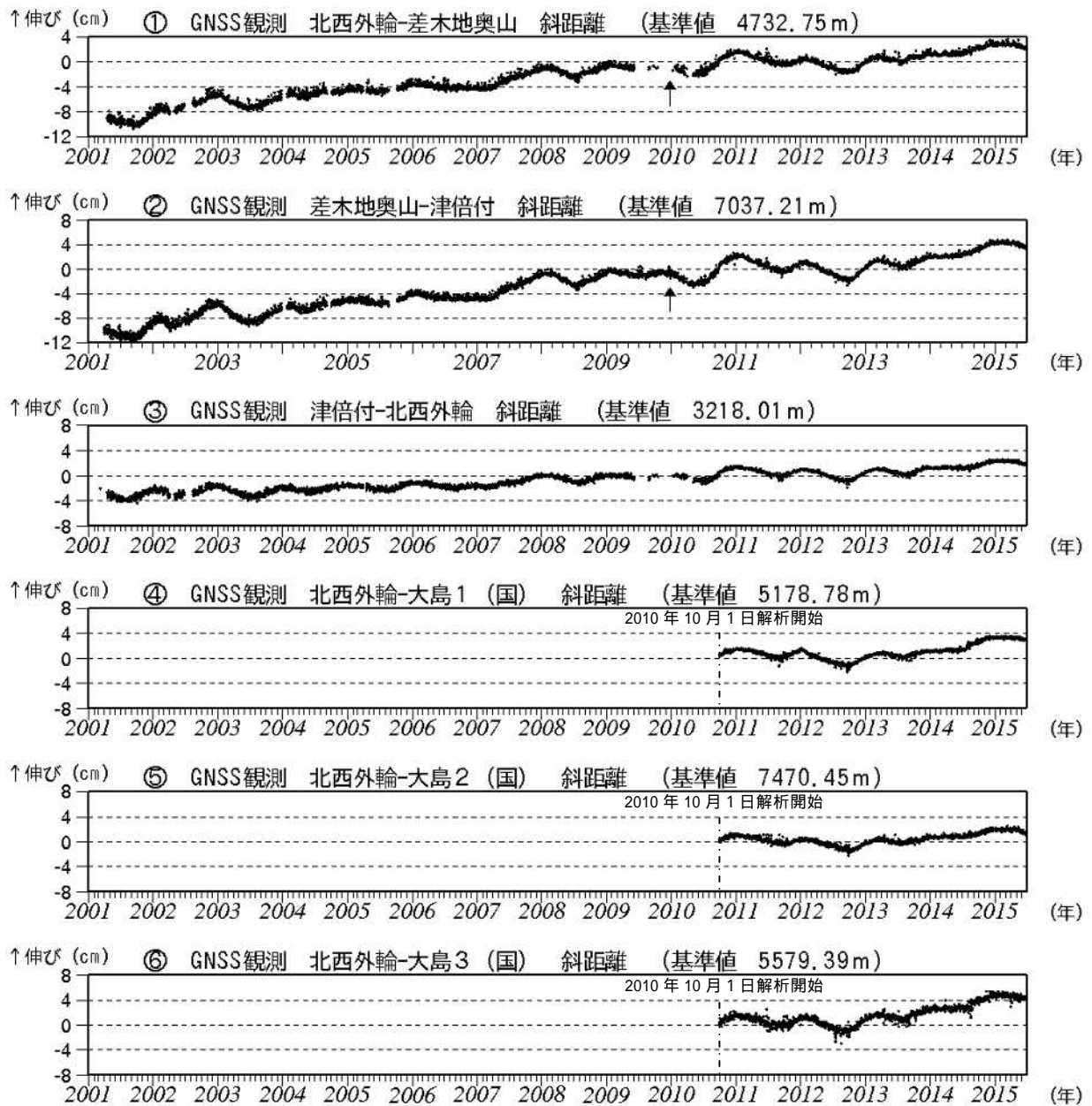
図3 伊豆大島 GNSS連続観測による基線長変化(2001年1月~2015年6月30日)(国): 国土地理院 2010年10月以降のデータについては、電離層の影響を補正する等、解析方法を改良しています。 ~ は図8のGNSS基線 ~ に対応しています。 グラフの空白部分は欠測。 、 の矢印は差木地奥山支柱工事を実施。
