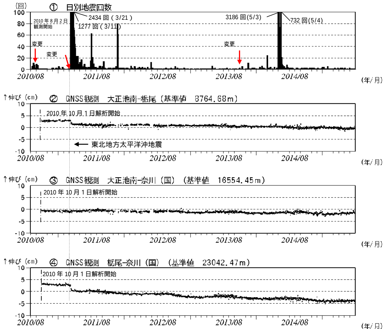
図 2 焼岳 火山活動経過図 (2010 年 8 月 2 日～2015 年 6 月 30 日)
