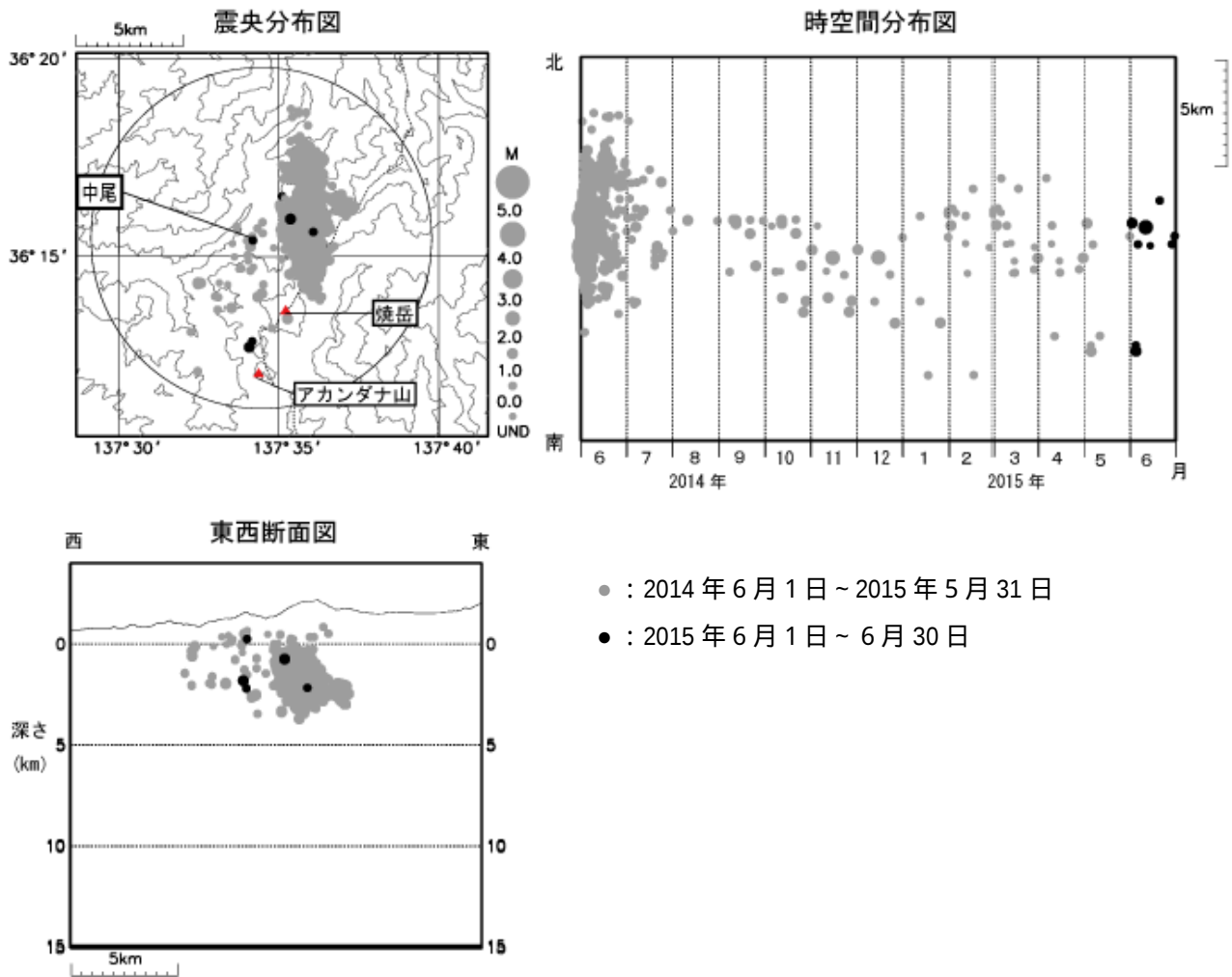
図 3 焼岳 震源分布図（2014 年 6 月 1 日 ~ 2015 年 6 月 30 日）
