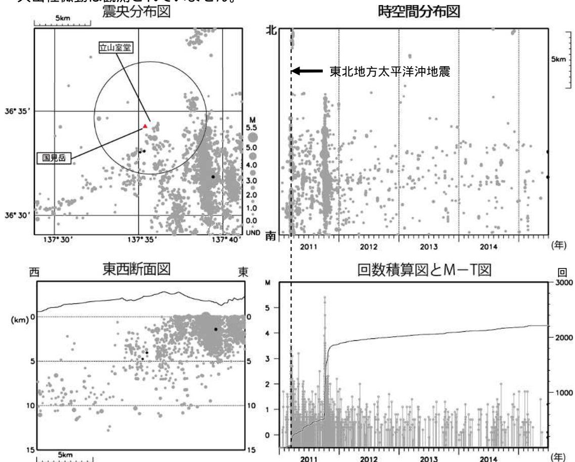
図 1 弥陀ヶ原 広域地震観測網による山体・周辺の地震活動（2011 年 1 月 1 日～2015 年 6 月 30 日）
