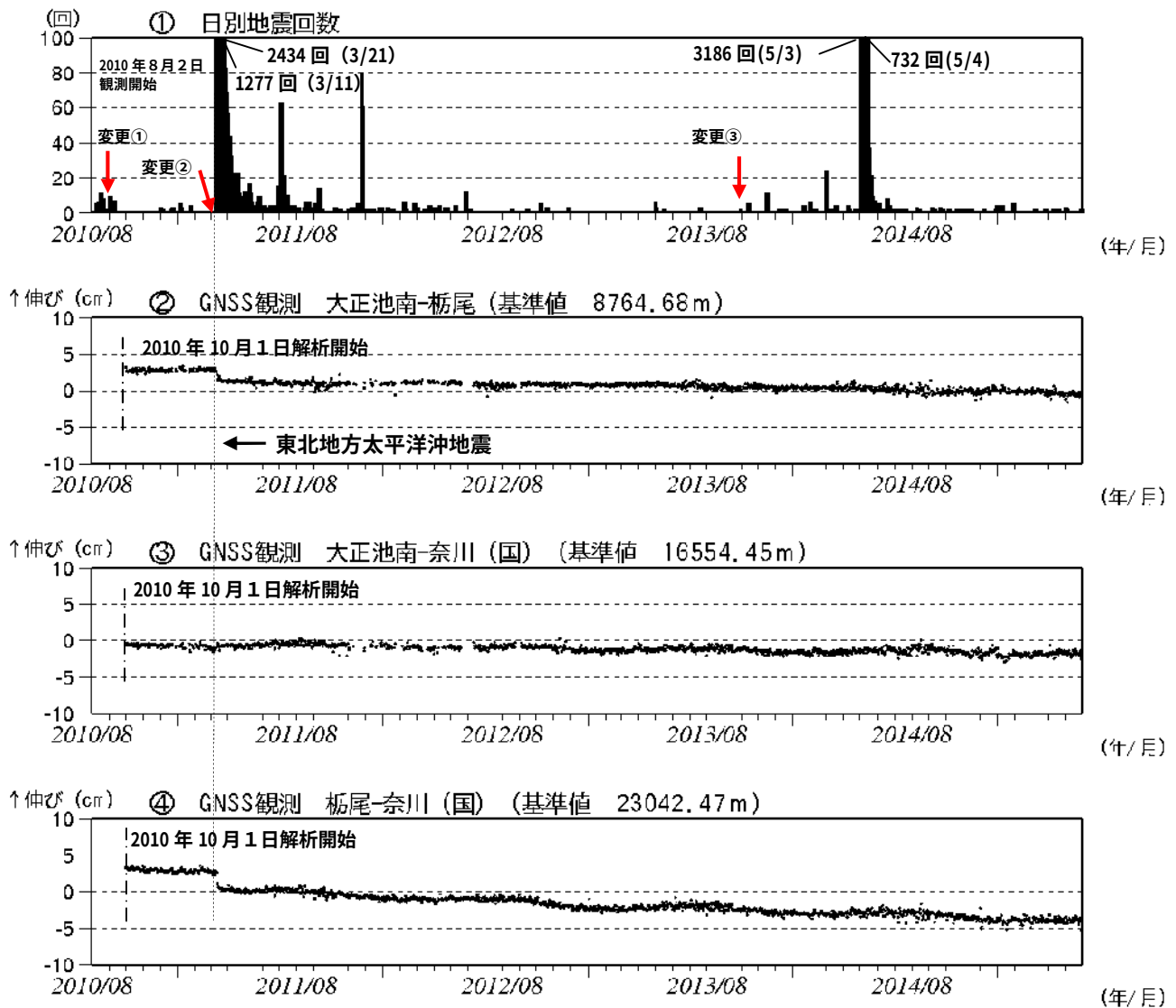
図2 焼岳 火山活動経過図（2010年8月2日～2015年5月31日）
