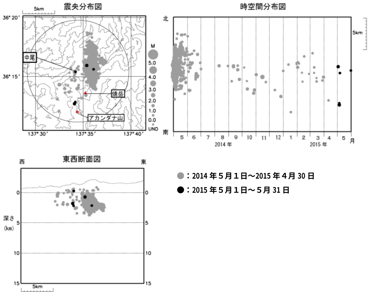
図 3 焼岳 震源分布図（2014 年 5 月 1 日～2015 年 5 月 31 日）
