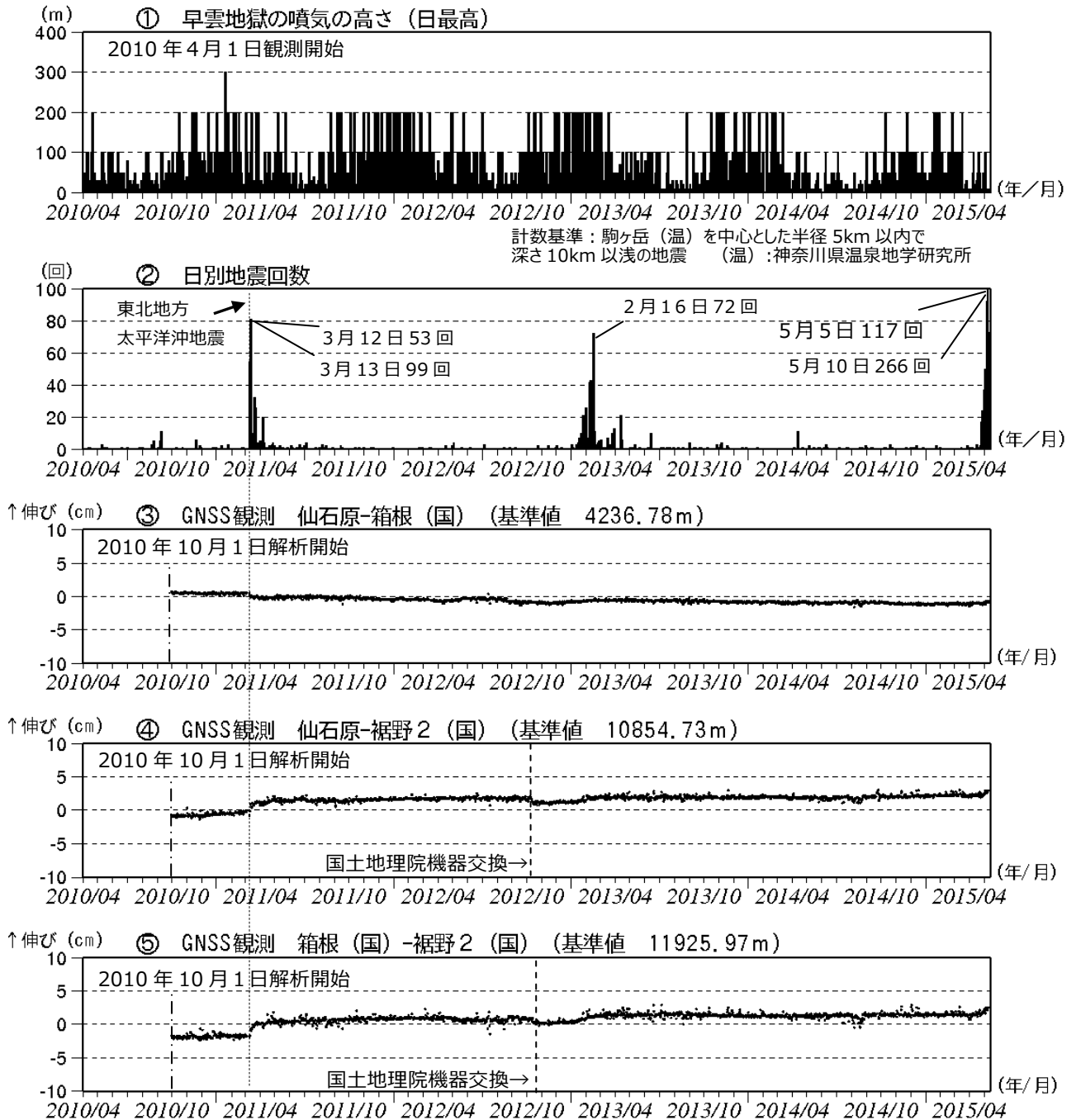
図 4 箱根山 火山活動経過図（2010 年 4 月 1 日～2015 年 5 月 14 日）
