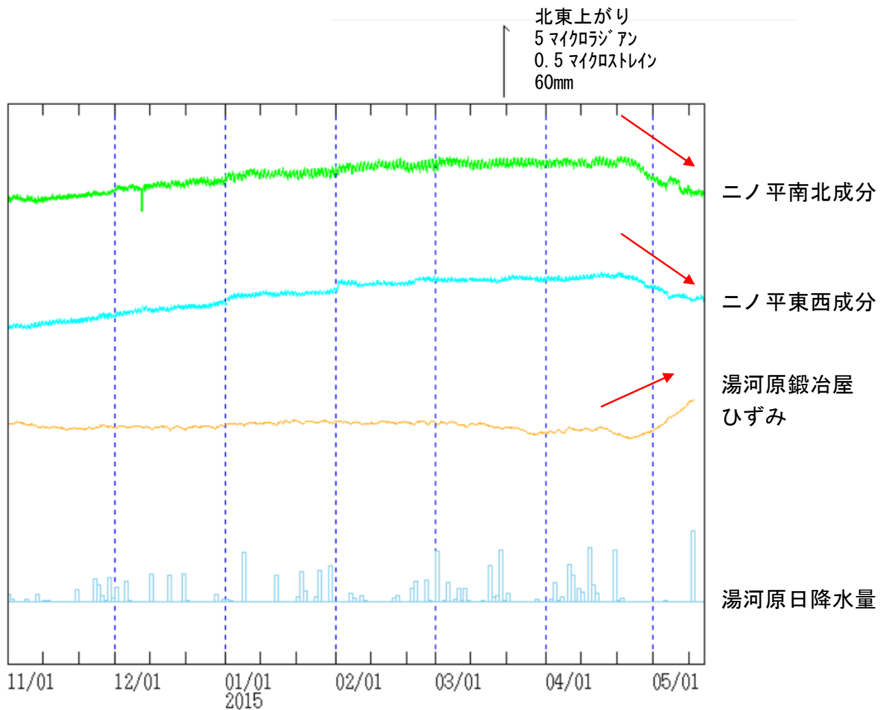
図 6 箱根山 気象庁ニの平観測点傾斜データ及び湯河原鍛冶屋観測点におけるひずみデータの変化 （2015 年 1 月 1 日 00 時～2015 年 5 月 15 日 09 時）
