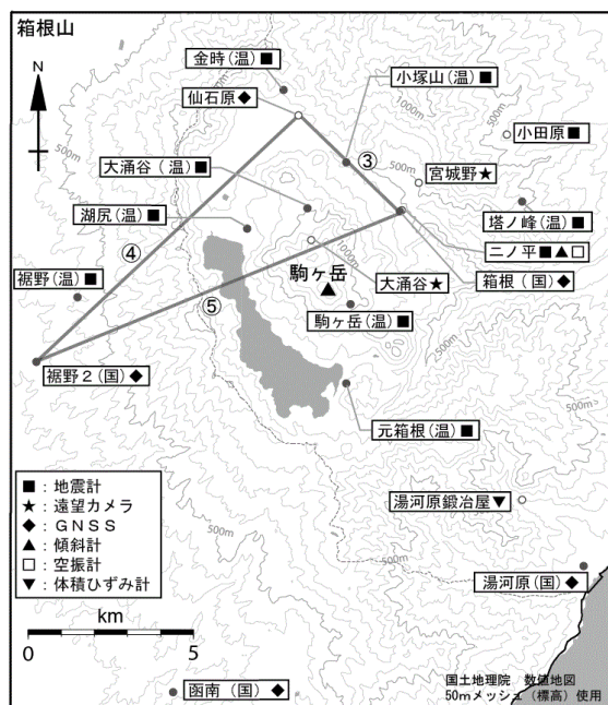
図7 箱根山 観測点配置図
