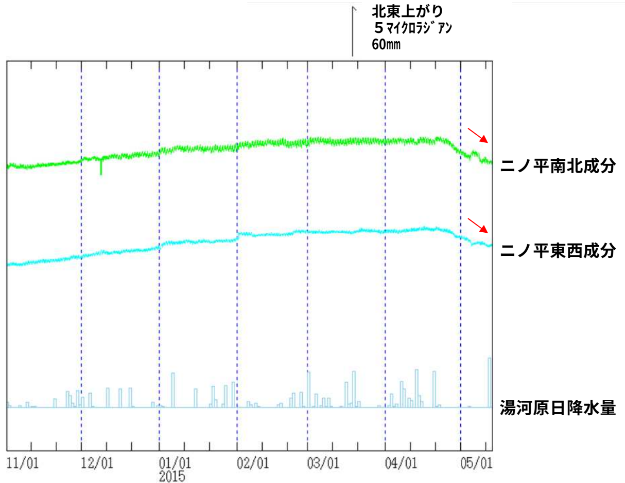
図 4 箱根山 気象庁ニの平観測点傾斜計による変化図 (2014 年 11 月 1 日 00 時～2015 年 5 月 13 日 15 時)
