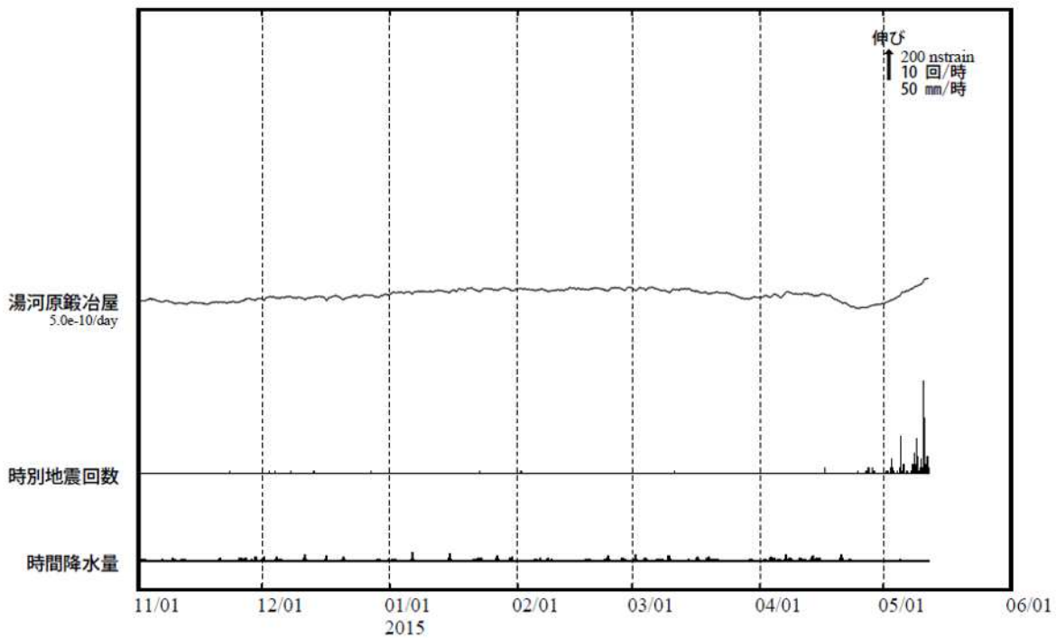
図 5 湯河原鍛冶屋観測点におけるひずみ変化と箱根山地震活動の推移 (2014 年 11 月 1 日～2015 年 5 月 11 日)
