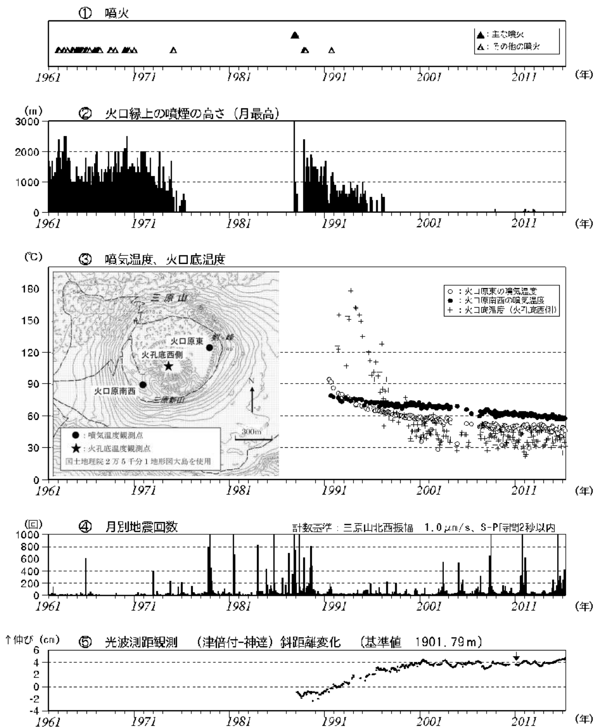
図1 伊豆大島 長期間の火山活動経過図 (1961年1月～2015年4月30日)
