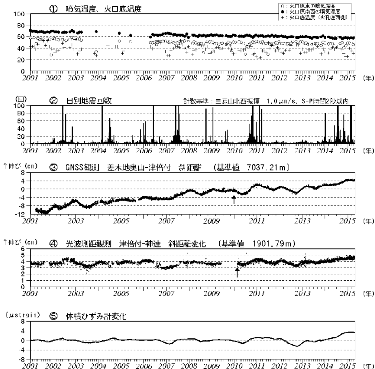
図2 伊豆大島 最近の火山活動経過図（2001年1月～2015年4月30日）
