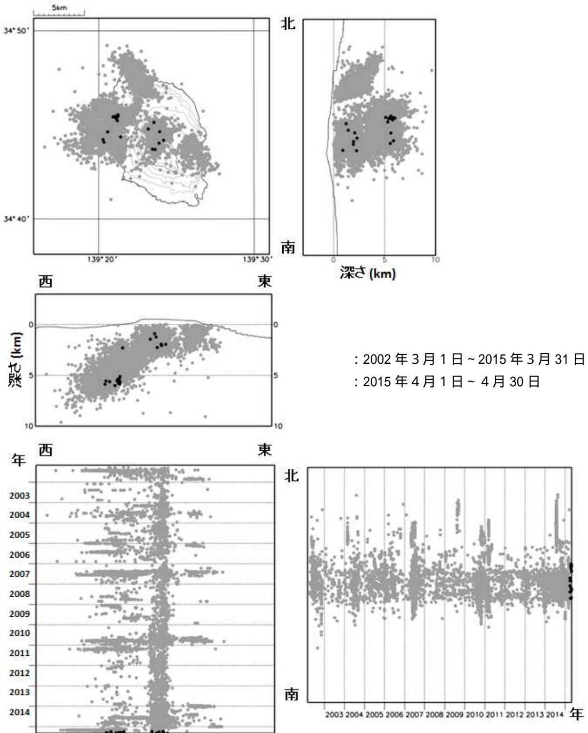
図 4 伊豆大島 震源分布図 (2002 年 3 月 1 日 ~ 2015 年 4 月 30 日)
