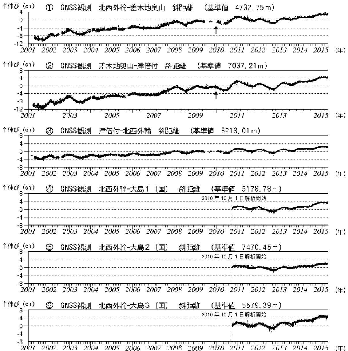
図3 伊豆大島 GNSS連続観測による基線長変化(2001年1月~2015年4月30日)(国): 国土地理院 2010年10月以降のデータについては、電離層の影響を補正する等、解析方法を改良しています。 ~ は図8のGNSS基線 ~ に対応しています。 グラフの空白部分は欠測。 の矢印は差木地奥山支柱工事を実施。
