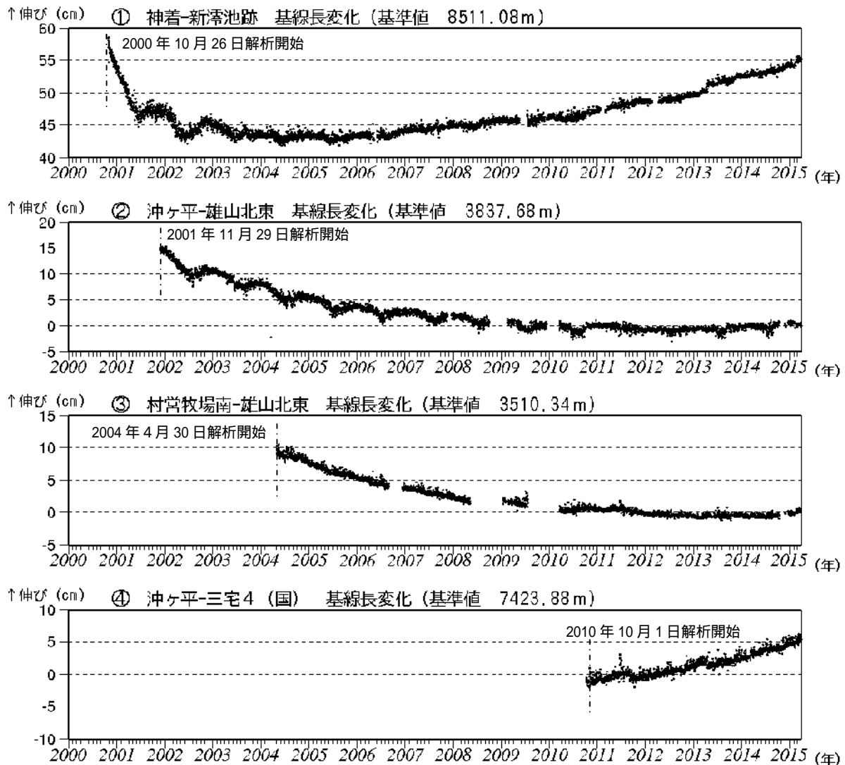
図5 三宅島 GNSS 連続観測結果 (2000年1月1日～2015年3月31日) (国): 国土地理院 ・基線 ~ は図8(観測点配置図)の ~ にそれぞれ対応します。 ・グラフの空白部分は欠測を示します。 ・2010年10月以降のデータについては、電離層の影響を補正する等、解析方法を改良しています。
