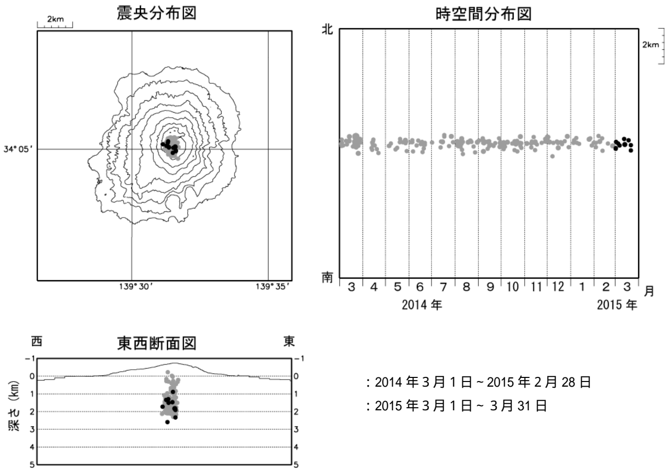
図6 三宅島 震源分布図(2014年3月1日~2015年3月31日)
