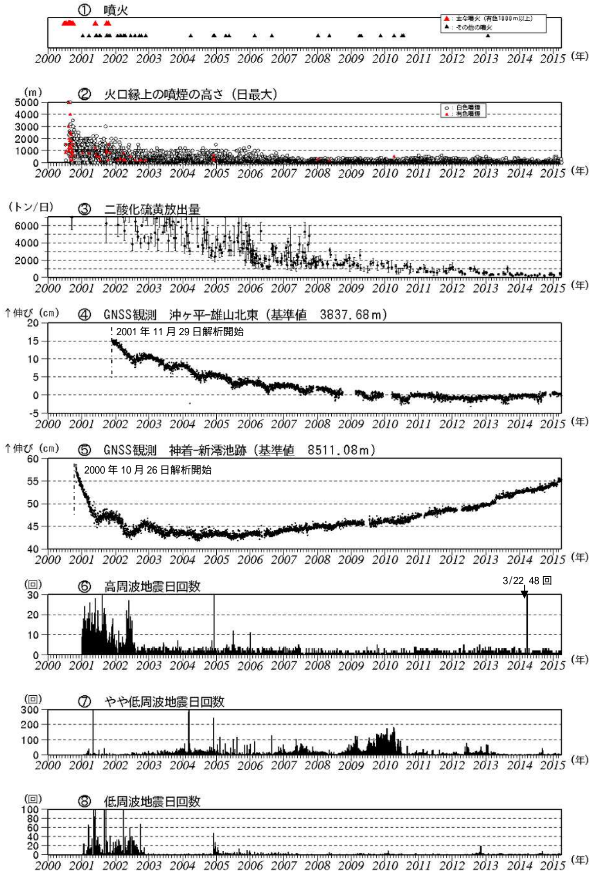
図4 三宅島 火山活動経過図 (2000年1月1日~2015年3月31日)
