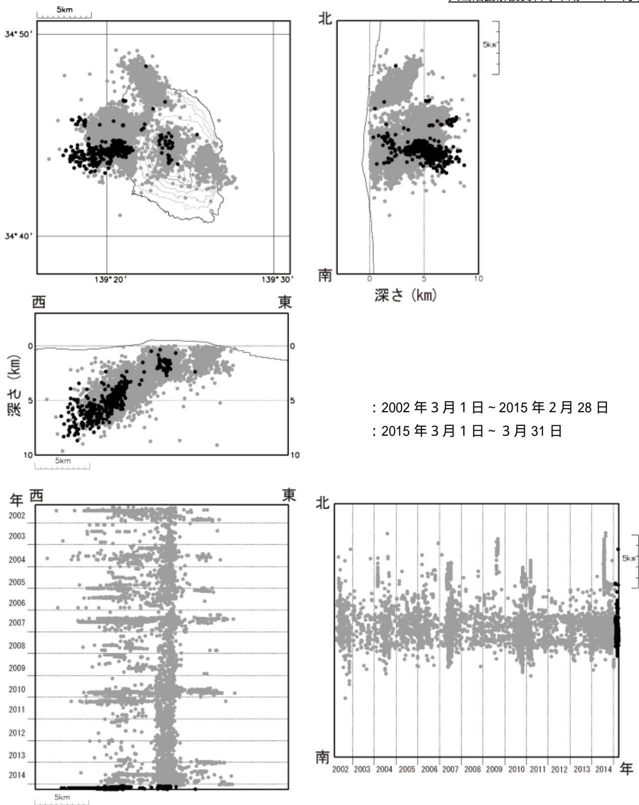
図4 伊豆大島 震源分布図(2002年3月1日~2015年3月31日)
