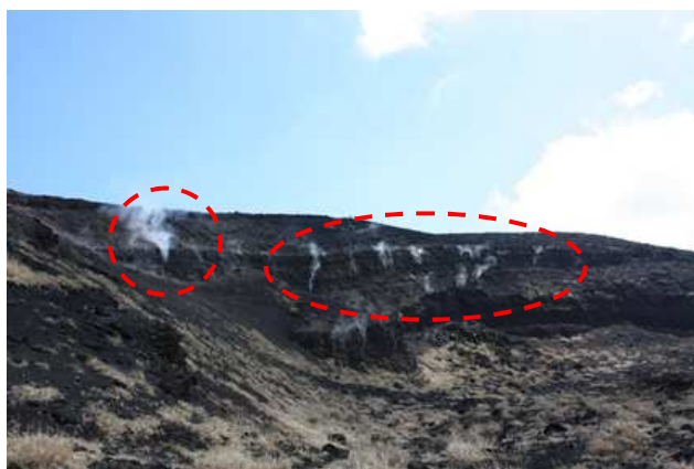
山頂部（3月17日、北西外輪遠望カメラによる） 剣ガ峰付近（3月17日、撮影方向は図7参照） 図5 伊豆大島 三原山山頂部及び山頂火口の状況 破線円内：ごく弱い噴気
