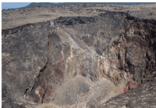
2015年3月17日の火孔内の可視画像
