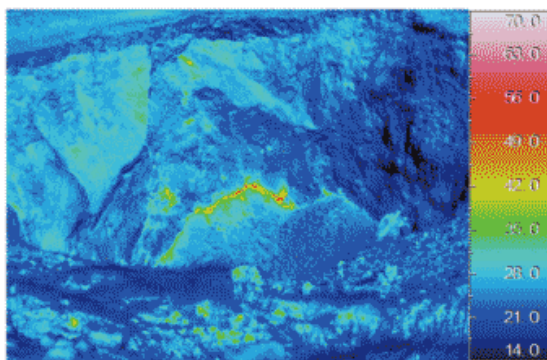
2015年3月17日10時38分撮影
