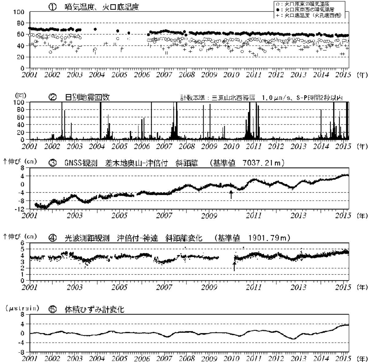
図2 伊豆大島 最近の火山活動経過図（2001年1月～2015年3月31日）
