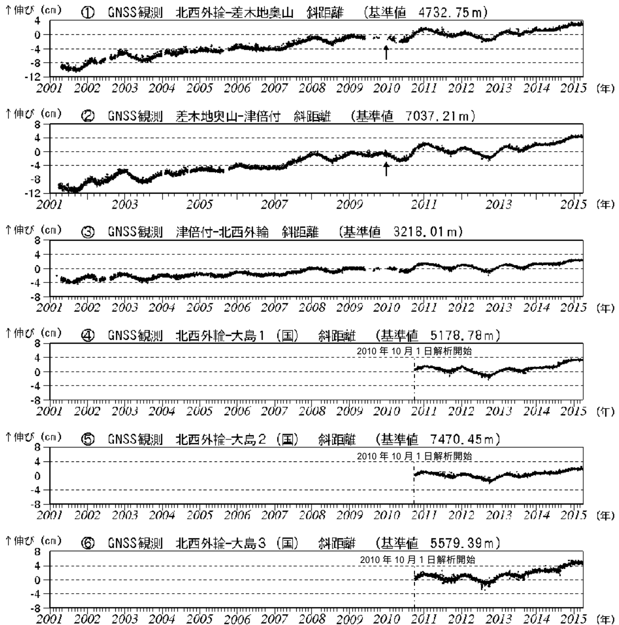
図3 伊豆大島 GNSS連続観測による基線長変化(2001年1月~2015年3月31日)(国): 国土地理院 2010年10月以降のデータについては、電離層の影響を補正する等、解析方法を改良しています。 ~ は図8のGNSS基線 ~ に対応しています。 グラフの空白部分は欠測。 の矢印は差木地奥山支柱工事を実施。
