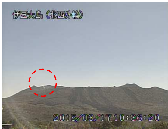
山頂部（3月17日、北西外輪遠望カメラによる） 剣ガ峰付近（3月17日、撮影方向は図7参照） 図5 伊豆大島 三原山山頂部及び山頂火口の状況 破線円内：ごく弱い噴気
