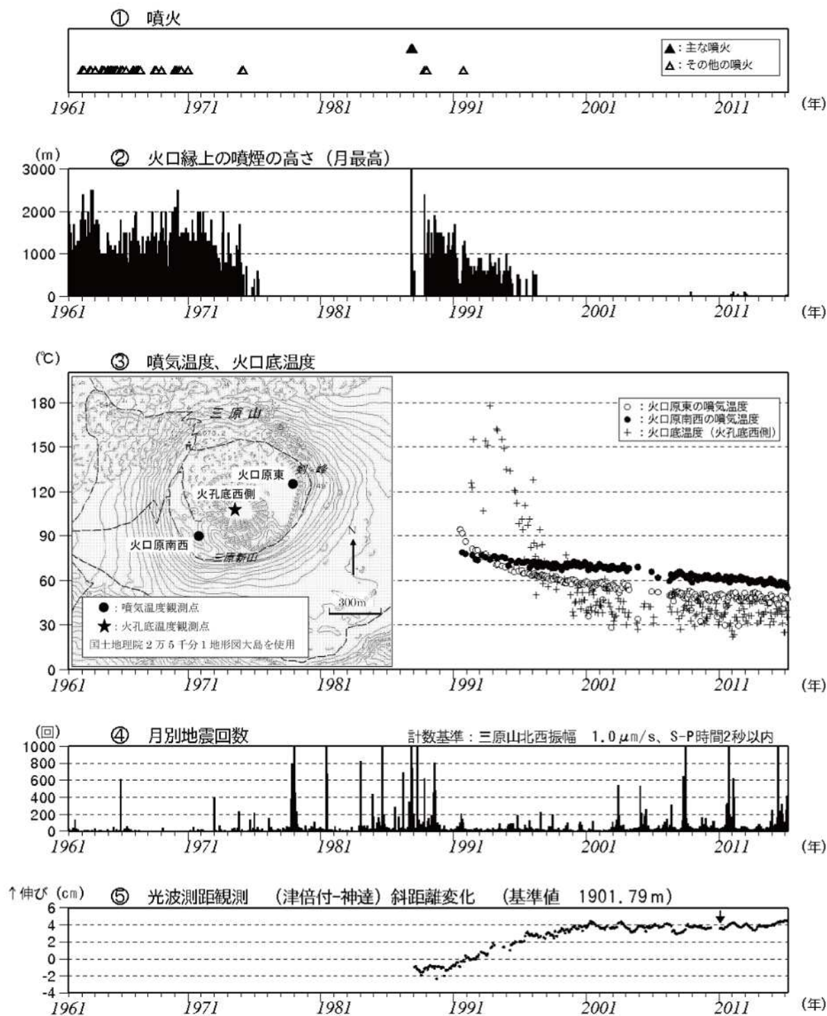
図1 伊豆大島 長期間の火山活動経過図 (1961年1月～2015年3月31日) 1991年12月18日までは火口縁上130m以上、2002年2月28日までは火口縁上300m以上の噴煙の高さを観測していました。 火口底温度 (火口底西側) は赤外放射温度計を用いて離れた場所から測定した値。 噴気温度 (火口原東、火口原南西) はサーミスタ温度計を用いて直接測定した値。 地震回数には伊豆大島周辺海域で発生した地震も一部含まれています。 光波距離計 5) による月平均値 (観測開始は1987年1月)。グラフの空白部分は欠測。矢印は機器更新を示します。
