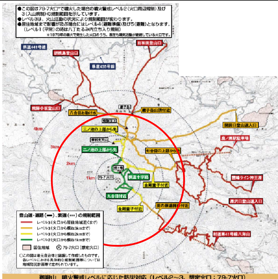
図 1 御嶽山 警戒が必要な範囲 ・赤円が山頂火口から 3 km の範囲
