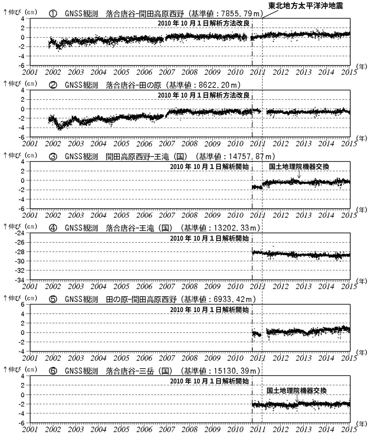
図 4 御嶽山 GNSS 連続観測による基線長の長期変化 (2001 年 1 月 1 日～2015 年 1 月 13 日)
