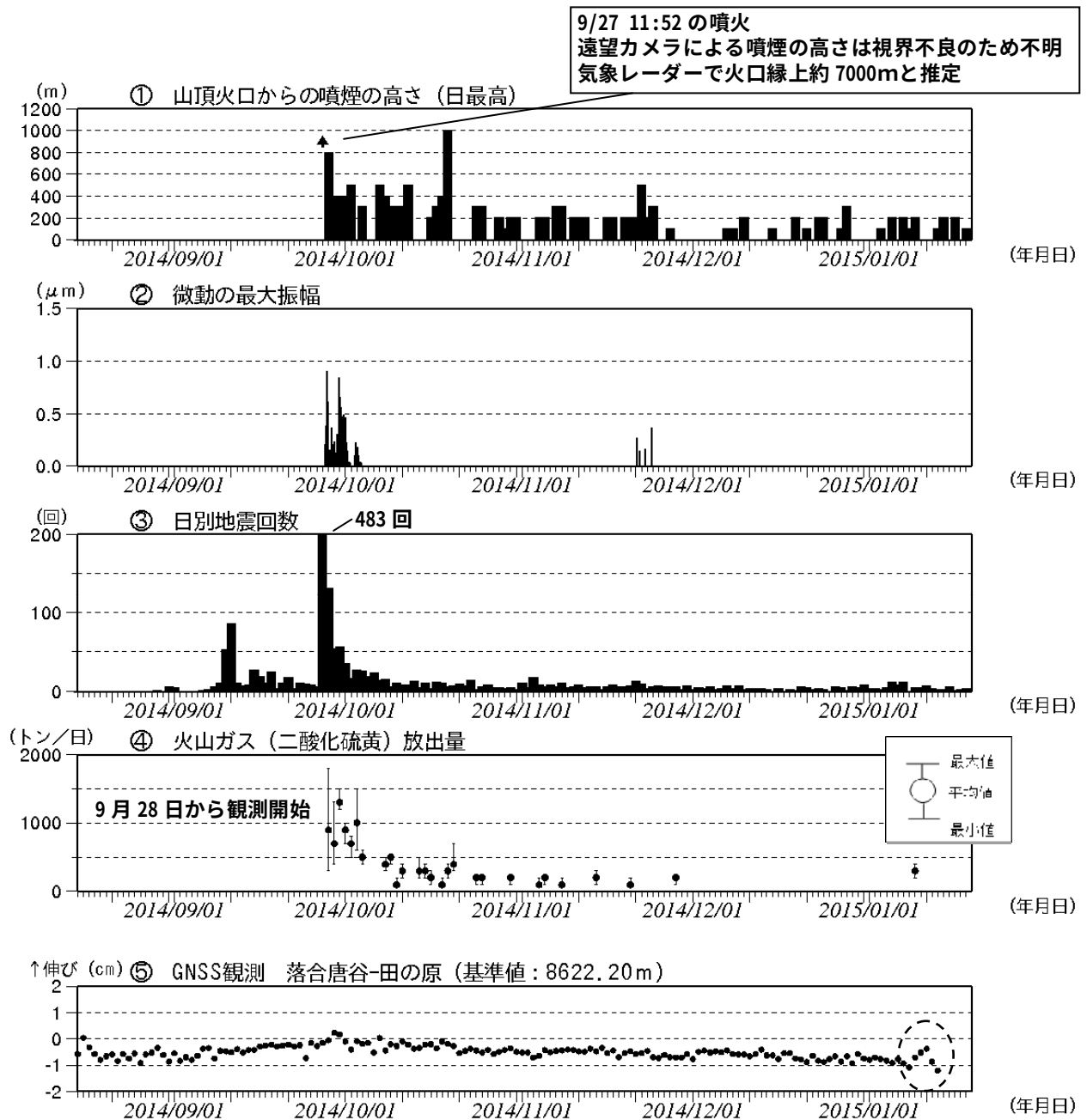
図3 御嶽山 日別活動状況（2014年8月15日～2015年1月18日（速報値含む））
