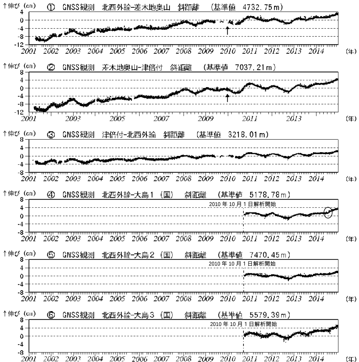
図3 伊豆大島 GNSS 連続観測による基線長変化(2001年1月~2014年12月31日)(国): 国土地理院
