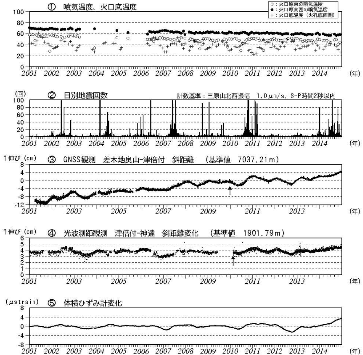
図2 伊豆大島 最近の火山活動経過図（2001年1月～2014年12月31日）
