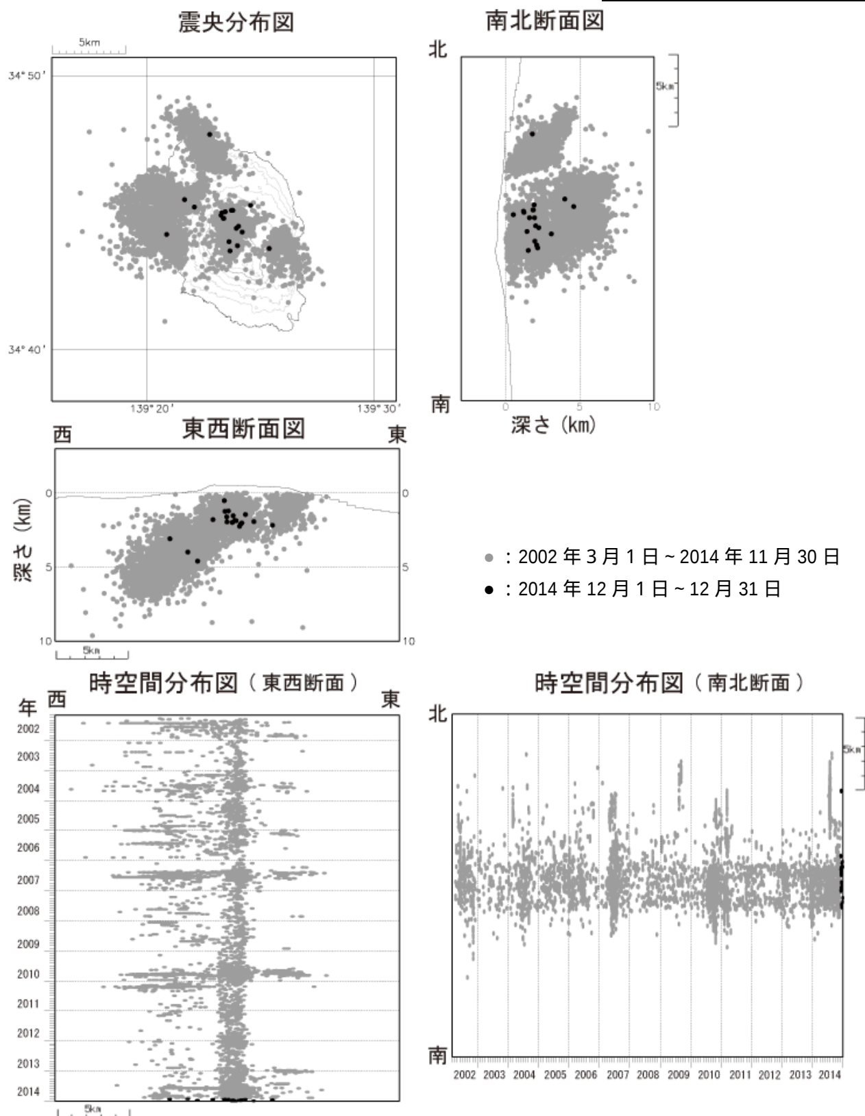
図 4 伊豆大島 震源分布図（2002 年 3 月 1 日 ~ 2014 年 12 月 31 日）
