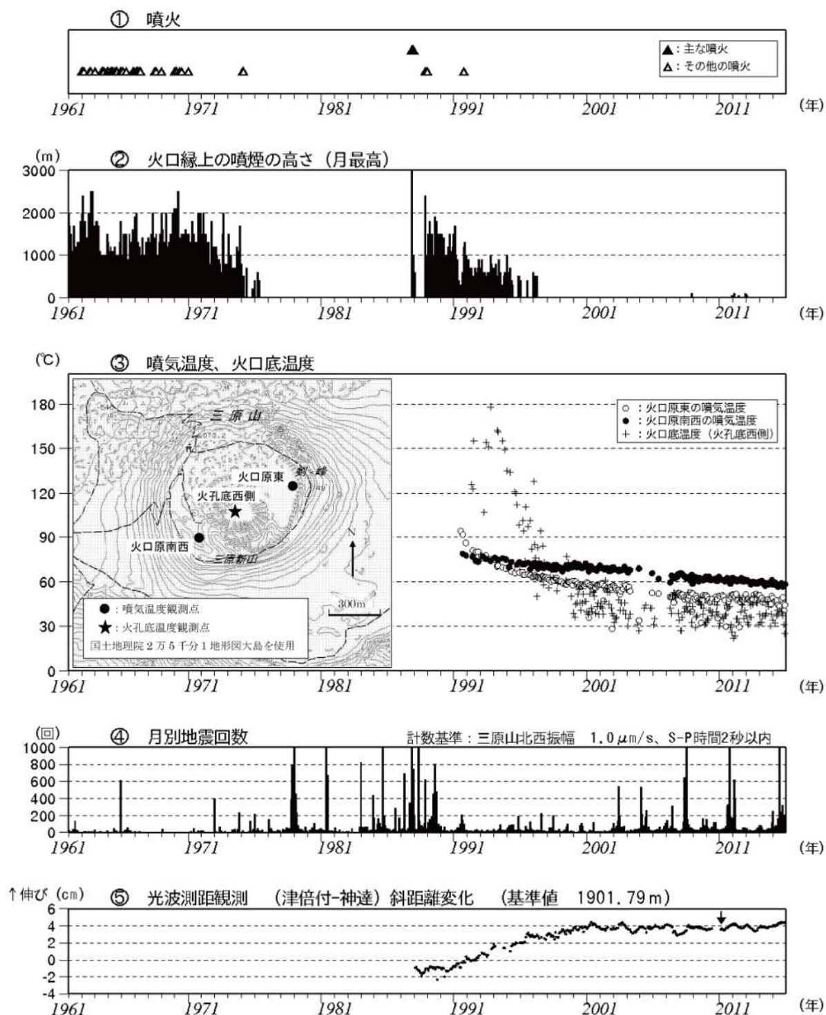
図 1 伊豆大島 長期間の火山活動経過図（1961 年 1 月～2014 年 12 月 31 日）
