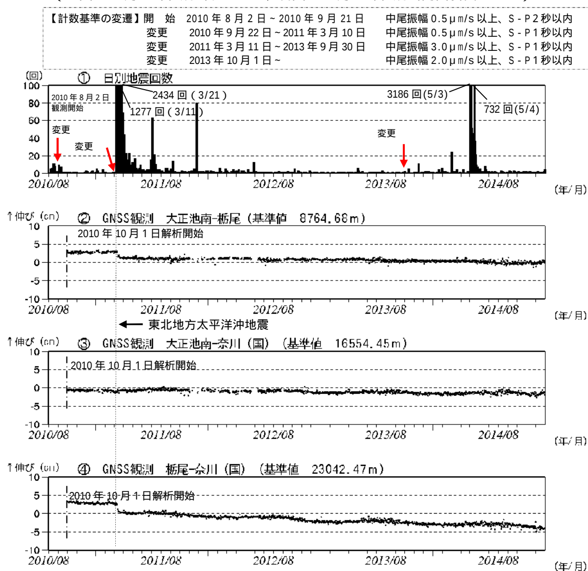
図 3 焼岳 火山活動経過図（2010年8月2日～2014年12月31日）
