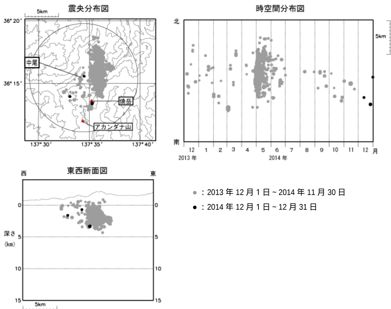
図 4 焼岳 震源分布図（2013 年 12 月 1 日 ~ 2014 年 12 月 31 日）
