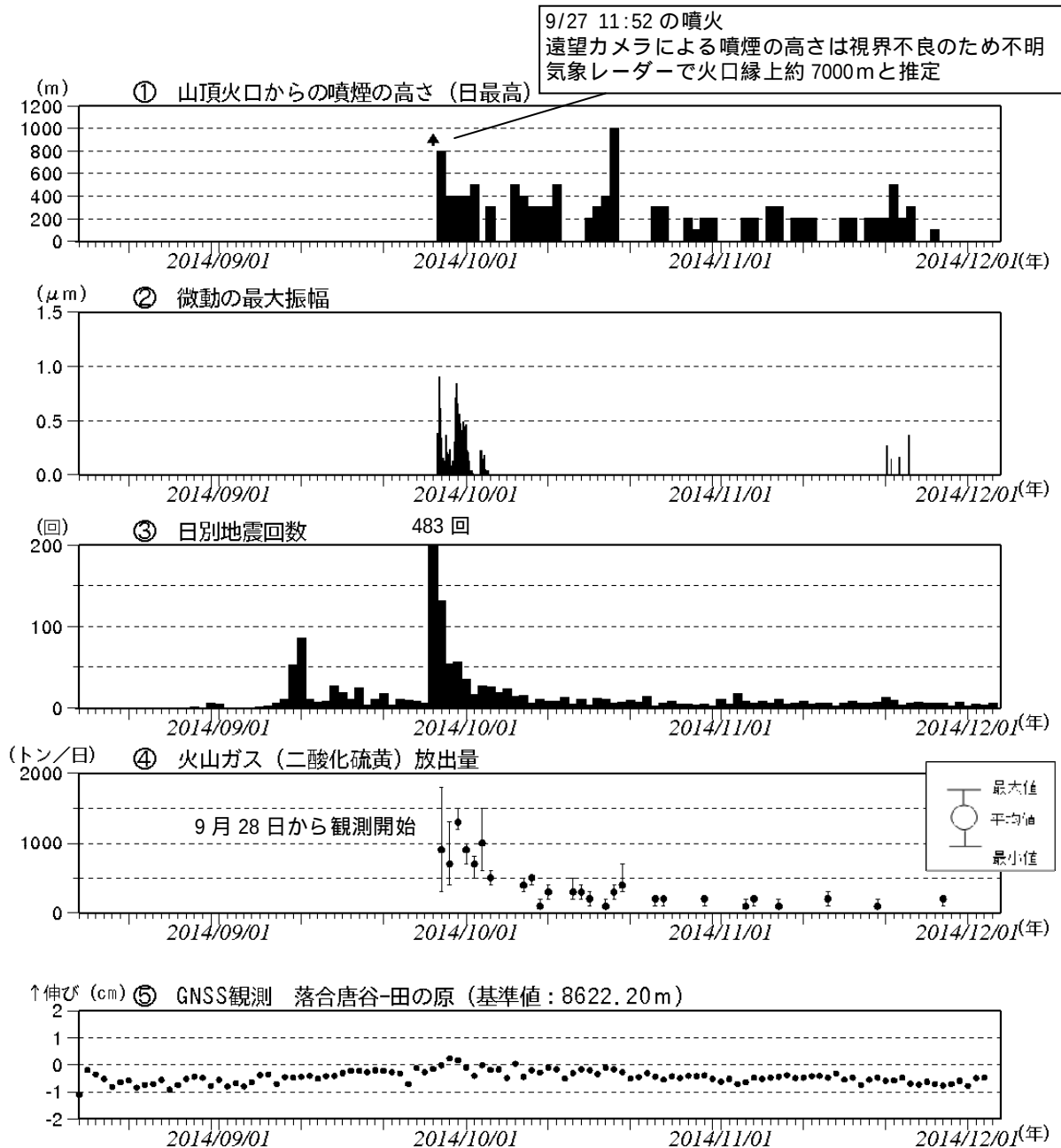
図 1 御嶽山 日別活動状況（2014 年 8 月 15 日～12 月 4 日（速報値含む）） 遠望カメラによる噴煙の高さ 噴煙の高さは日最大値（噴火時以外は定時観測（09 時・15 時）の値）。 矢印は噴火開始を示します。 微動の最大振幅 田の原上観測点（剣ヶ峰南東約 2 km）の上下動の変位振幅。 日別地震回数 計数基準：田の原上振幅 1.5 \mu\text{m/s} 以上、S - P 1 秒以内。 GNSS 観測 図 3 の基線 に対応。
