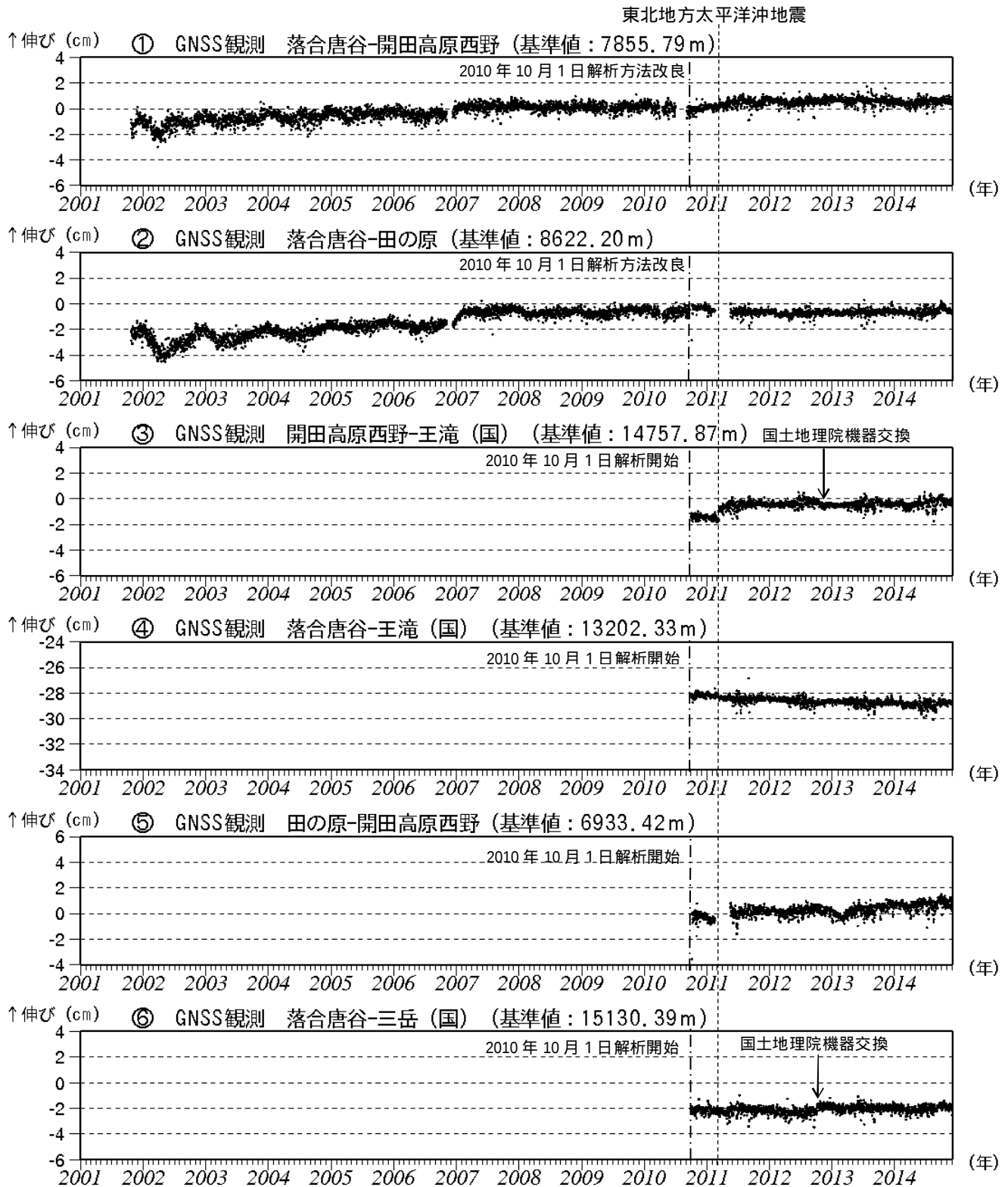
図 2 御嶽山 GNSS 連続観測による基線長の長期変化 (2001 年 1 月 1 日～2014 年 12 月 3 日)
