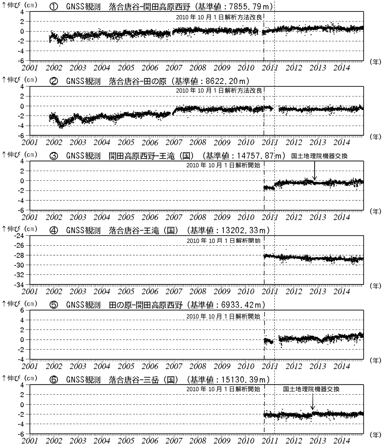
図 3 御嶽山 GNSS 連続観測による基線長の長期変化（2001 年 1 月 1 日～2014 年 11 月 26 日）
