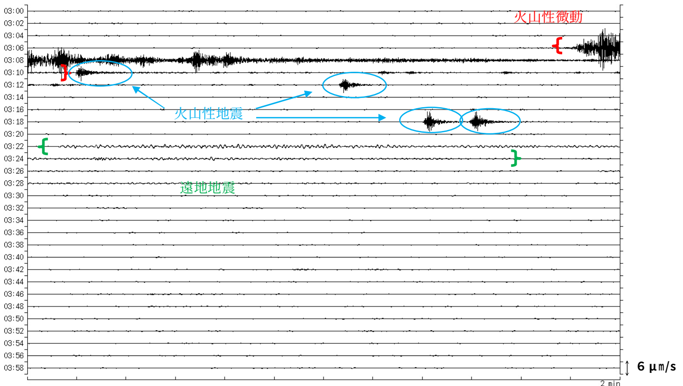
図 2 御嶽山 微動及び地震の発生状況
