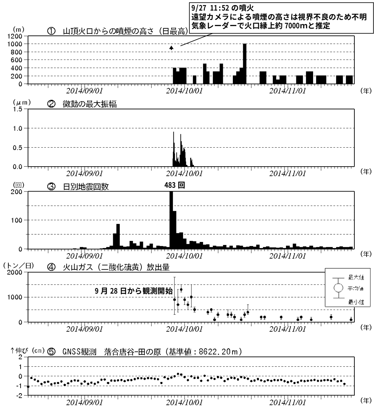
図 3 御嶽山 日別活動状況（2014 年 8 月 15 日～11 月 20 日（速報値含む））
