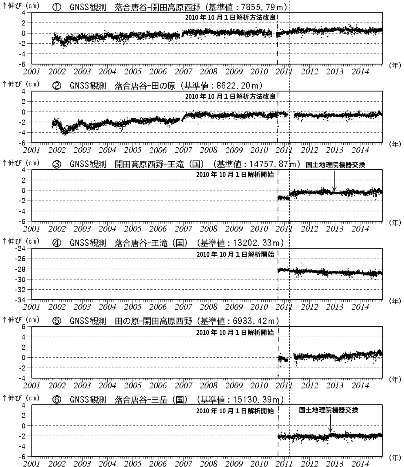
図4 御嶽山 GNSS 連続観測による基線長の長期変化 (2001年1月1日~2014年11月18日)
