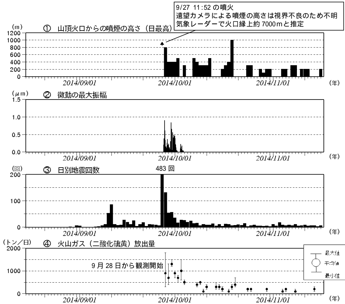
図3 御嶽山 日別活動状況（2014年8月15日～11月16日（速報値含む））
