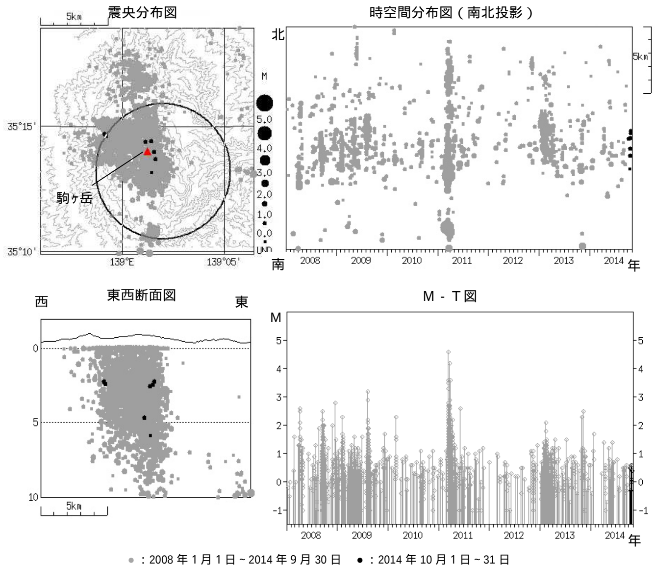
図 5 箱根山 広域地震観測網による山体周辺の震源分布図（2008 年 1 月 1 日 ~ 2014 年 10 月 31 日） M（マグニチュード）は地震の規模を表します。 図中の震源要素は一部暫定値が含まれており、後日変更することがあります。 震源分布図の円は、駒ヶ岳観測点（温）を中心とした半径 5 km の範囲を示しています。
