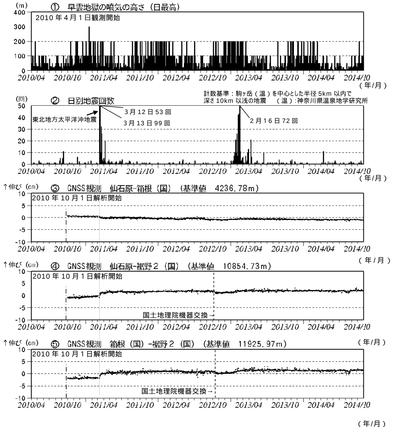
図 4 箱根山 火山活動経過図（2010 年 4 月 1 日～2014 年 10 月 31 日）
