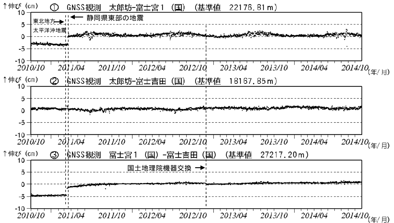
図4 富士山 GNSS 連続観測による基線長変化 (2010 年 10 月 1 日～2014 年 10 月 31 日)
