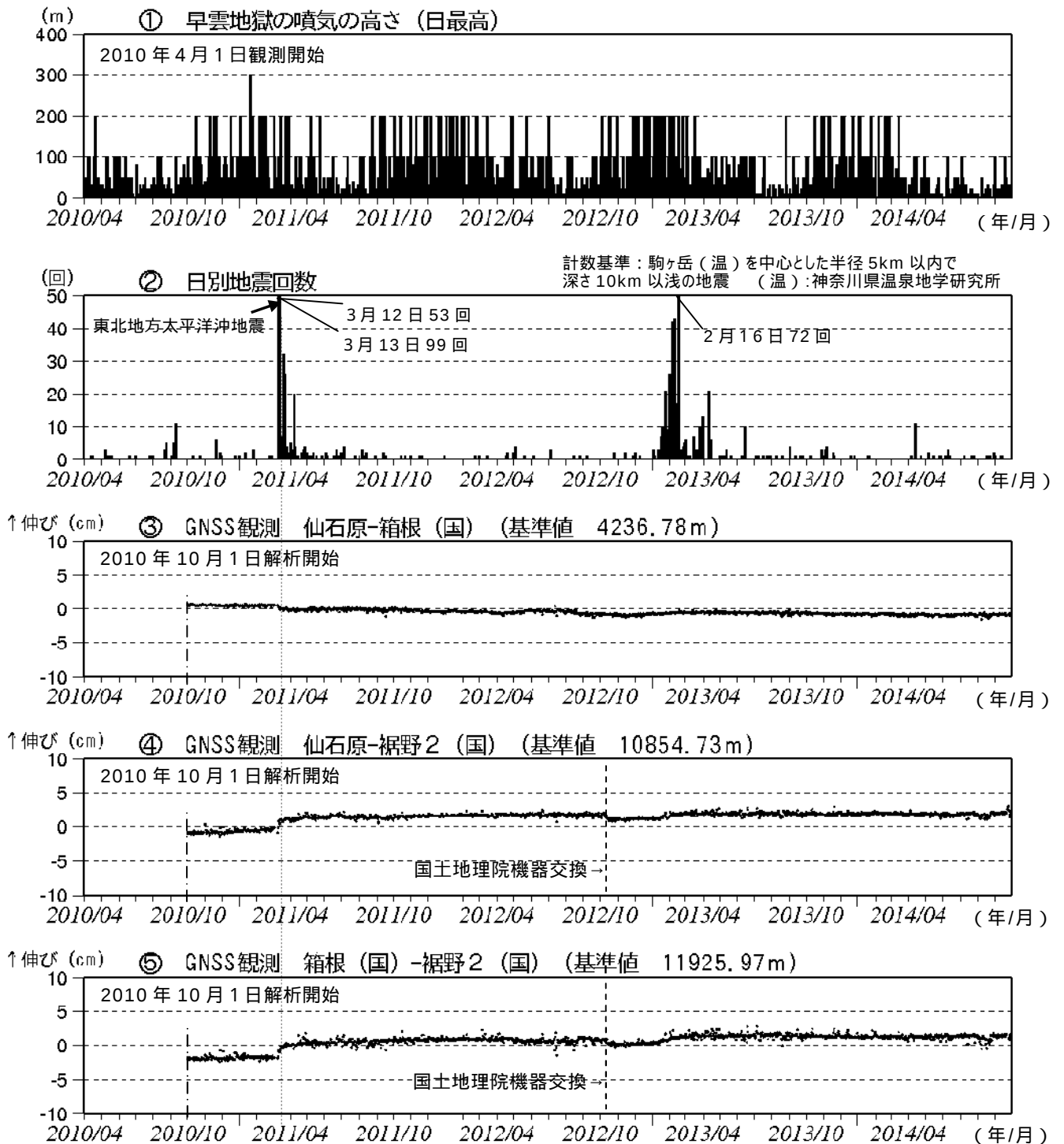
図 4 箱根山 火山活動経過図（2010 年 4 月 1 日～2014 年 9 月 30 日）
