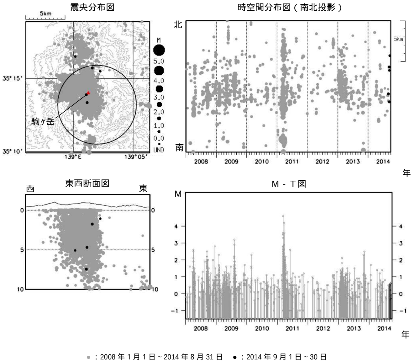
図 5 箱根山 広域地震観測網による山体周辺の震源分布図（2008 年 1 月 1 日 ~ 2014 年 9 月 30 日） M（マグニチュード）は地震の規模を表します。 図中の震源要素は一部暫定値が含まれており、後日変更することがあります。 震源分布図の円は、駒ヶ岳観測点（温）を中心とした半径 5 km の範囲を示しています。
