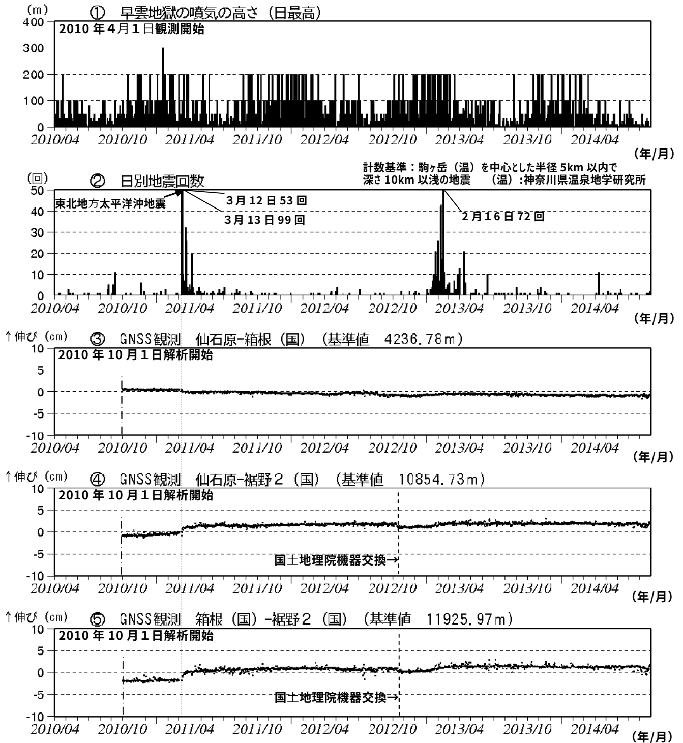
図4 箱根山 火山活動経過図（2010年4月1日～2014年8月31日）
