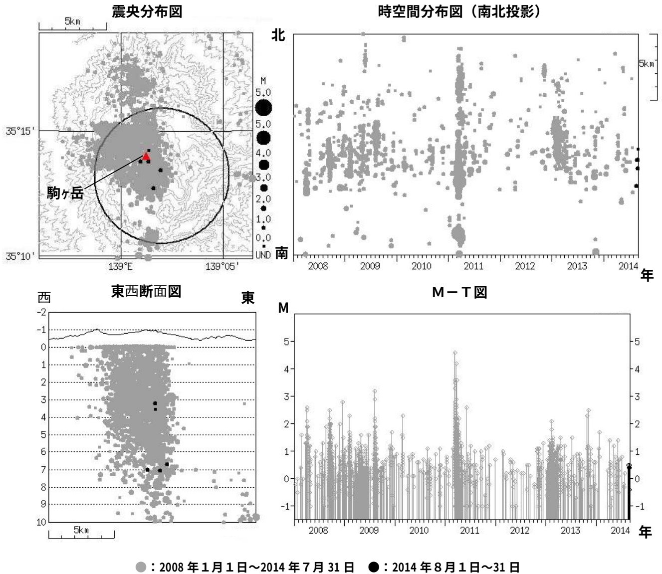
図5 箱根山 広域地震観測網による山体周辺の震源分布図（2008 年 1 月 1 日～2014 年 8 月 31 日） M（マグニチュード）は地震の規模を表します。 図中の震源要素は一部暫定値が含まれており、後日変更することがあります。 震源分布図の円は、駒ヶ岳観測点（温）を中心とした半径 5 km の範囲を示しています。
