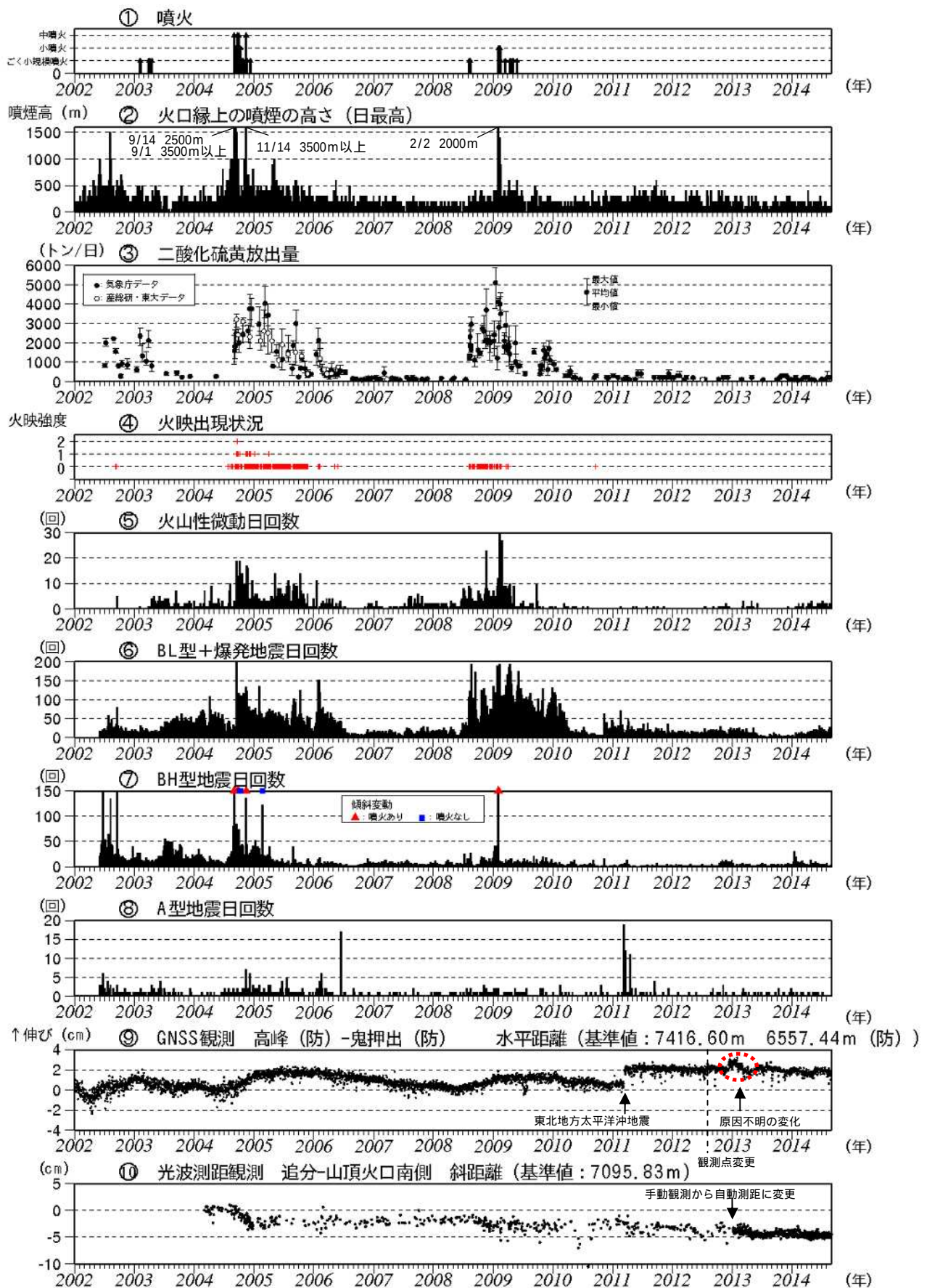
図5 浅間山 火山活動経過図 (2002年1月1日～2014年8月31日)
