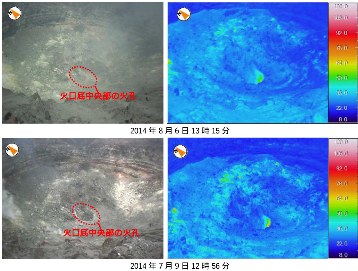
図 3 浅間山 山頂火口内の状況及び地表面温度分布 1)
