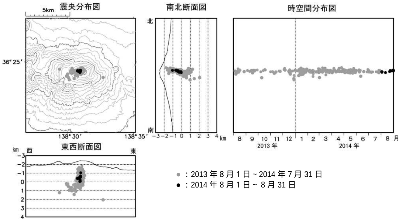
図 6 浅間山 震源分布図（2013 年 8 月 1 日～2014 年 8 月 31 日）
