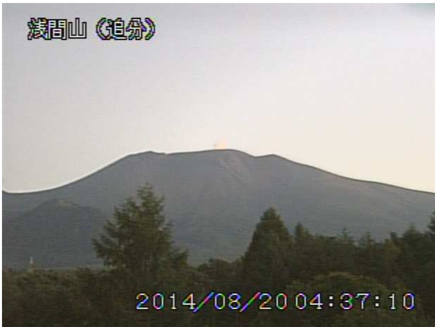
図2 浅間山 山頂部の噴煙の状況 (8月20日、追分遠望カメラによる)
