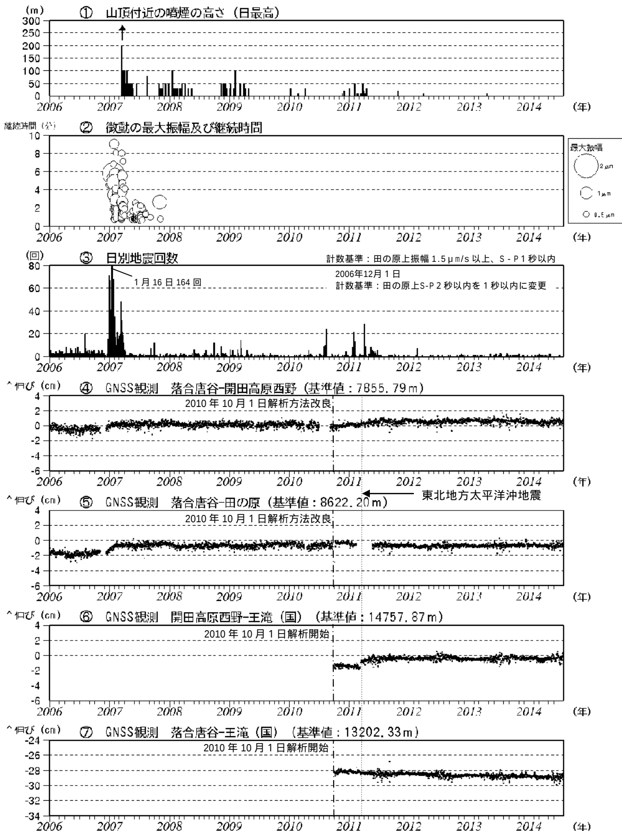
図3 御嶽山 火山活動経過図(2006年1月1日~2014年7月31日)
