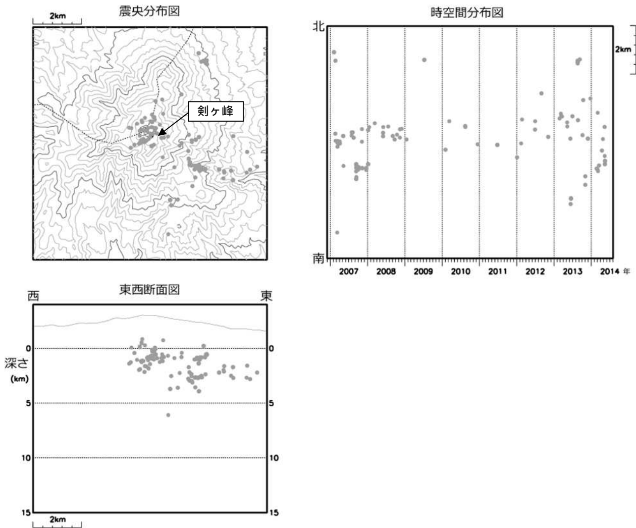
図 4 御嶽山 震源分布図（2006 年 12 月 1 日～2014 年 7 月 31 日） ●：2006 年 12 月 1 日～2014 年 6 月 30 日 ●：2014 年 7 月 1 日～7 月 31 日
