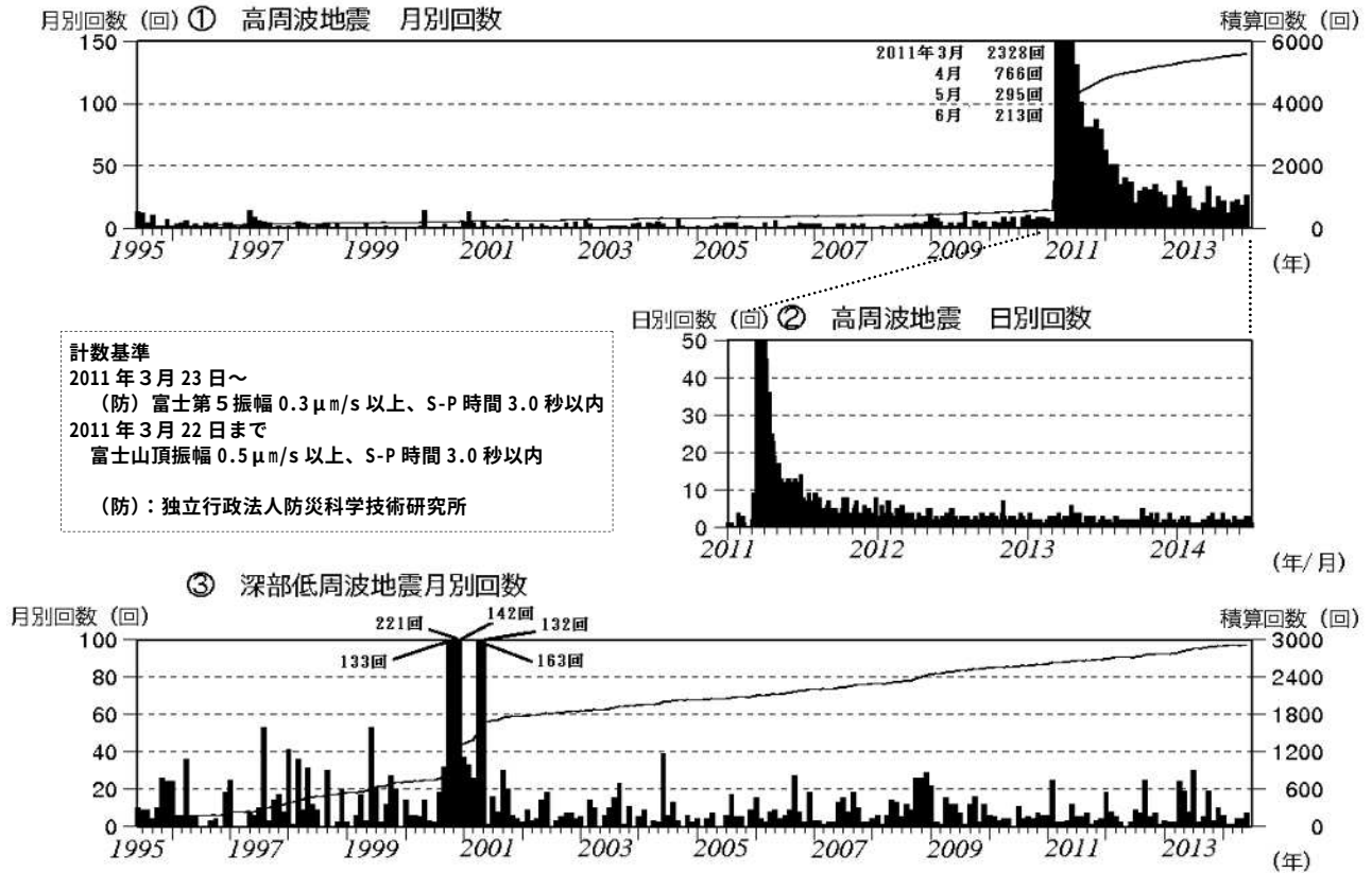
図2 富士山 月別及び日別地震回数（1995年6月1日～2014年6月30日）
