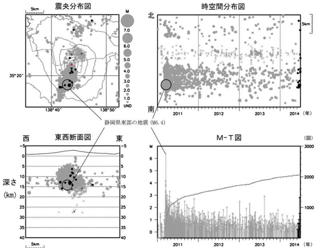
図3 富士山 広域地震観測網による山体・周辺の地震活動（2011年1月1日～2014年6月30日）
