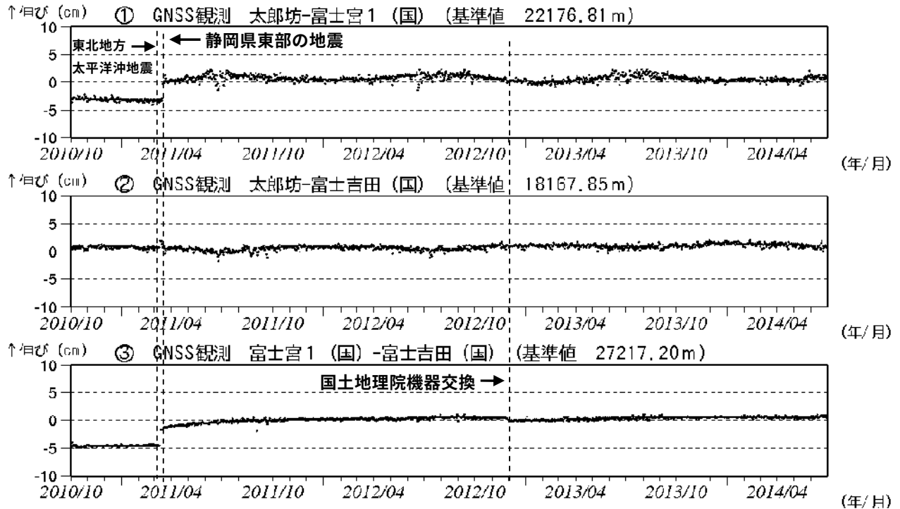
図4 富士山 GNSS 連続観測による基線長変化（2010 年 10 月 1 日～2014 年 6 月 30 日）
