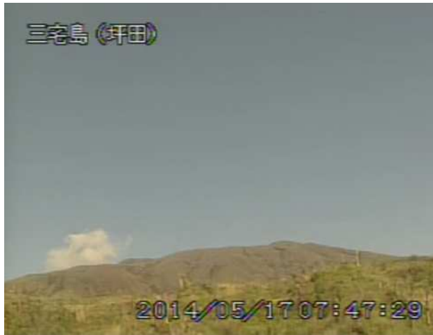
図1 三宅島 山頂火口からの噴煙の状況 （5月17日、坪田遠望カメラによる）
