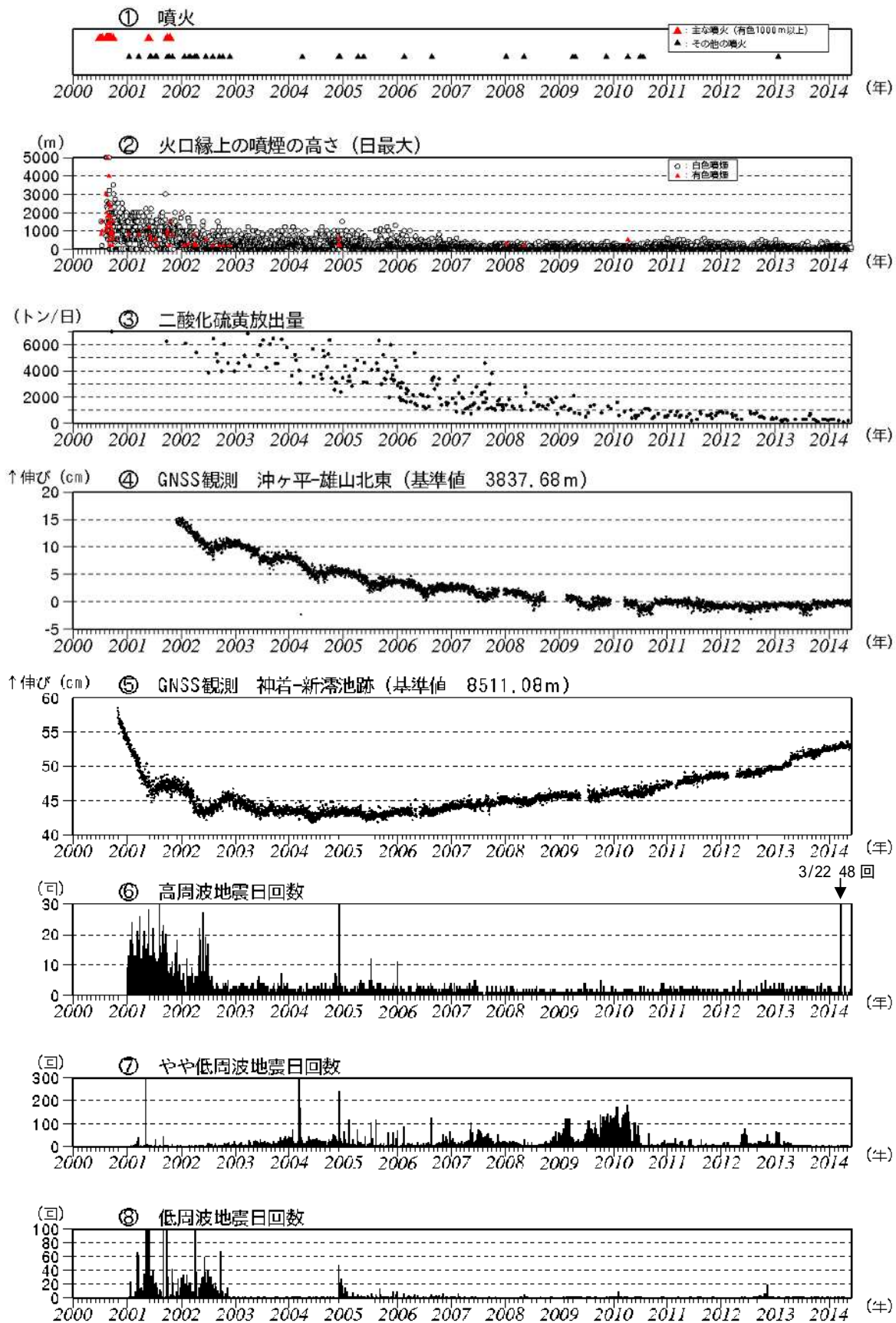
図4 三宅島 最近の火山活動の経過図 (2000年1月~2014年5月)
