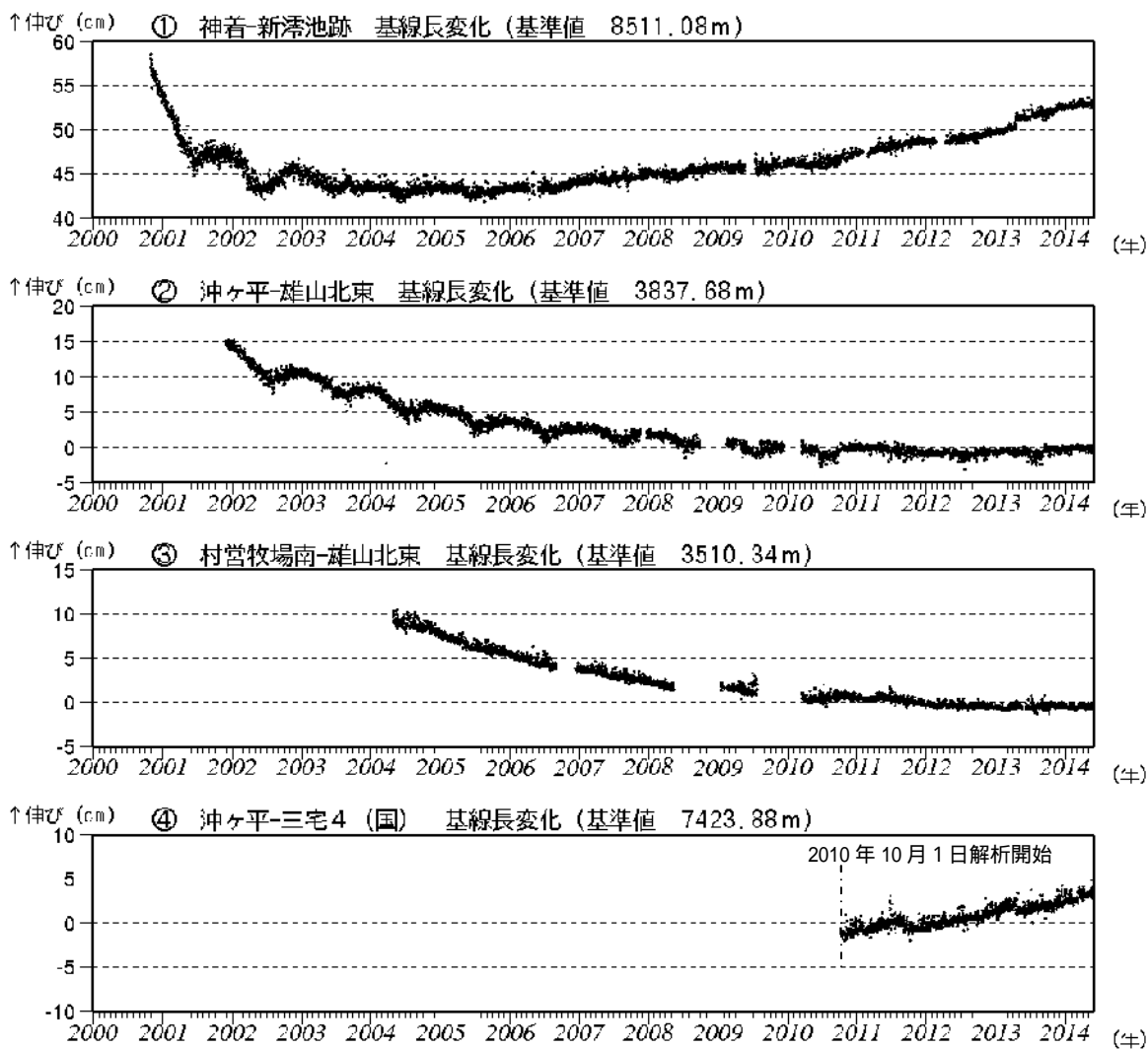
図 5 三宅島 GNSS 連続観測結果(2000 年 1 月~2014 年 5 月) (国): 国土地理院 ・基線 ~ は図 8 (観測点配置図)の ~ にそれぞれ対応します。 ・グラフの空白部分は欠測を示します。 ・2010 年 10 月以降のデータについては、電離層の影響を補正する等、解析方法を改良しています。
