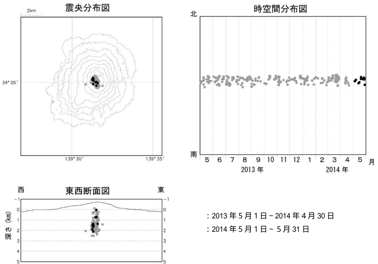
図6 三宅島 震源分布図(2013年5月1日～2014年5月31日)
