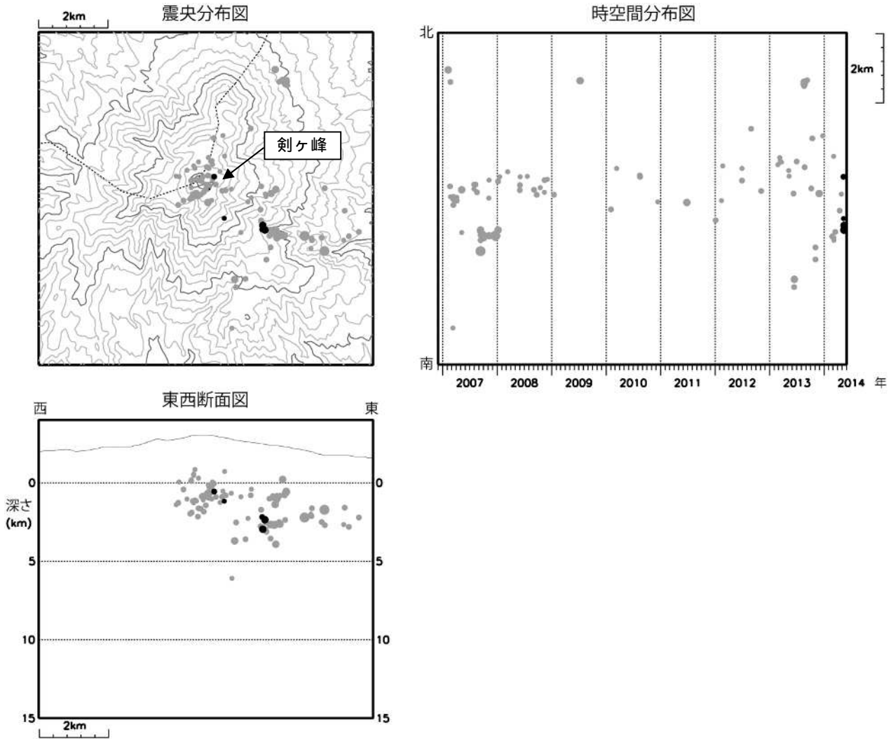
図4 御嶽山 震源分布図(2006年12月1日~2014年5月31日) : 2006年12月1日~2014年4月30日 : 2014年5月1日~5月31日
