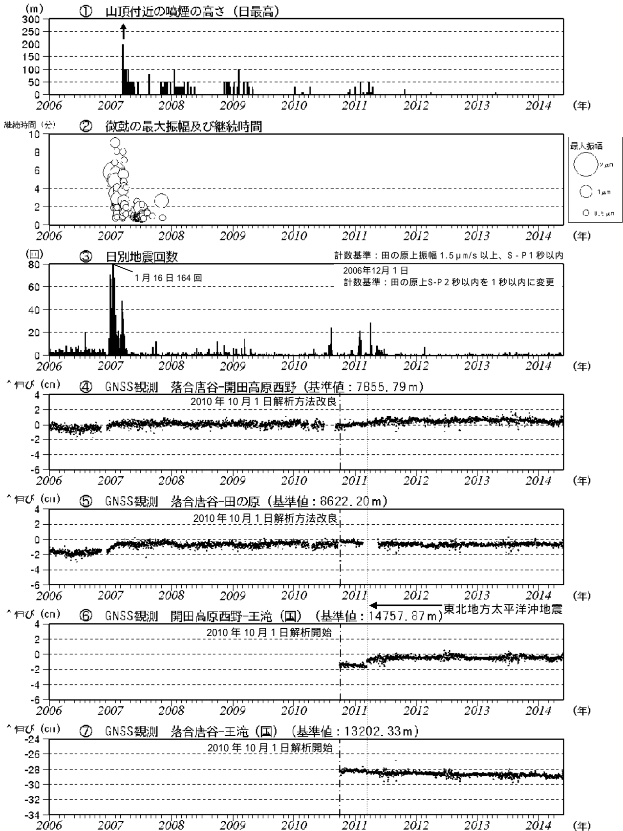
図3 御嶽山 最近の火山活動経過図(2006年1月1日~2014年5月31日)
