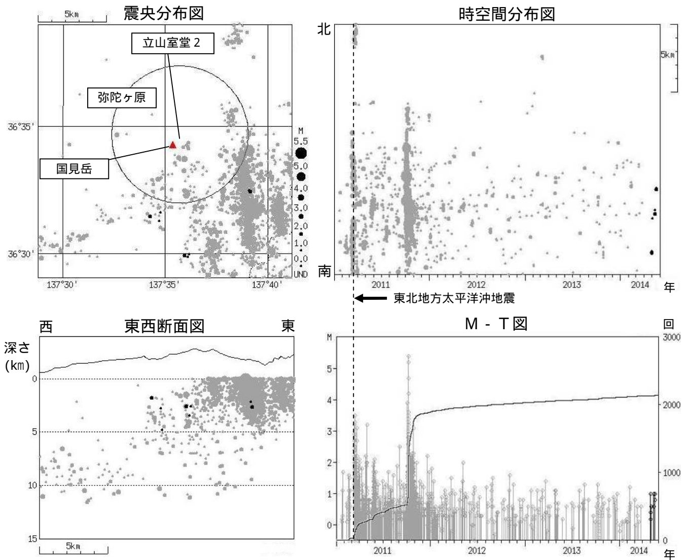
図 2 弥陀ヶ原 広域地震観測網による山体・周辺の地震活動（2011 年 1 月 1 日～2014 年 5 月 31 日） ●：2011 年 1 月 1 日～2014 年 4 月 30 日 ●：2014 年 5 月 1 日～5 月 31 日 ・ 緑色の点線の円は、立山室堂に設置した地震計（立山室堂 2）で S-P 時間 1 秒以内となるおよその範囲を示します。 ・ M（マグニチュード）は地震の規模を表します。 ・ 図中の震源要素は一部暫定値が含まれており、後日変更することがあります。 ・ 弥陀ヶ原近傍の地震活動は、低調な状況で経過しました。
