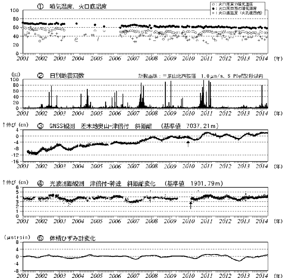
図 2 伊豆大島 最近の火山活動経過図（2001 年 1 月～2014 年 4 月 30 日）
