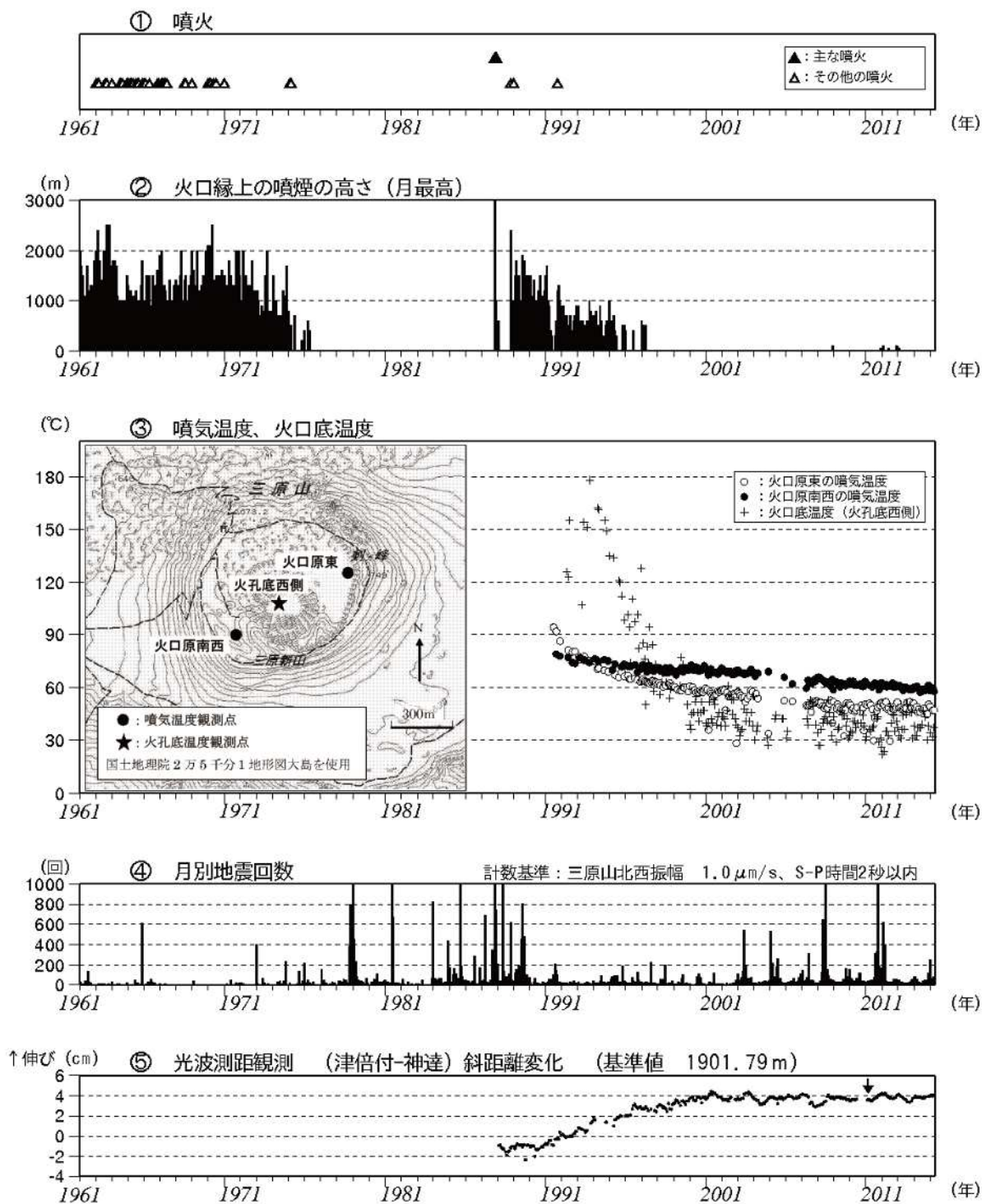
図 1 伊豆大島 長期間の火山活動経過図（1961 年 1 月～2014 年 4 月 30 日） 1991 年 12 月 18 日までは火口縁上 130m 以上、2002 年 2 月 28 日までは火口縁上 300m 以上の噴煙の高さを観測していました。 火口底温度（火口底西側）は赤外放射温度計を用いて離れた場所から測定した値。 噴気温度（火口原東、火口原南西）はサーミスタ温度計を用いて直接測定した値。 地震回数には伊豆大島周辺海域で発生した地震も一部含まれています。 光波距離計 4) による月平均値（観測開始は 1987 年 1 月）。グラフの空白部分は欠測。矢印は機器更新を示します。
