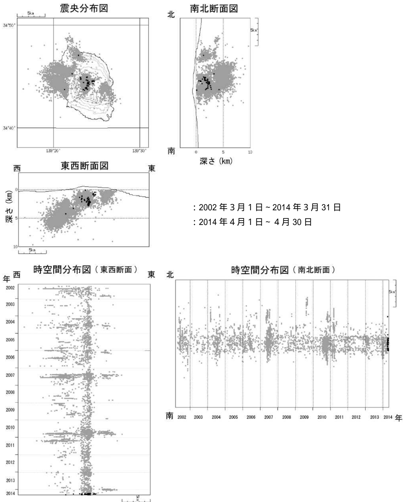
図 7 伊豆大島 震源分布図（2002 年 3 月 1 日 ~ 2014 年 4 月 30 日）
