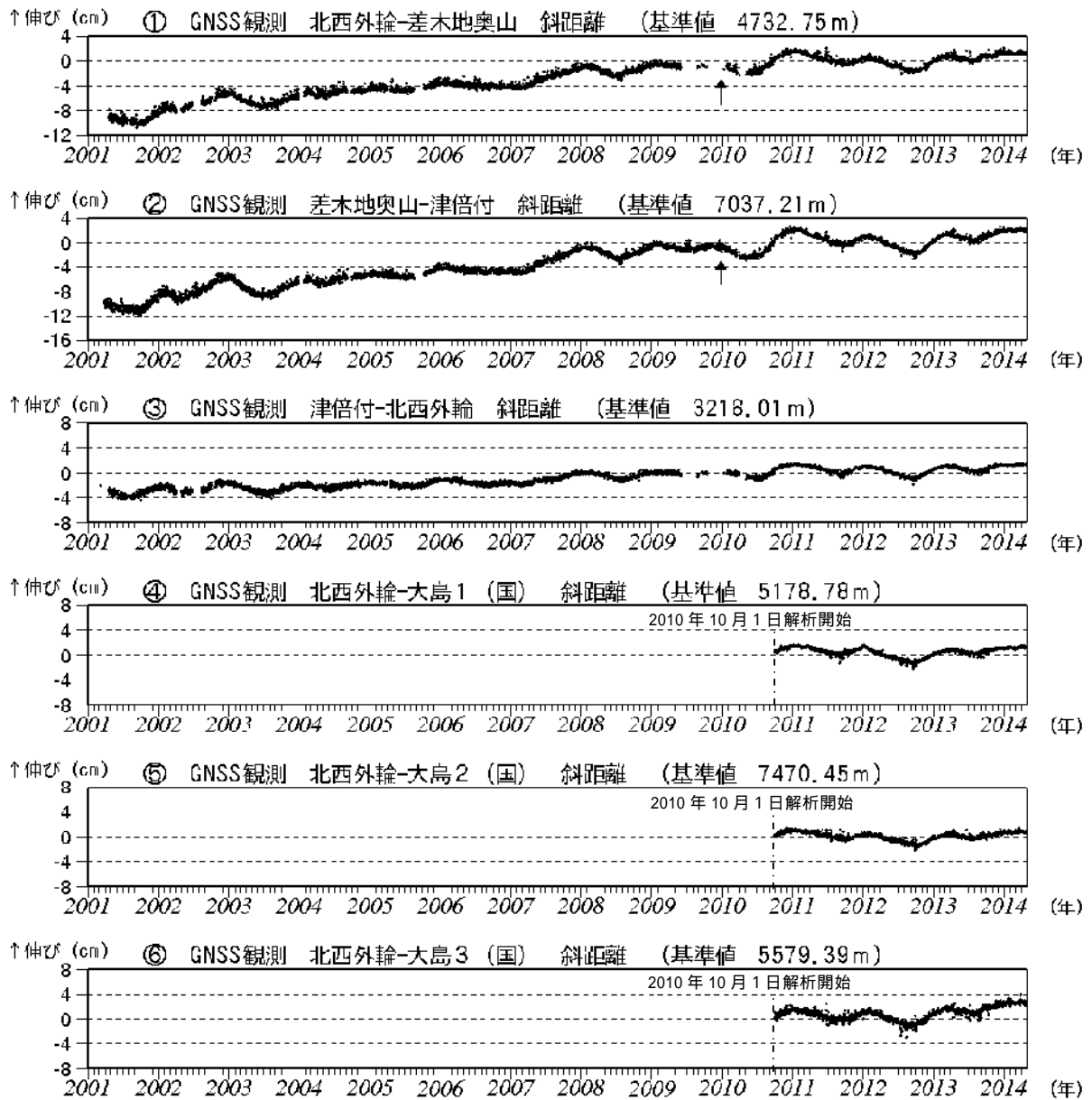
図3 伊豆大島 GNSS連続観測による基線長変化(2001年1月~2014年4月30日)(国): 国土地理院 2010年10月以降のデータについては、電離層の影響を補正する等、解析方法を改良しています。 ~ は図8のGNSS基線 ~ に対応しています。 グラフの空白部分は欠測。 の矢印は差木地奥山支柱工事を実施。
