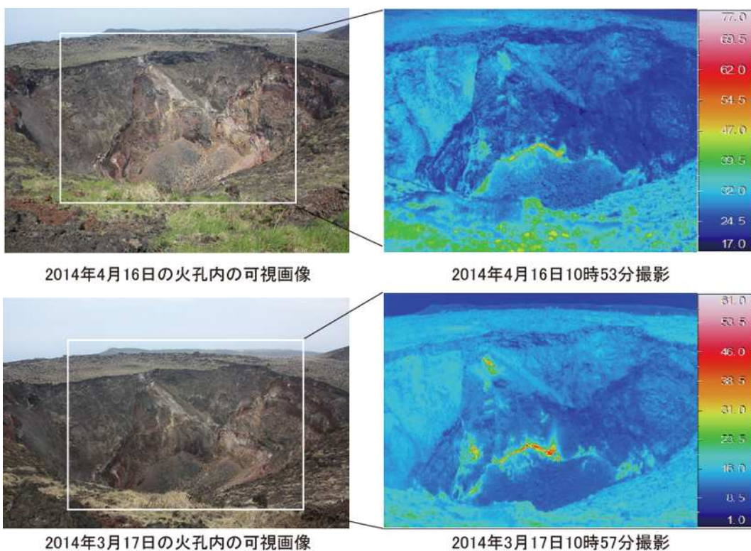
図5 伊豆大島 中央火口内の状況（左）と地表面温度分布 2) （右）
