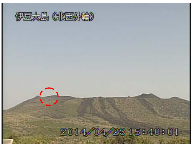
山頂部（4月23日、北西外輪遠望カメラによる） 剣ガ峰付近（4月16日、撮影方向は図6参照） 図4 伊豆大島 三原山山頂部及び山頂火口の状況 破線円内：ごく弱い噴霧
