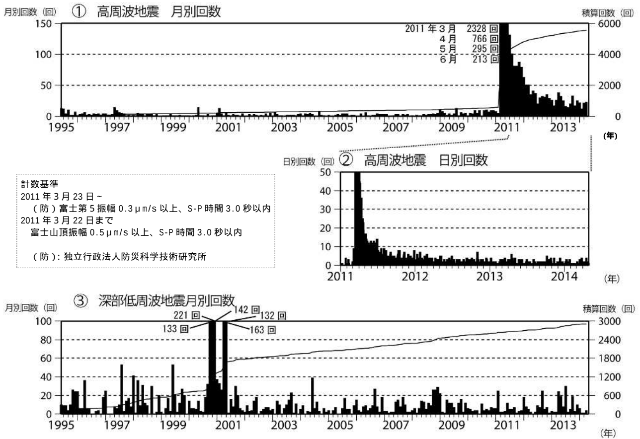
図 2 富士山 月別及び日別地震回数（1995 年 6 月 1 日～2014 年 4 月 30 日）
