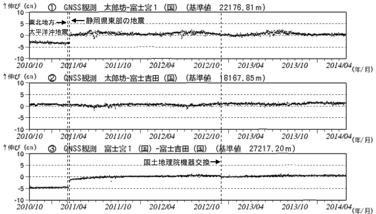
図4 富士山 GNSS 連続観測による基線長変化 (2010 年 10 月 1 日～2014 年 4 月 30 日)
