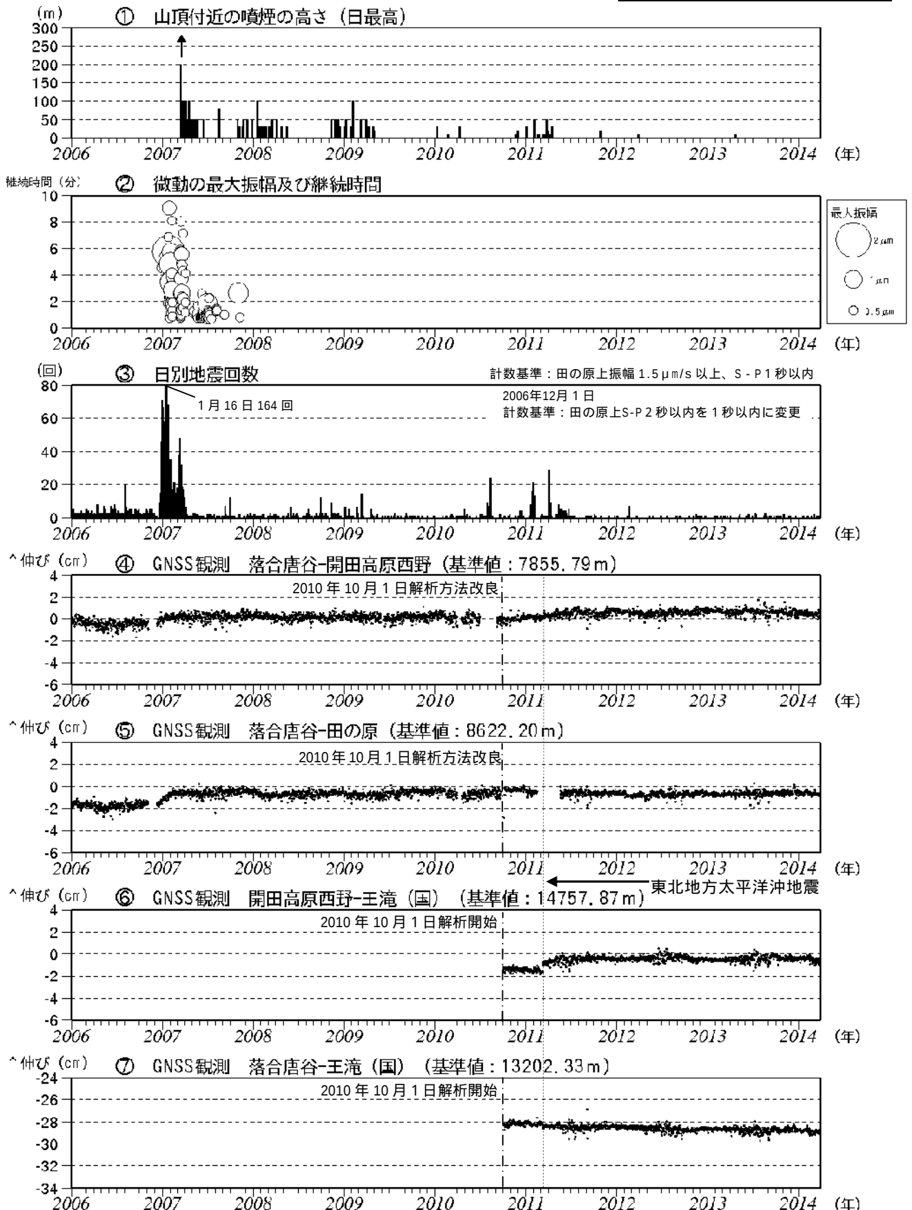
図3 御嶽山 最近の火山活動経過図（2006年1月1日～2014年3月31日）
