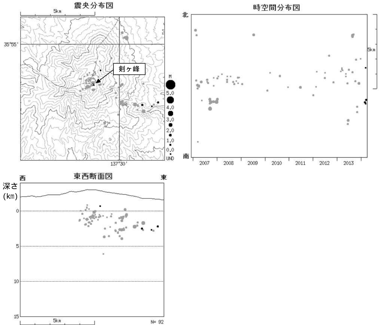
図 4 御嶽山 震源分布図（2006 年 12 月 1 日～2014 年 3 月 31 日） ●：2006 年 12 月 1 日～2014 年 2 月 28 日 ●：2014 年 3 月 1 日～3 月 31 日
