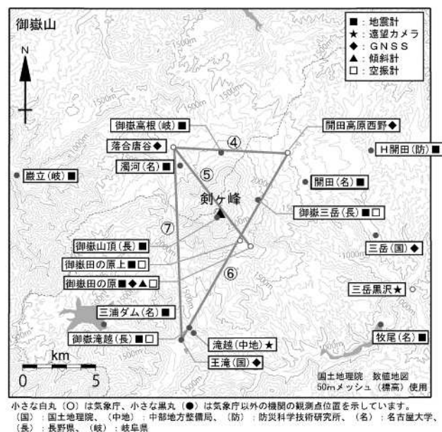
図 5 御嶽山 観測点配置図 図中の GNSS 基線 ～ は図 3 の ～ に対応しています。
